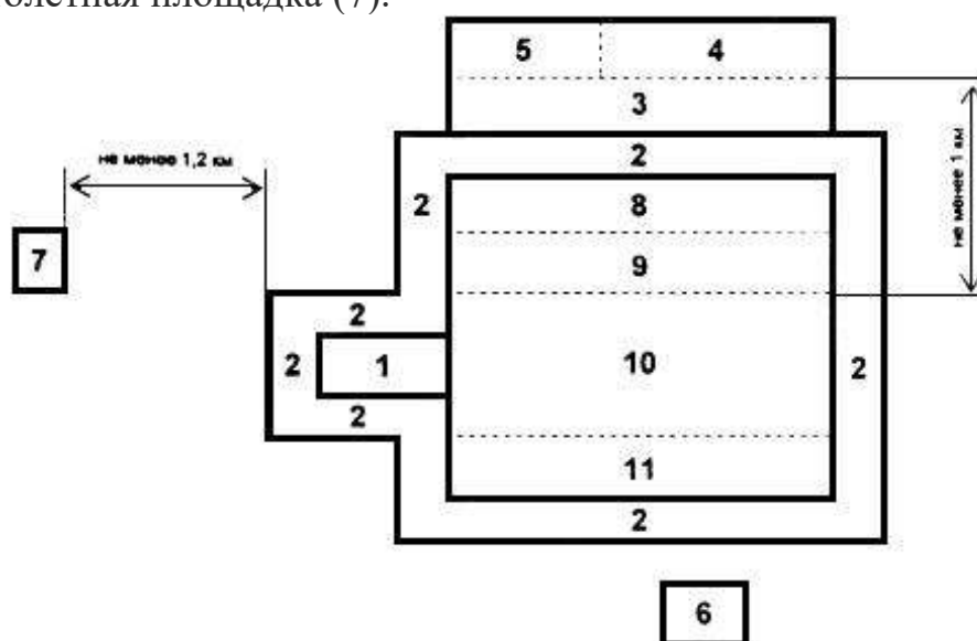
Рисунок 1 – Типовая схема территории базы
