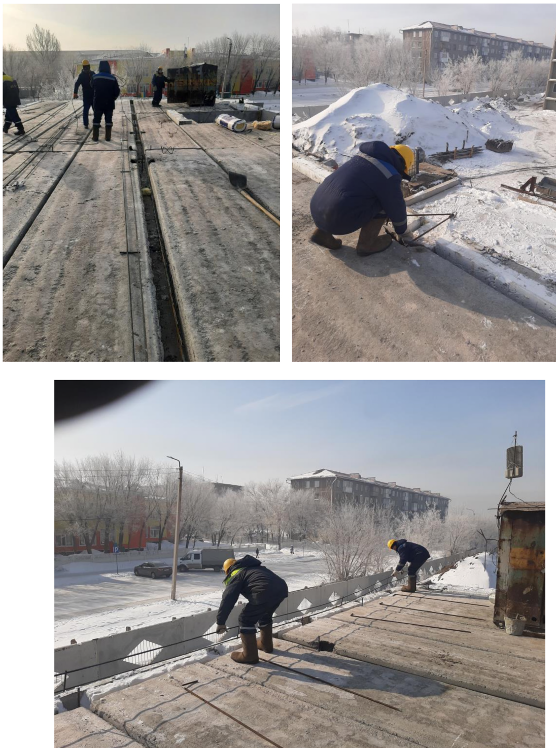
Рисунок 7 – Армирование швов плит перекрытий
