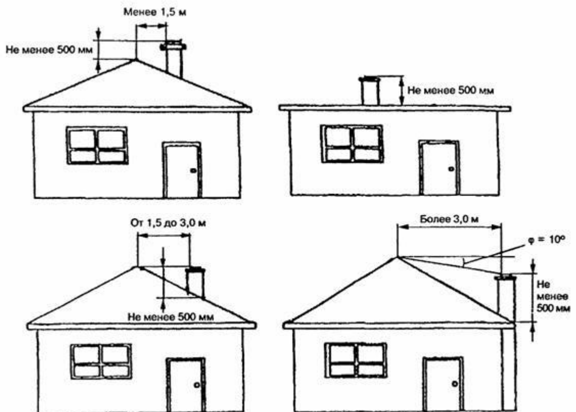
Рисунок 7.8 – Расстояние от дымовой трубы до строительных конструкций
