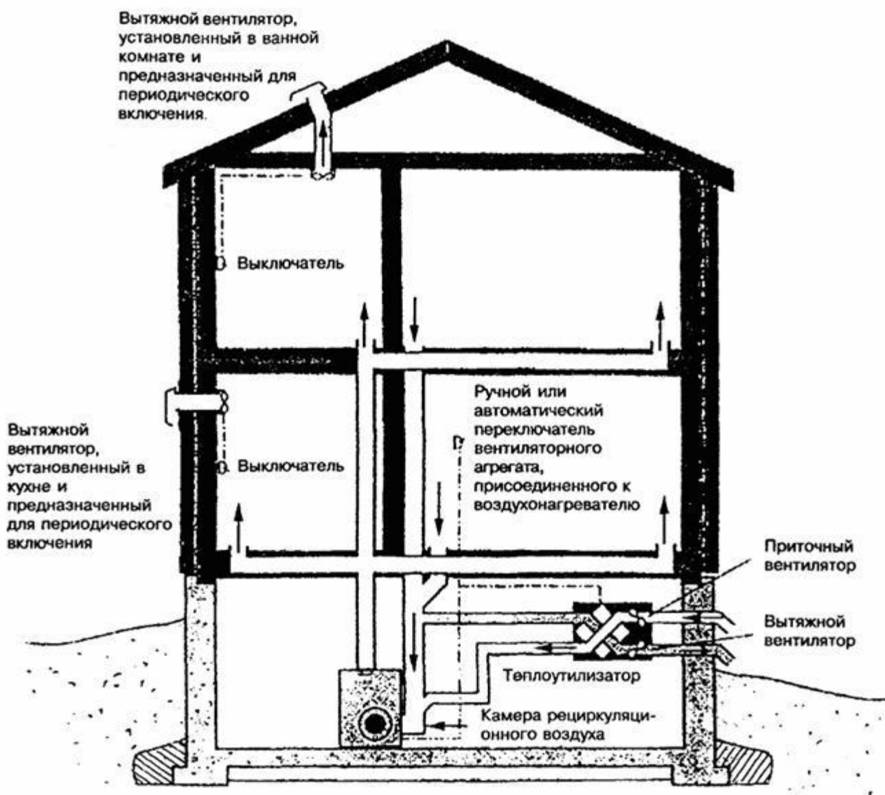
Рисунок 7.3 – Присоединение теплоутилизационного агрегата к камере подогрева воздуха
