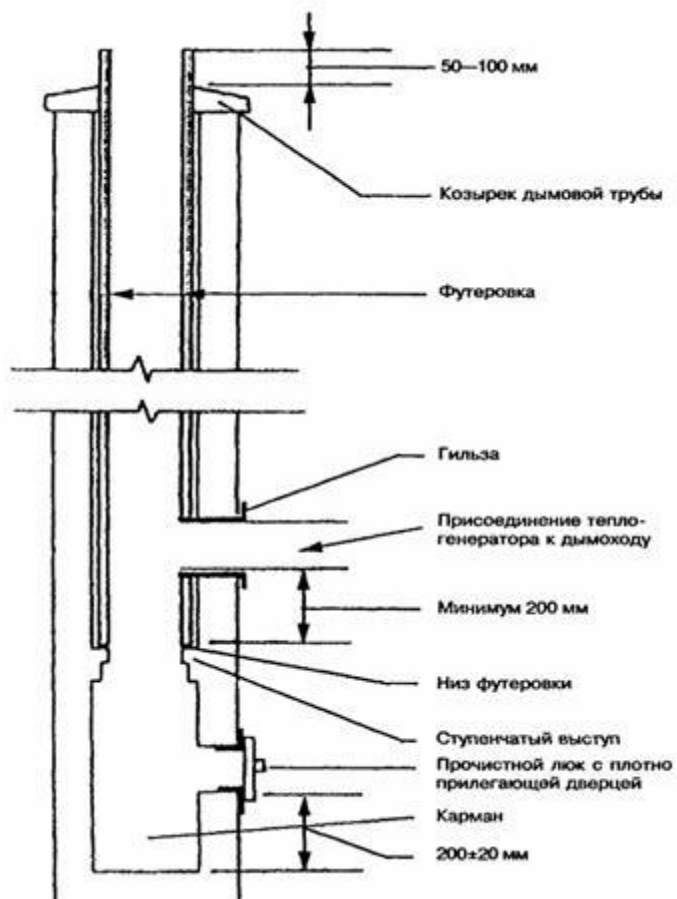
Рисунок 7.6 – Облицовка дымохода
