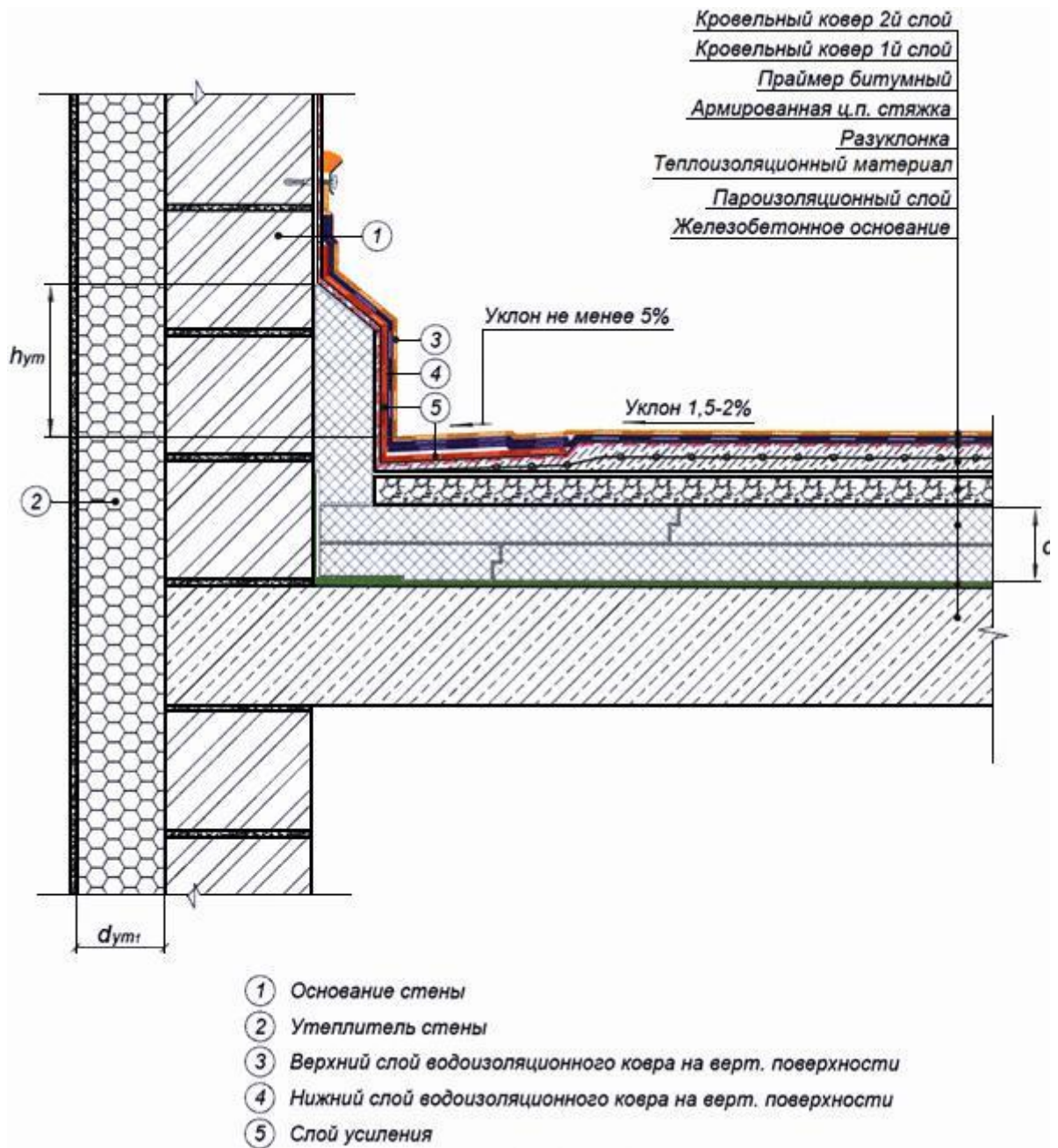
Рисунок Г.4 - Схема сопряжения СФТК с совмещенным кровельным покрытием
