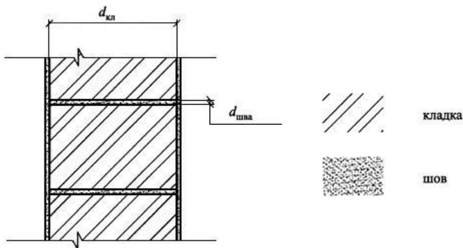
Рисунок Г.1 - Схема узла прохождения растворного шва
