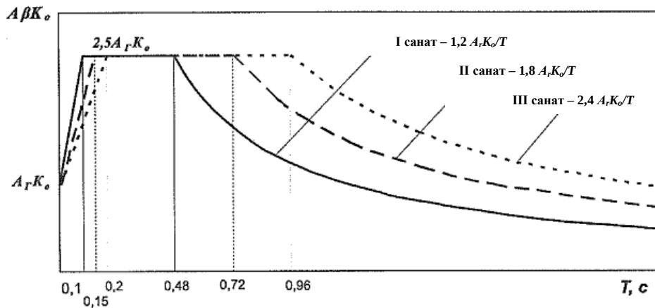
А.1-сурет – Сейсмикалық әсердің көлденең құрамдасына арналған реакция спектрі
