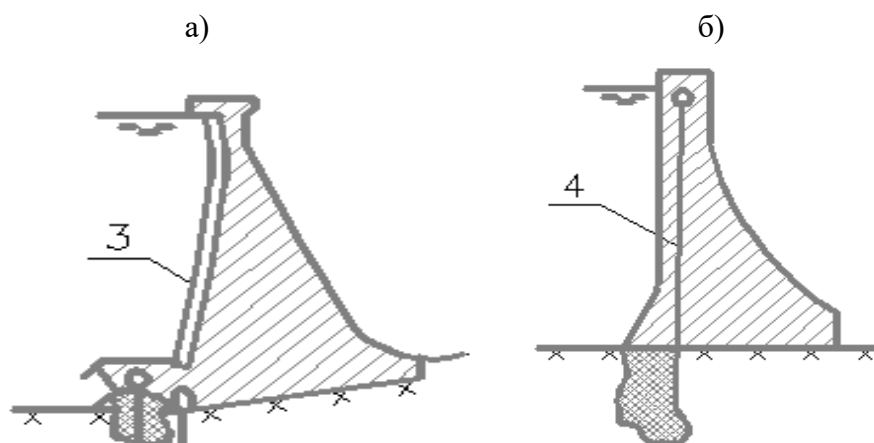
Рисунок 2 – Схемы разрезов гравитационных плотин
