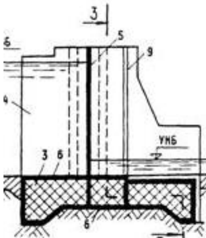
Рисунок 9 - Схемы расположения уплотнений в постоянных деформационных швах плотин на скальном (а, б) и нескальном (в, г) основаниях
