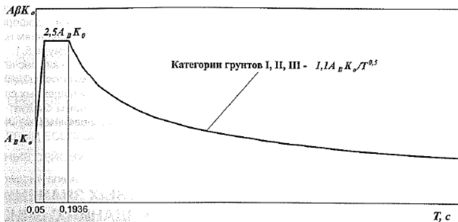
Рисунок А.2 – Спектр реакции для вертикальной составляющей сейсмического воздействия
