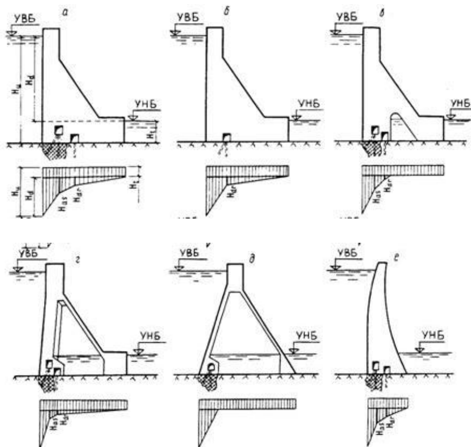
Рисунок 11 - Эпюры пьезометрического напора по подошве плотины
