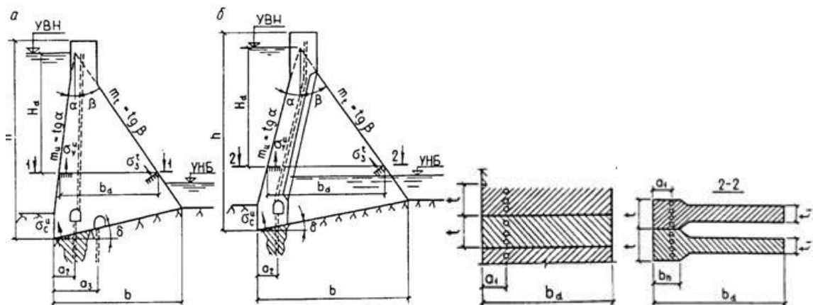
15-сурет – Бөгетті беріктілікке есептеуге берілген белгілер\
