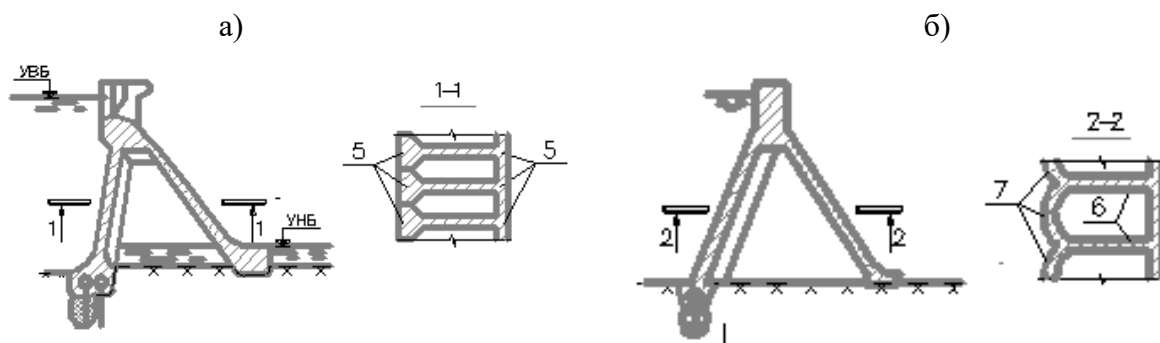
Рисунок 3 – Схемы разрезов контрфорсных плотин
