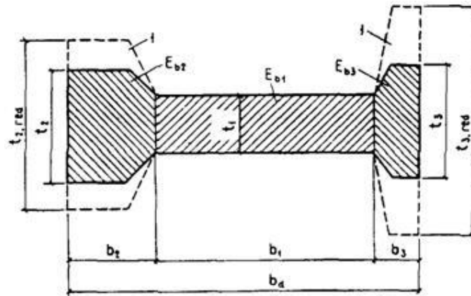
Рисунок 18. Схема к определению размеров приведенного сечения контрфорса
