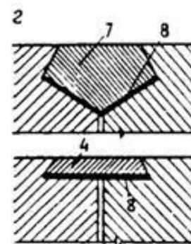
Рисунок 10 - Схемы основных уплотнений деформационных швов бетонных и железобетонных плотин
