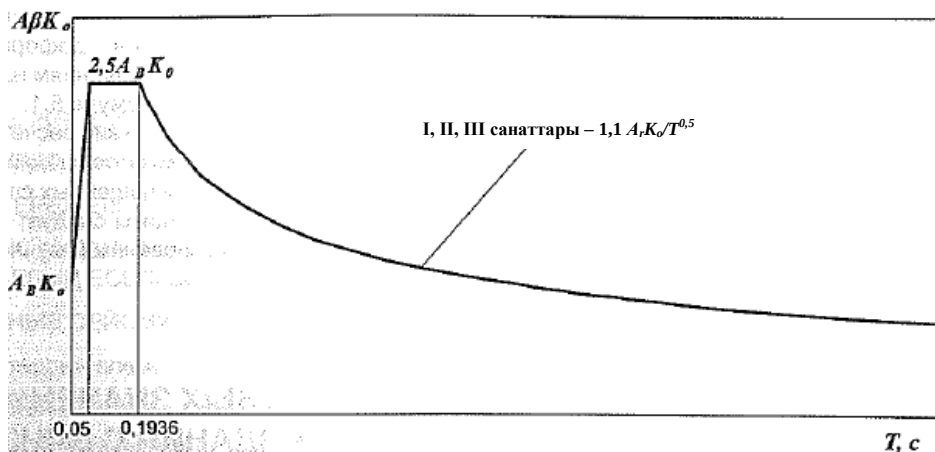
А.2-сурет – Сейсмикалық әсердің тік құрамдасына арналған реакция спектрі
