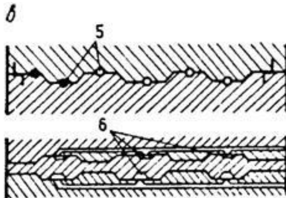
Рисунок 10 - Схемы основных уплотнений деформационных швов бетонных и железобетонных плотин
