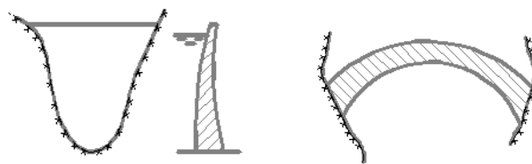
Рисунок 5 Схема разреза арочной плотины
