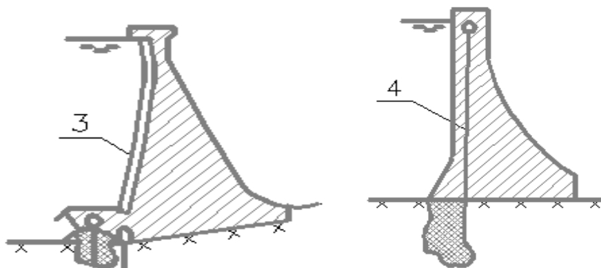
2-сурет – Гравитациялық бөгеттердің кесіктерінің схемалары (а – ағындық шегінде экраны бар бөгет; б – іргесінде анкерлеуі бар бөгет; 3 – экран; 4 – алдын-ала кернелген анкер)
