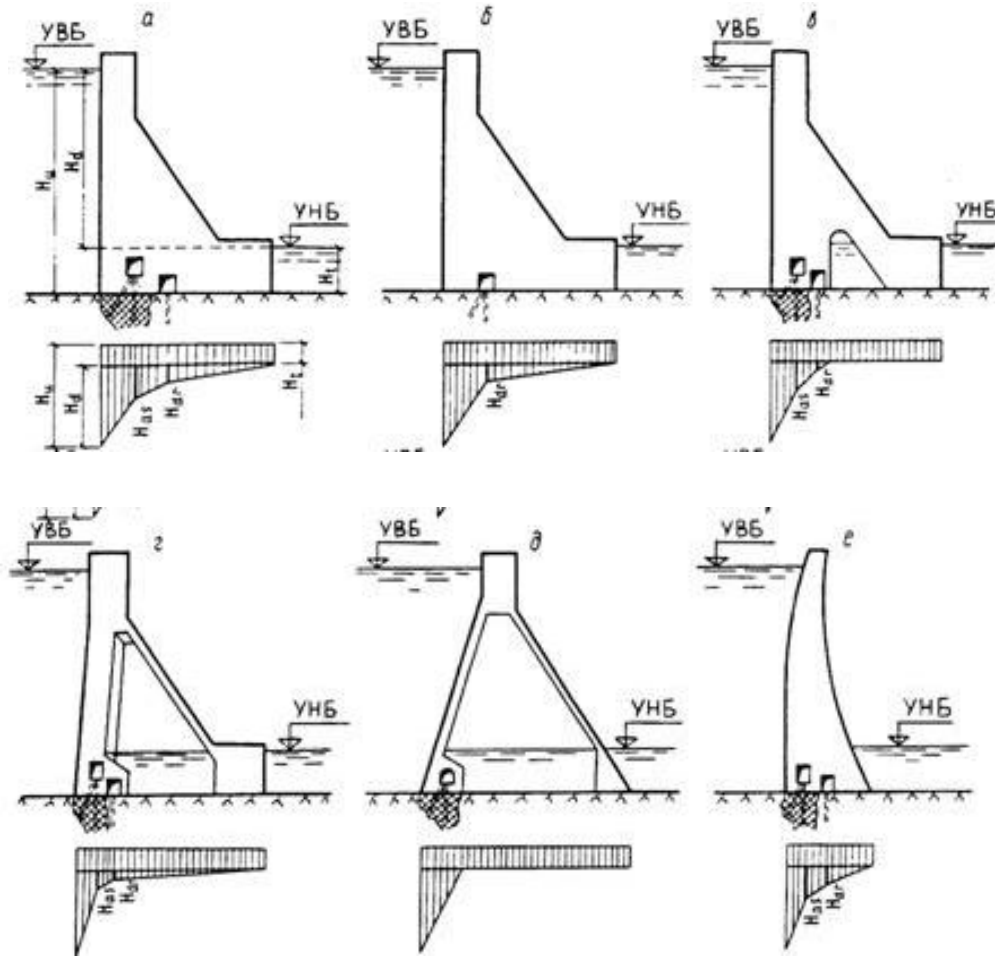
11-сурет – Бөгеттің табаны бойынша пьезометрикалық ағынның эпюралары
