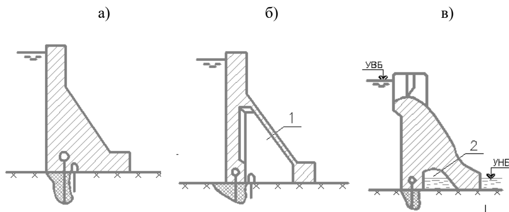
Рисунок 1 – Схемы разрезов гравитационных плотин
