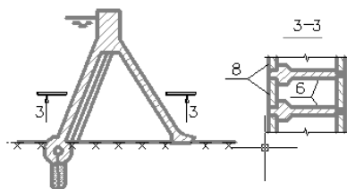
Рисунок 4 - Схема разреза контрфорсной плотины с плоским перекрытием (8 - плоское перекрытие)
