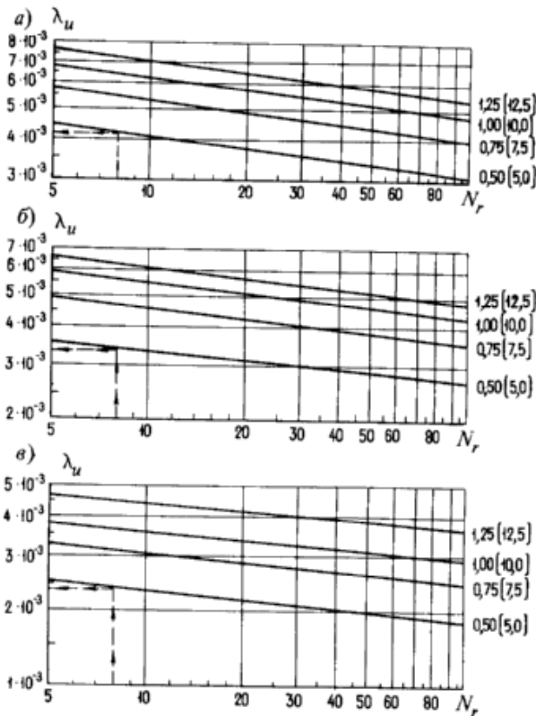
8- сызба. Топырақтарда салынатын қатты емес аэродромдық жабындылардың \lambda_u шектік салыстырмалы иілімдерді анықтау кестесі. а – құмайт, балшық, саз (қиыршық тас қоспасымен топырақты қоса алғанда), б – шаңды құм, в – құмды ірі, орта іріліктегі және ұсақ тасты; кесте желілеріндегі сызықтар әуе кемесінің пневматикалық доңғалағында ауаның ішкі қысымын білдіреді, P_a , МПа (кг/см 2 ).
