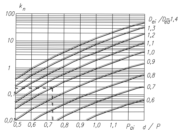
Черт.11. Номограмма для определения коэффициентов приведения нагрузки к расчетной k_n для нежестких покрытий
