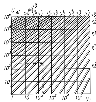
Черт. 4. Номограмма для определения эквивалентного числа приложения нагрузки U_{ei}
