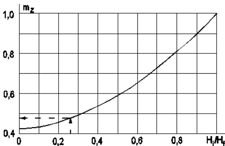
Черт. Г.2 График для определения коэффициента m_z
