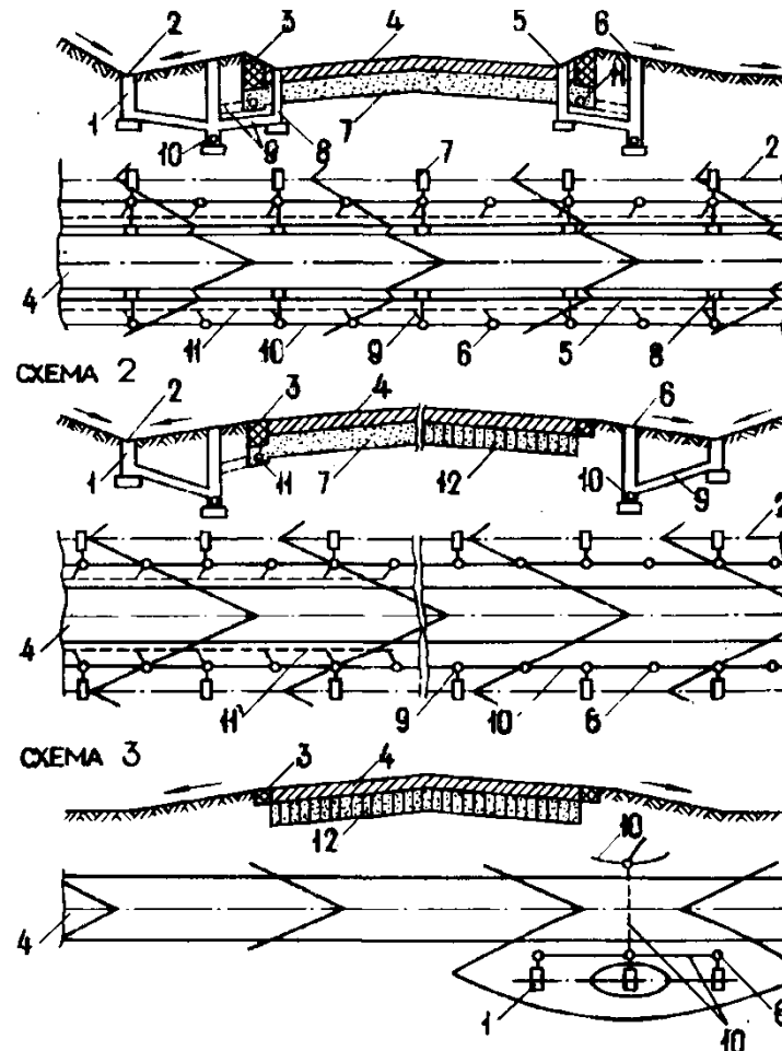
Рисунок 5 - Схемы водоотводных и дренажных систем аэродромов (поперечный профиль и план)
