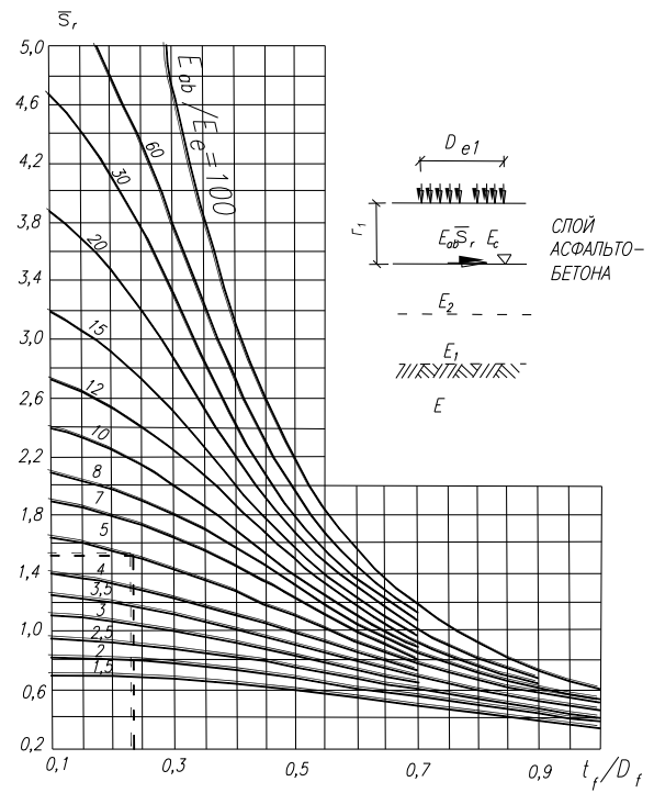
Черт. 9. Номограмма для определения удельных растягивающих напряжений при изгибе S_r в асфальтобетоне
