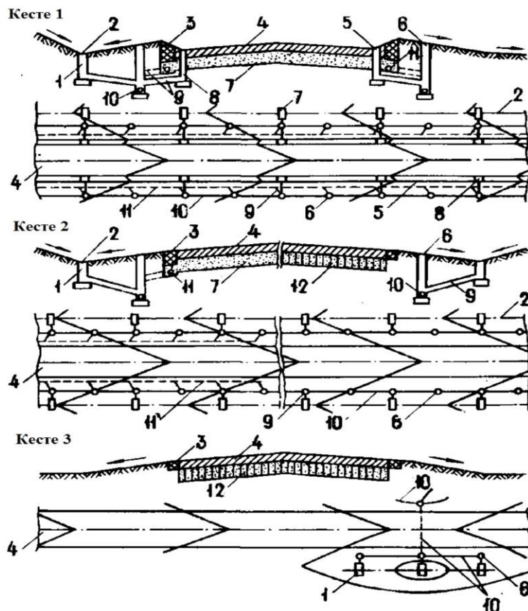
5-сурет - Аэродромның суды қашыртқы және дренаждық кестелері (көлденең профилі және жоспар)
