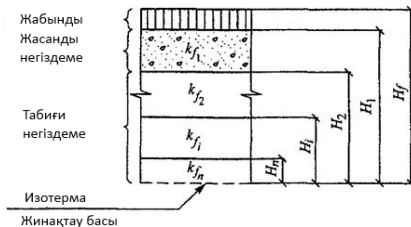
Г.1-сызба. Қабатты негіздеменің есептік кестесі
