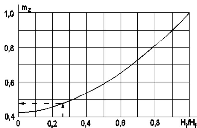
Г.2-сызба. m_z коэффициентін анықтауға арналған кесте
