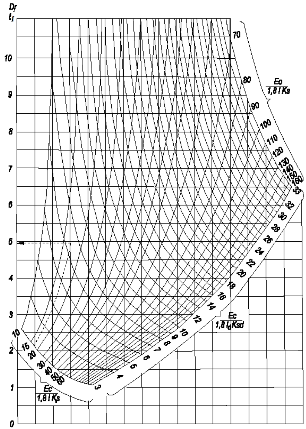
Черт. Ж.2. Номограмма для определения соотношения \frac{D_r}{t_f}
