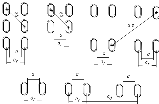
Черт. 11. Расчетные расстояния a , a_r и a_d между колесами опор воздушных судов
