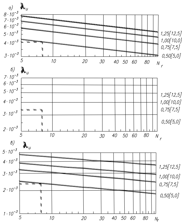
Черт. 8. График для определения предельных относительных прогибов \lambda_u м, нежестких аэродромных покрытий, устраиваемых на грунтах
