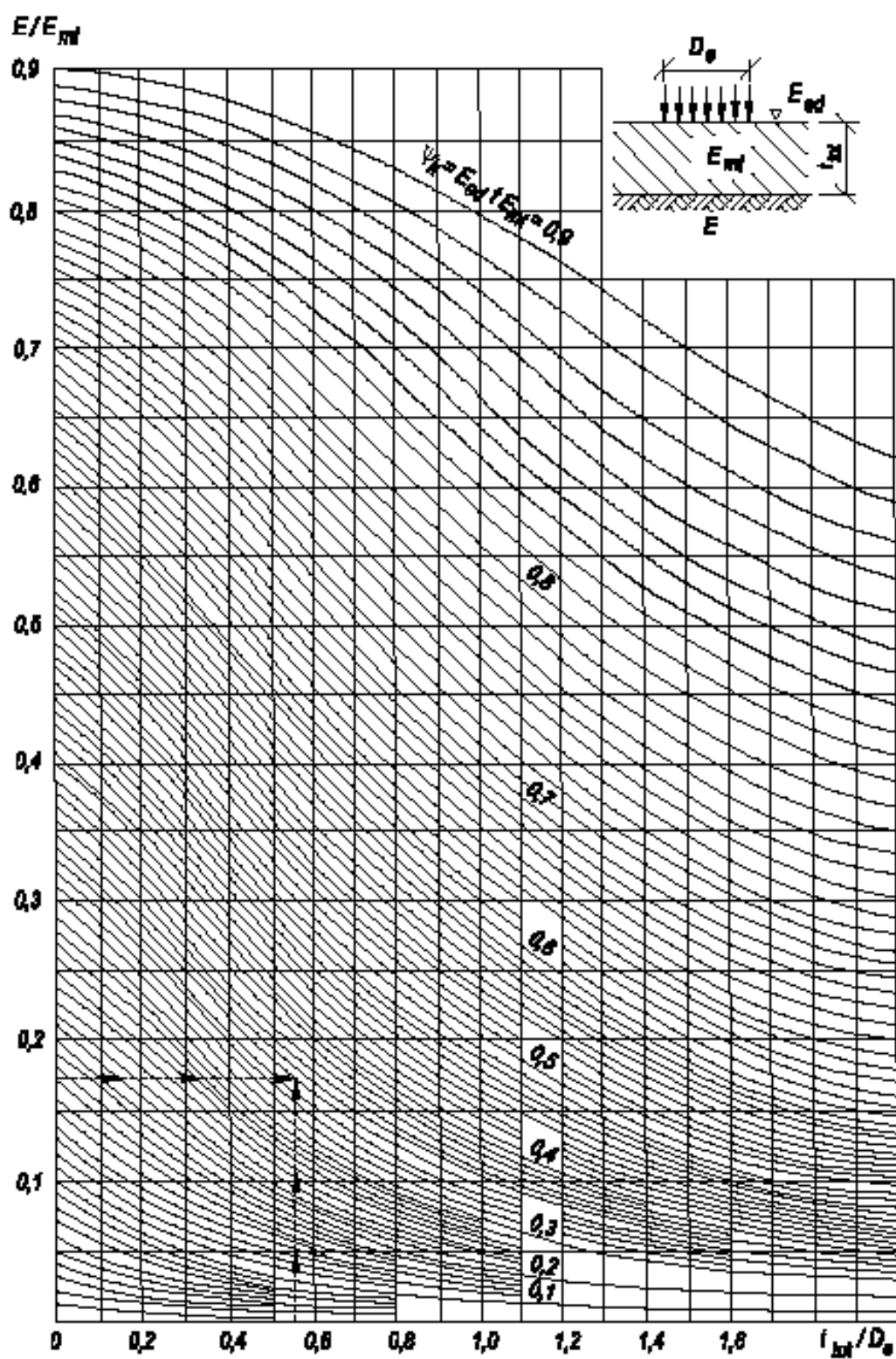
Е.7-сызба. Қатаң емес төсем үшін \Psi_k коэффициентін анықтау үшін номограмма
