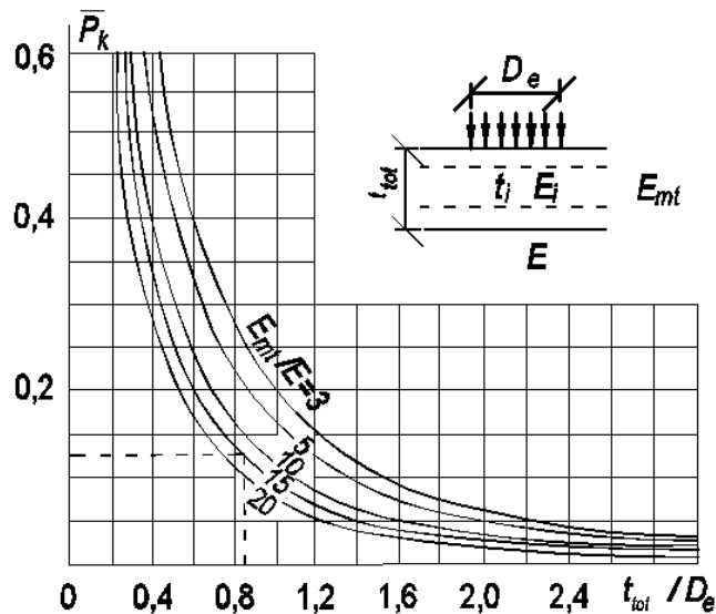
Қатаң емес төсемінің топырақтық негіздеме беттерінде \bar{p}_k алшақ байланыс қысымын анықтау үшін номограмма
