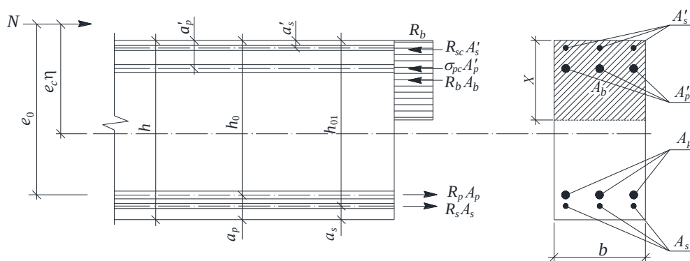
5-сурет - Беріктілігін есептеген кезде, орталықтандырылмай қысылған темірбетон элементтің, ұзыннан өсіне қалыпты, қимадағы кернеу эпюрасы мен күшеюдің сызбасы
