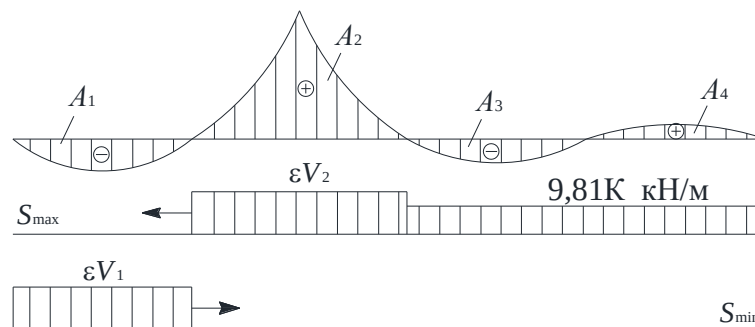
Е.5-суреті- Төзімділікке қатысты есептеу кезінде ең жоғарғы және ең төменгі күштерді (кернеулерді) анықтауға арналған әсер ету сызығының учаскелерін жүктеу схемасы
