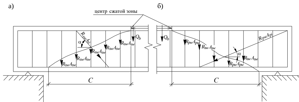
Рисунок 7 - Схема усилий в сечении, наклонном к продольной оси железобетонного элемента, при расчете его по прочности на действие поперечной силы
