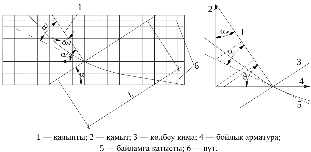
10-сурет - Қалыпты көлденең арматурадағы көлбеу қимаға түсетін күш проекциясы
