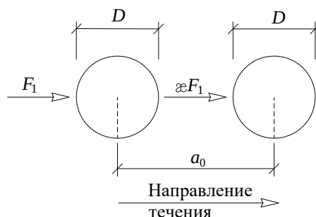
Рисунок Л.1 – Схема расположения в одном створе вдоль течения реки двух опор
