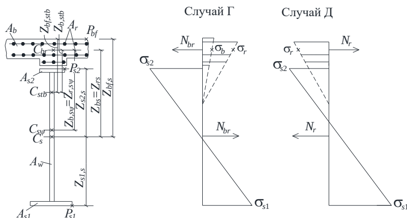
Рисунок 17 — Усилия и напряжения в сталежелезобетонном поперечном сечении, воспринимающем отрицательный изгибающий момент
