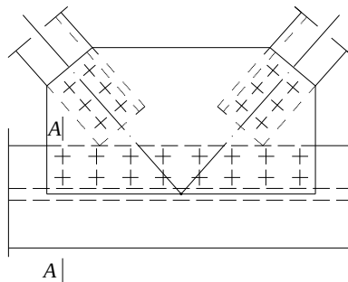
Рисунок У.3 - Расположение проверяемого на выносливость расчетного сечения А – А по основному металлу в сечении брутто по первому ряду высокопрочных болтов в прикреплении фасонки к нестыкуемым в данном узле поясам сплошных балок и элементам решетчатых форм
