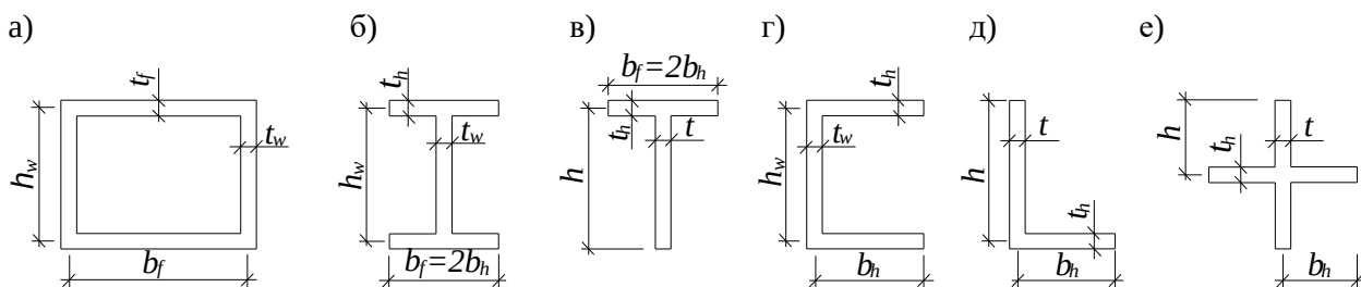
Рисунок 11 — Схемы расчетных сечений элементов, не подкрепленных
