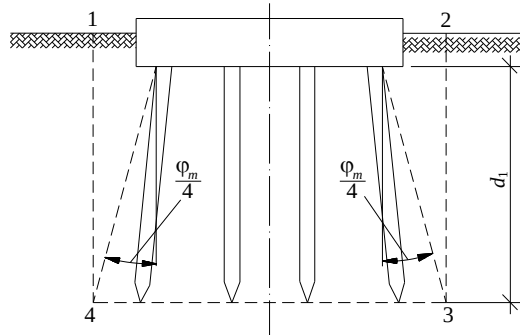
Я.1-суреті- Қадалардың \phi_m/4 кем көлбеу бұрышы кезіндегі, топыраққа тереңдетілген ростверкті, шартты қада іргетасы
