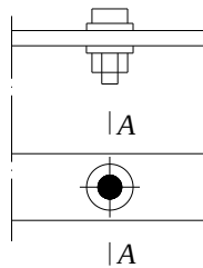
Рисунок У.2 - Расположение проверяемого на выносливость расчетного сечения А – А по основному металлу в сечениях нетто у отверстия с поставленным в него высокопрочным болтом, затянутым на нормативное усилие
