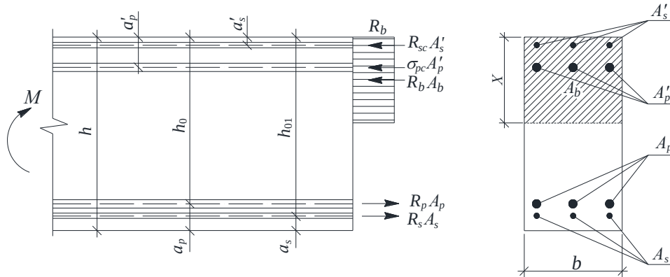
2-сурет — Беріктілігін есептеген уақытта иілетін темірбетон элементтің ұзыннан өсіне қалыпты қимадағы кернеу эпюрасының және күшеюінің сызбасы
