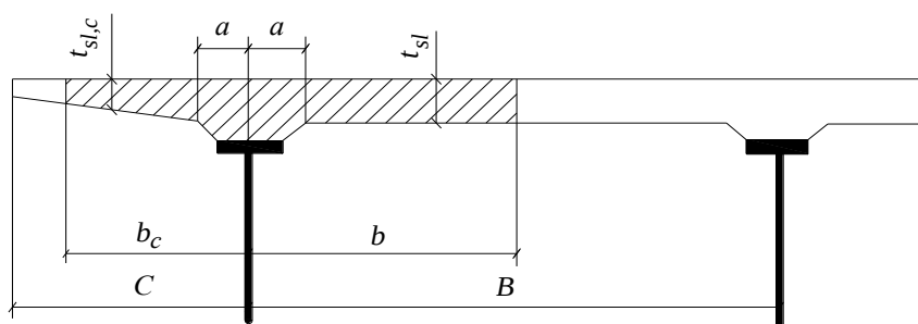
15-сурет - Қима құрамында ескерілген темірбетон плитаның есептік енін анықтауға арналған схема
