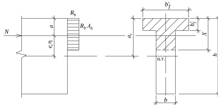
Рисунок 4 - Схема усилий и эпюра напряжений в сечении, нормальном к продольной оси внецентренно сжатого бетонного элемента
