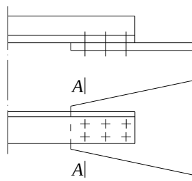
У.6-суреті- Төзімділігі тексерілетін есептік қиманың орналасуы, Торапқа бекітуде немесе біржақты жаймалары бар бір қабырғалы элементтердің түйіспесіндегі бірінші төзімділігі жоғары бұрандамалардың бірінші қатары бойынша брутто қимасындағы негізгі металл бойынша А – А
