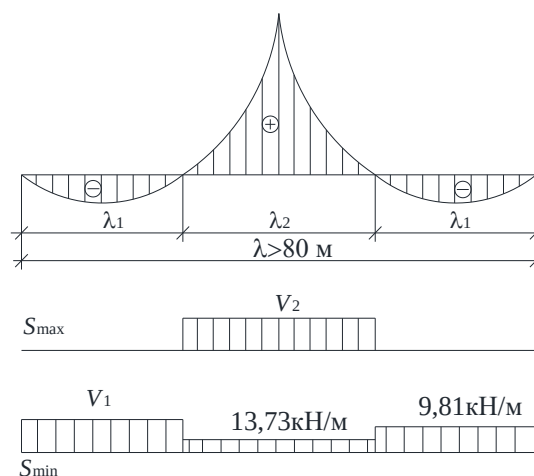
Е.3-суреті- \lambda > 80 м болған кезде әсер ету желісінің учаскелерін жүктеу схемасы
