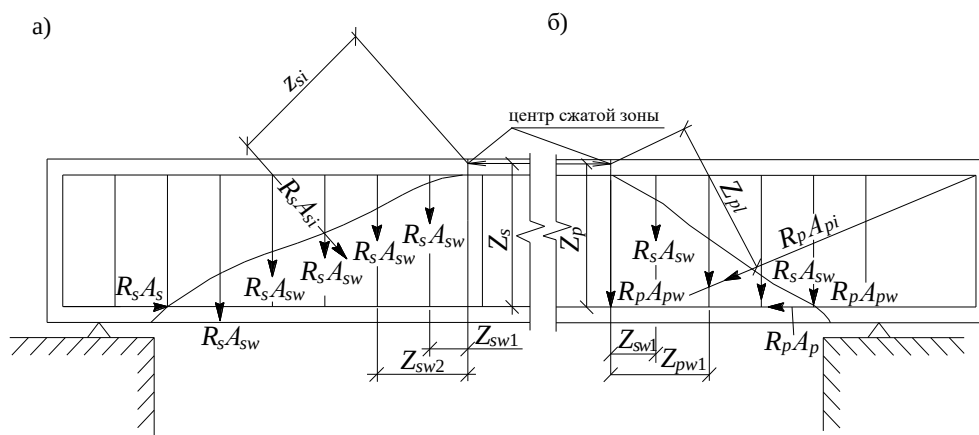
Рисунок 8 - Схема усилий в сечении, наклонном к продольной оси
