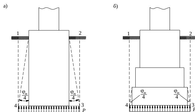
Рисунок Я.4 — Условный свайный фундамент с ростверком, расположенным над грунтом, при угле наклона свай более \varphi_m/4
