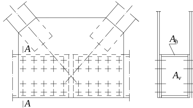
У.5-суреті- Төзімділігі тексерілетін есептік қиманың орналасуы, орапқа бекітуде немесе біржақты жаймалары бар екі қабырғалы элементтердің түйіспесіндегі бірінші төзімділігі жоғары бұрандамалардың бірінші қатары бойынша брутто қимасындағы негізгі металл бойынша А – А
