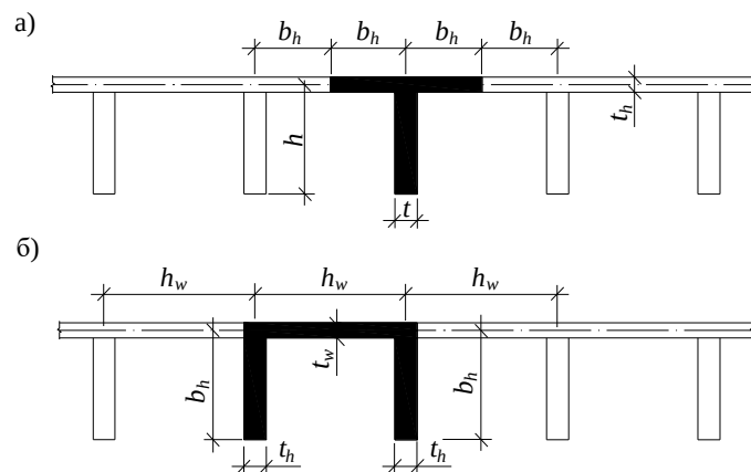
Рисунок 12 — Схемы расчетных сечений пластинок ортотропных плит
