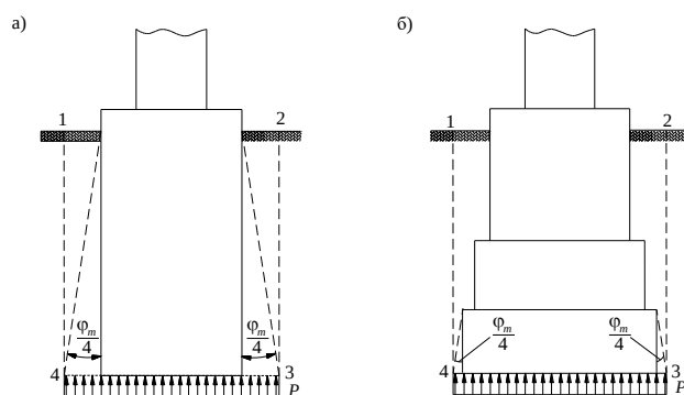
Я.4-суреті- Қадалардың, \varphi_m/4 артқы, көлбеу бұрышы кезіндегі, топырақ үстіне орналасқан ростверкті, шартты қада іргетасы
