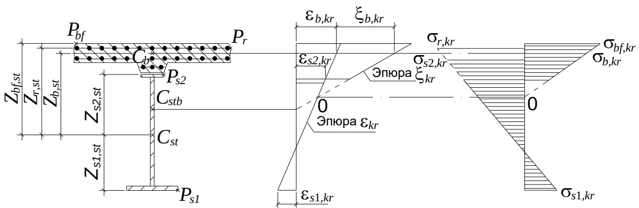
Х.1-суреті— Салыстырмалы деформациялардың және бетонның жылжығыштығынан түсетін ішкі кедергілердің эпюралары
