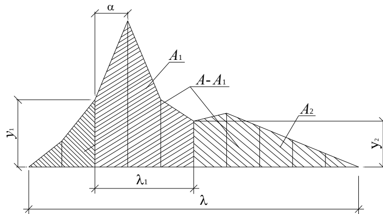
Е.2-суреті- Оның жоғарғы бөлігін қоса алғанда ұзындығы \lambda әсер ету сызығының бөлігі
