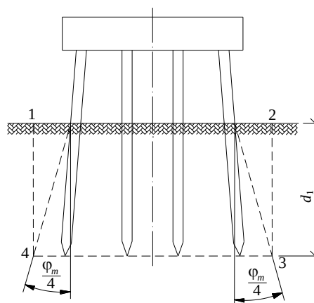
Я.3 –суреті - Қадалардың, \phi_m/4 кем, көлбеу бұрышы кезіндегі, топырақ үстіне орналасқан ростверкті, шартты қада іргетасы
