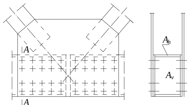
Рисунок У.5 — Расположение проверяемого на выносливость расчетного сечения А – А по основному металлу в сечении брутто по первому ряду высокопрочных болтов в креплении к узлу или в стыке двухстенчатых элементов с односторонними накладками
