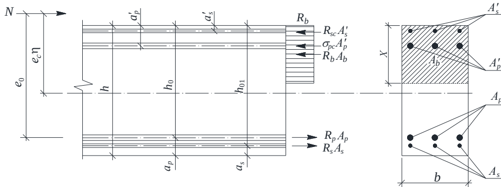
Рисунок 5 - Схема усилий и эпюра напряжений в сечении, нормальном к продольной оси внецентренно сжатого железобетонного элемента, при расчете его по прочности
