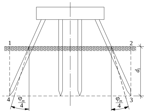
Рисунок Я.4 — Условный свайный фундамент с ростверком, расположенным над грунтом, при угле наклона свай более \varphi_m/4
