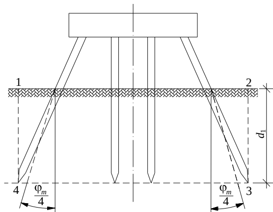
Я.4-суреті- Қадалардың, \varphi_m/4 артқы, көлбеу бұрышы кезіндегі, топырақ үстіне орналасқан ростверкті, шартты қада іргетасы
