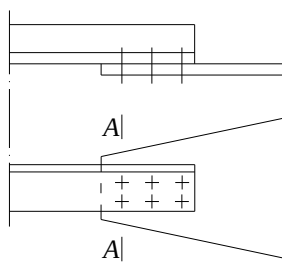
Рисунок У.6 — Расположение проверяемого на выносливость расчетного сечения А – А по основному металлу в сечении брутто по первому ряду высокопрочных болтов в креплении к узлу или в стыке одностенчатых элементов с односторонними накладками
