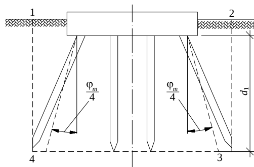
Я.2-суреті- Қадалардың, \phi_m/4 артық, көлбеу бұрышы кезіндегі, топыраққа тереңдетілген ростверкті, шартты қада іргетасы
