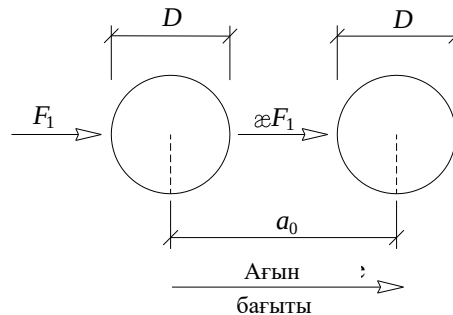
Л.1-суреті– Өзен ағысының бойымен екі тіреудің бір жақтауда орналасу сызбасы
