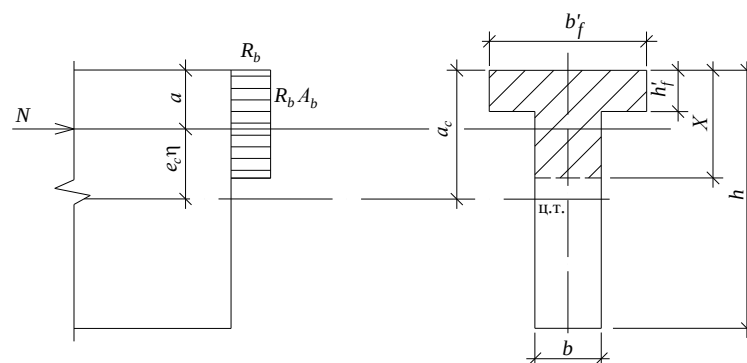
4-сурет - Орталықтандырылмай қысылған бетон элементтің ұзыннан өсіне қалыпты, қимадағы кернеу эпюрасы мен күшеюдің сызбасы
