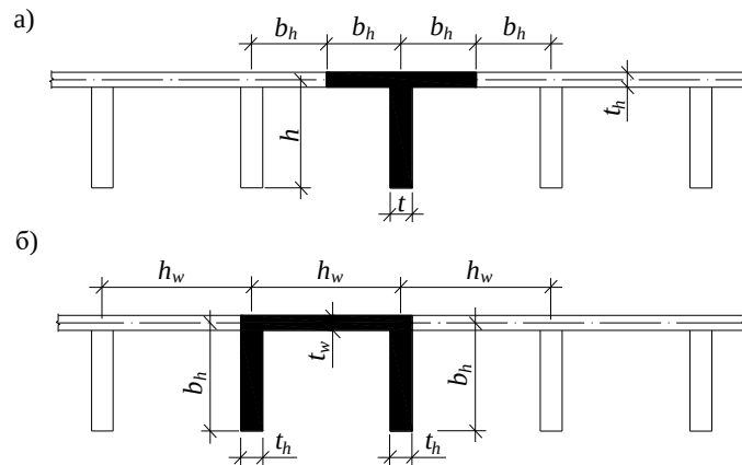
12-сурет - Ортотропты плиталар пластиналарының есептелген қималарының сызбалары
