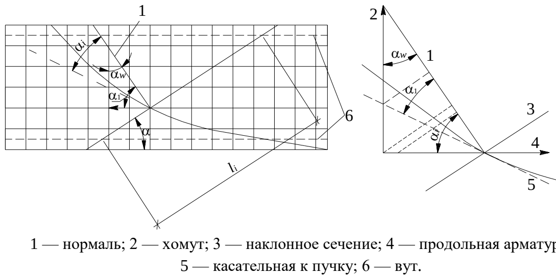
Рисунок 10 - Проекция усилий в поперечной арматуре на нормаль к наклонному сечению
