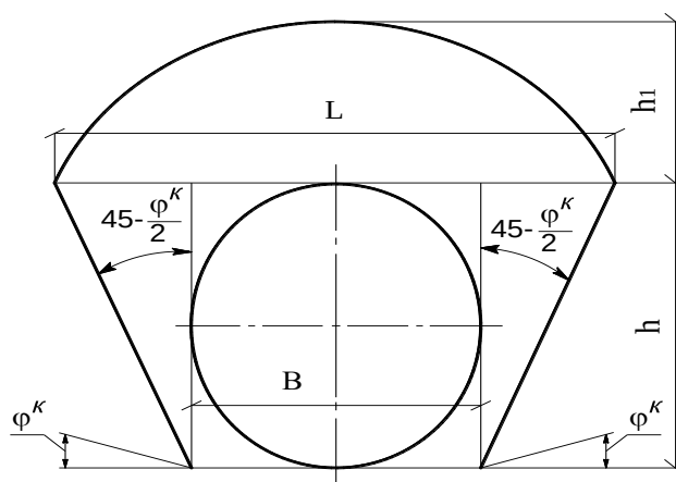
1-сурет – Опырылу күмбезі биіктігін есептеуге арналған сызбанұсқа
