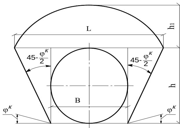
Рисунок 1 - Схема для расчета высоты свода обрушения
