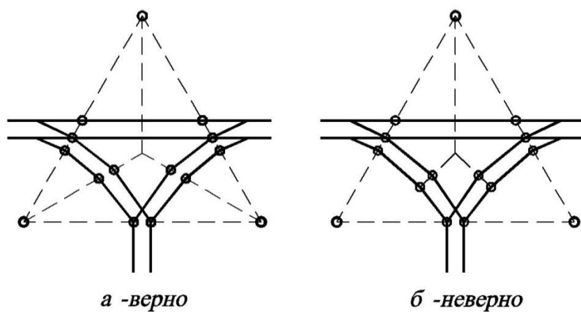
Рисунок В.3 - Схема фиксации контактных проводов трамвая на кривых участках пути
