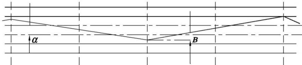
В.1-сурет - Трамвай жолдарының қосылу бөлімдеріндегі иректелу сұлбасы Қабылданатын шығынқы мм – 250-а, мұнда "а" – жол осьтерінің аралық қашықтығы
