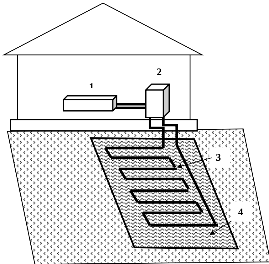
1 - жылыту аппараты; 2 – жылулық сорғыш; 3 – пластик құбыр, 4 – су қоймасы
