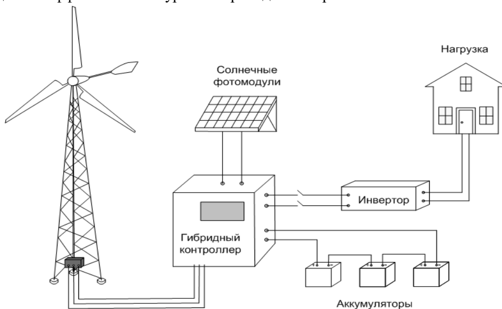
Рисунок 10 - Ветро-Солнечная (гибридная) установка и ее элементы
