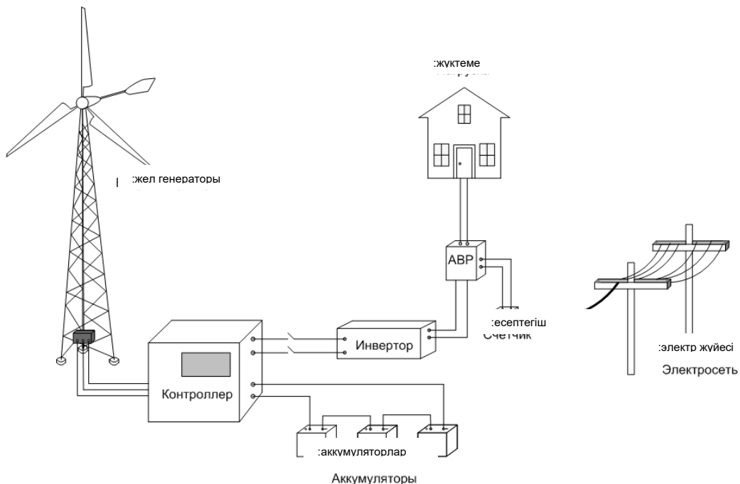
11-сурет – Желілік жел қондырғысы және оның элементтері
