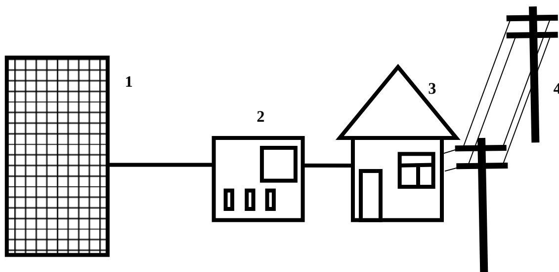
1 – солнечные панели, 2 - инвертор
