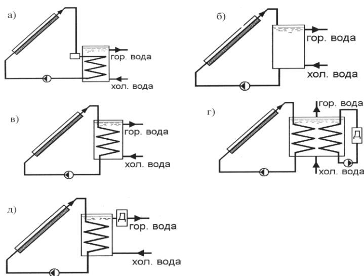
а) осушаемого типа, б) без промежуточного теплоносителя, в) с промежуточным теплоносителем, г) СК и дублирующий источник работают на один бак-аккумулятор, д) СК для предварительного подогрева
