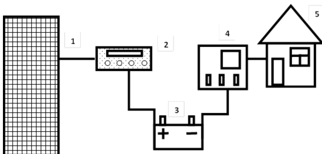
Рисунок 6 – Основные элементы с полной мощностью электроснабжения от солнечной системы
