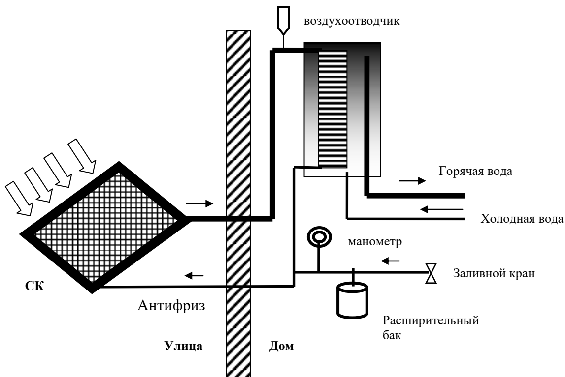
Рисунок 4 – Схема подключения солнечного коллектора для горячего водоснабжения в зимнее время
