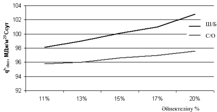
30-сурет – Коттедж ғимараты қасбетінің әйнектелуі және бағдарына орай меншікті энергияны қолдану тәуелділігінің мысалы
