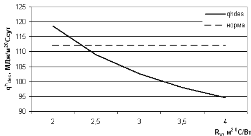
31-сурет – Коттедж ғимараты сыртқы қабырғаларының көрсетілген қарама-қайшылығына орай меншікті энергияны қолдану тәуелділігінің мысалы
