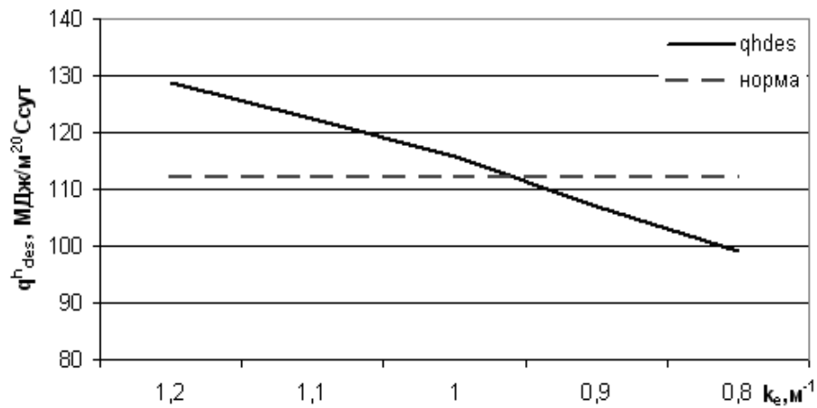
29-сурет – Коттедж ғимаратының ықшамдылығына орай меншікті энергияны қолдану тәуелділігінің мысалы
