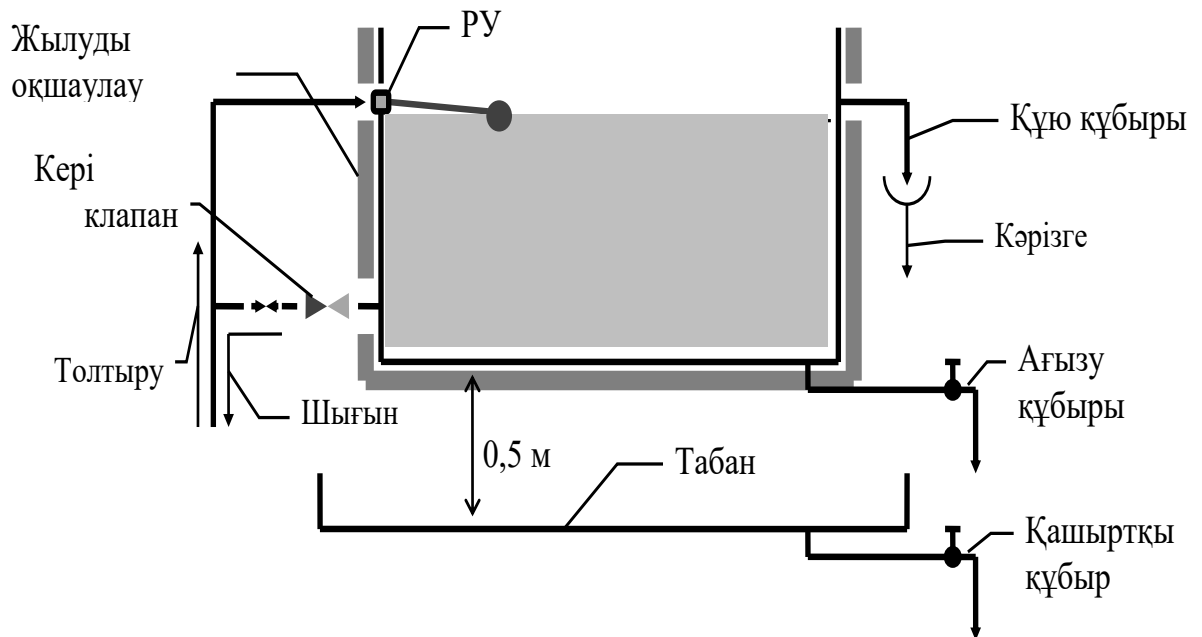
25-сурет - Күбі-аккумуляторды бекіту
