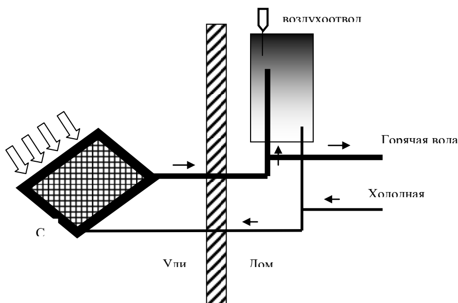
Рисунок 3 – Схема подключения солнечного коллектора для горячего водоснабжения в летнее время
