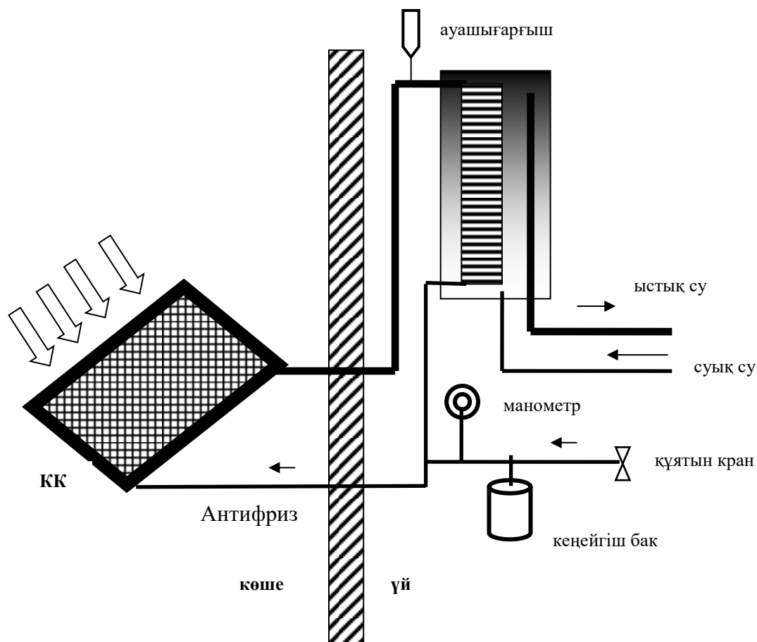
4-сурет – Қыс мезгілінде ыстық сумен қамтуға арналған күн коллекторын жалғау сызбасы
