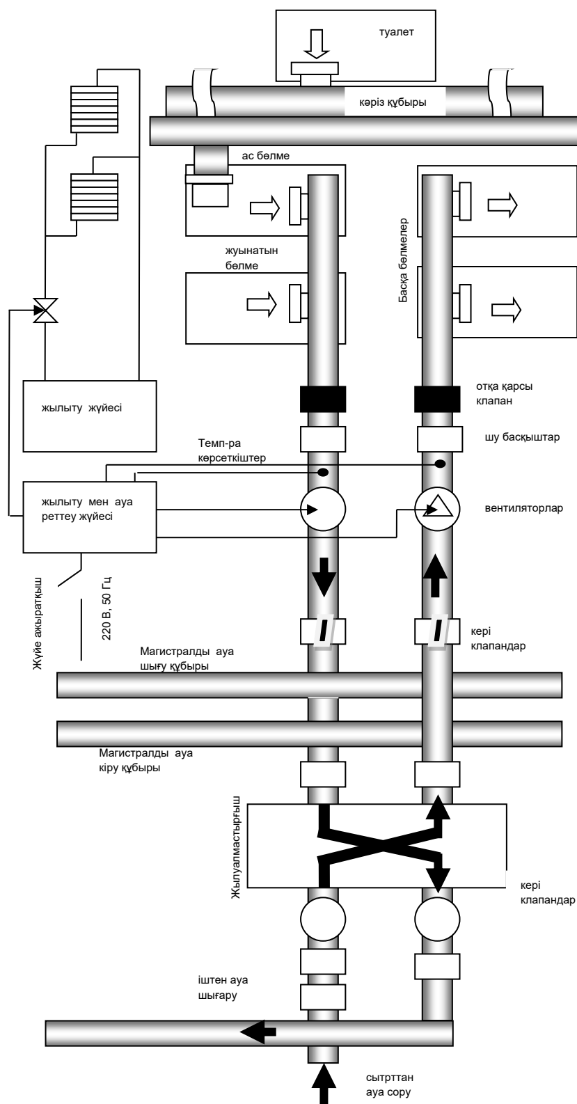
35-сурет – Газдық ас үй пеші бар коттедж ғимаратын инженерлік жабдықтаудың функционалдық сызбасы
