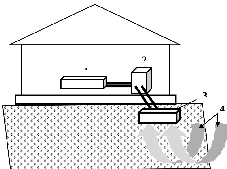
1 - отопительный аппарат; 2 - тепловой насос; 3 –система сбора тепла воздуха (4)
