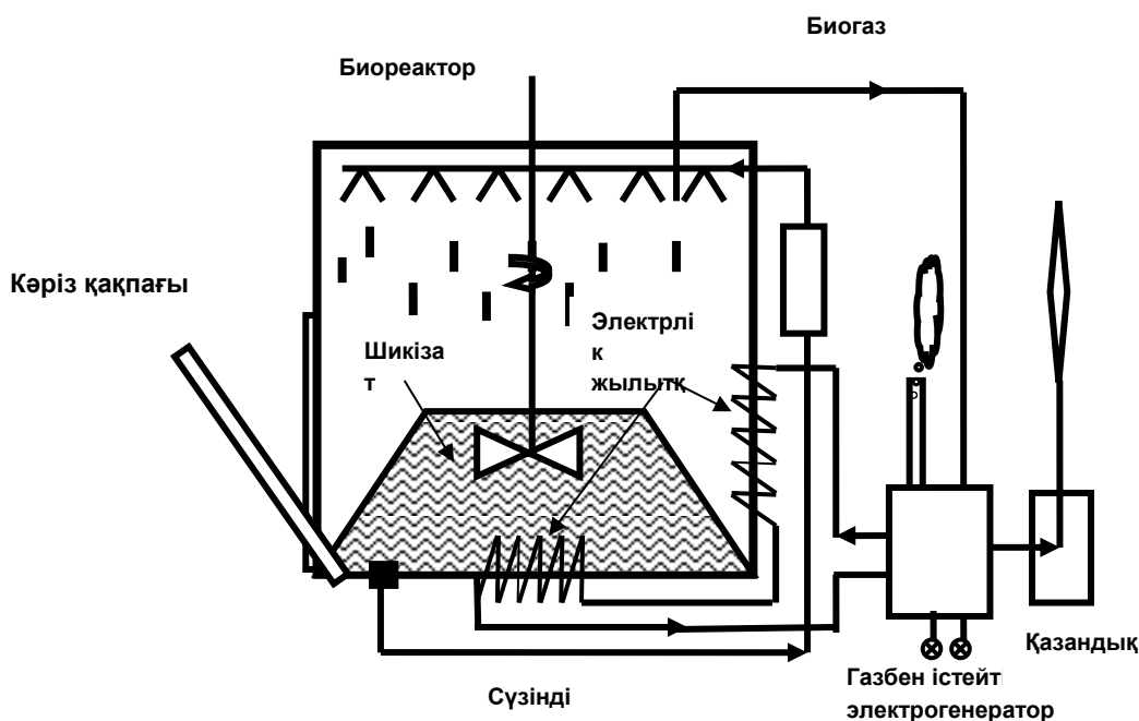
18 сурет – Биогаз қондырғысының қысқаша сызбасы
