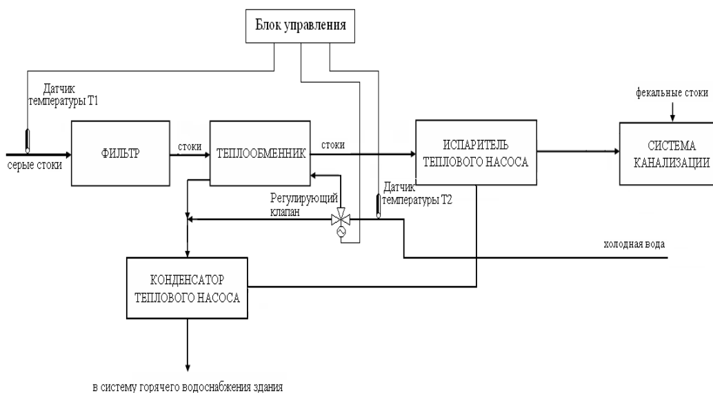
23 сурет – Күн коллекторын пайдаланып коттедж ғимаратын жылу алмастырғыш және жылулық сорғышты пайдалану жолымен жылумен қамту жүйесі
