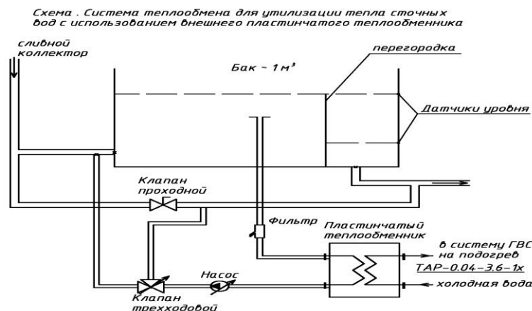
Рисунок 24 - Система теплообмена для утилизации тепла сточных вод с
