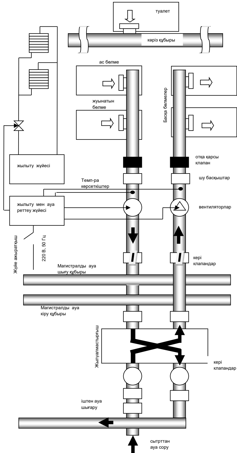
34-сурет – Электрлік ас үй пеші бар коттедж ғимаратын инженерлік жабдықтаудың функционалдық сызбасы
