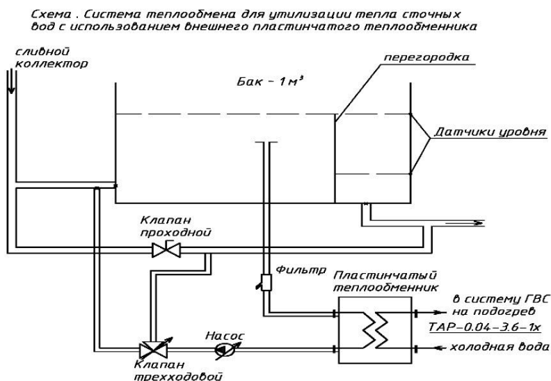
24 сурет –Геотермальді жылыту сорғышының күбі -аккумуляторы мен табақша тәрізді жылу алмастырғышты пайдаланып коттедж ғимаратын аралас жылумен қамту жүйесі
