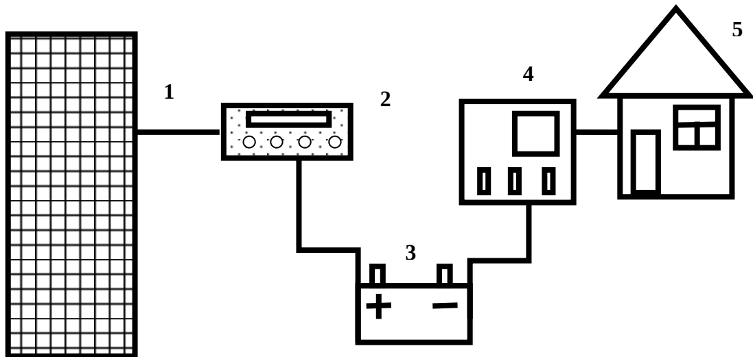
1 – күн тақталары, 2 – қуат контролері, 3 – аккумулятор батареялары, 4 – инвертор 6-сурет – Толық дербес электр энергиясымен күн арқылы қамту жүйесінің негізі элементтері
