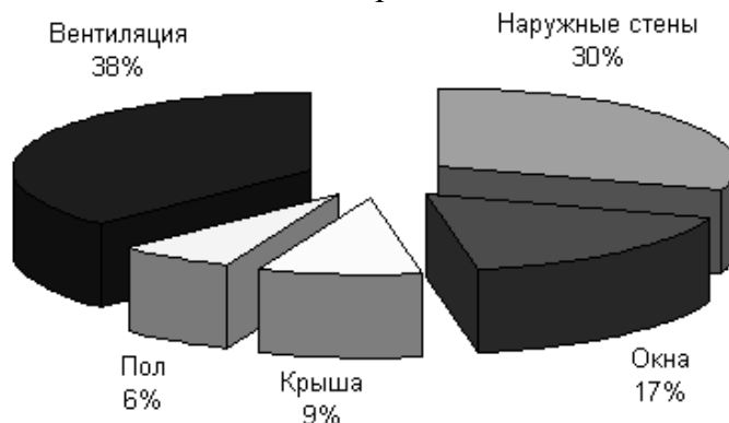
Рисунок 32 – Пример структуры теплопотерь коттеджного здания
