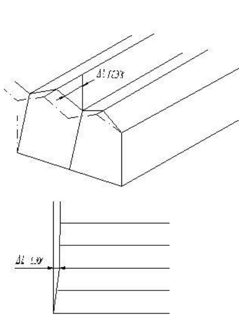
Рисунок А.1 - Горизонтальные смещения теплицы на уровне водосточного желоба в направлении параллельно водосточного желоба
