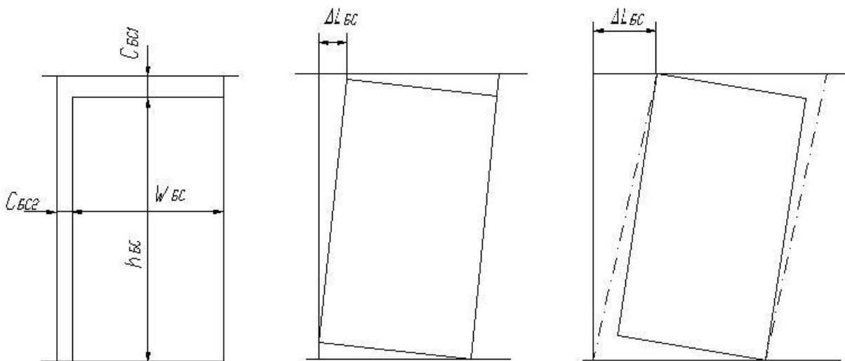
Рисунок А.3 - Параметры, ограничивающие перемещение облицовочной панели для расчета \Delta L_{BC}
