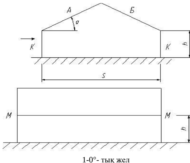
Б.2-суреті – Екі құламалы ангарлық жылыжайлардың қабырғалары мен шатырларына арналған аймақтар
