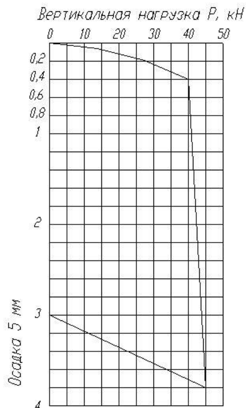
Е.5-суреті – «Қалдық-жүктеме» графикі
