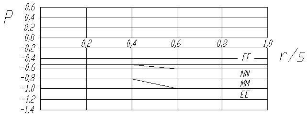
Б.11-суреті – Коньки бағытындағы жел үшін екі құламалы жылыжайлардың қабырғалары мен шатырларына арналған P_H қысымының жергілікті коэффициенттері
