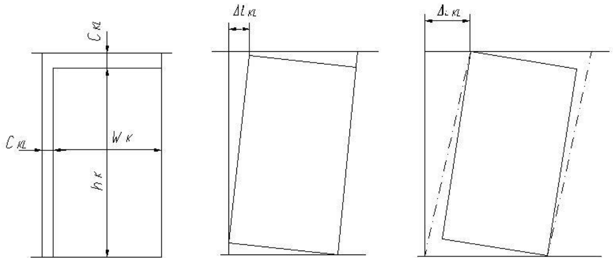
A.5 - суреті - \Delta L_{III} есептеу үшін қаптау тақтасының орын ауыстыруын шектейтін параметрлер
