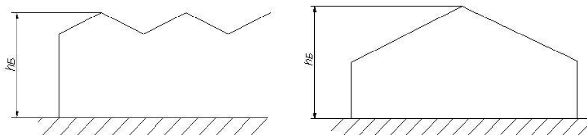
Рисунок Б.1 - Базовая высота h_B для ангарных и блочных теплиц
