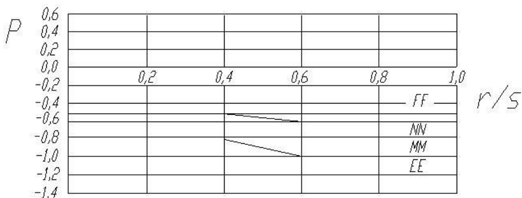
Б.14-суреті – Коньки бағытындағы жел үшін блоктық жылыжайлардың қабырғалары мен шатырларына арналған p_H қысымының жергілікті коэффициенттері
