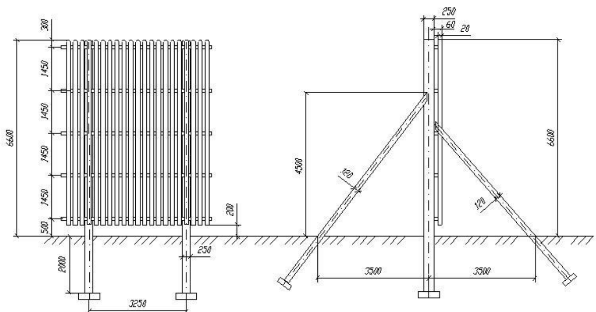
М.4-суреті – Қалыпты керегесі бар ағаш дуалдың түрі
