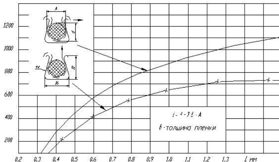
Д.2-суреті– Бекітудің салмақ түсетін қабілетінің бекіту құрылғыларына және үлдір ұалындығының өлшемдеріне қатынасынан тәуелділігі
