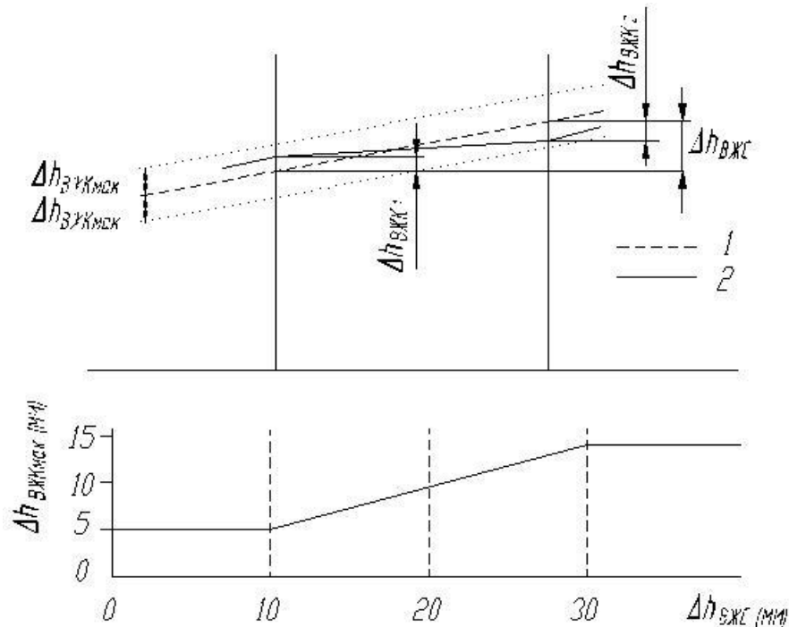
3-сурет – Бағаналар ұштарындағы су ағатын науаның жобалық қалыптан шектік тік жылжуы
