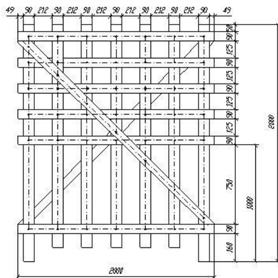
М.2-суреті – Сиретілген керегесі бар қар қалқанының түрі
