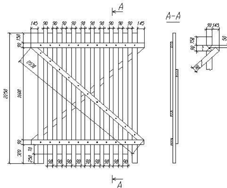
М.1-суреті - Қалыпты керегесі бар қар қалқанының түрі
