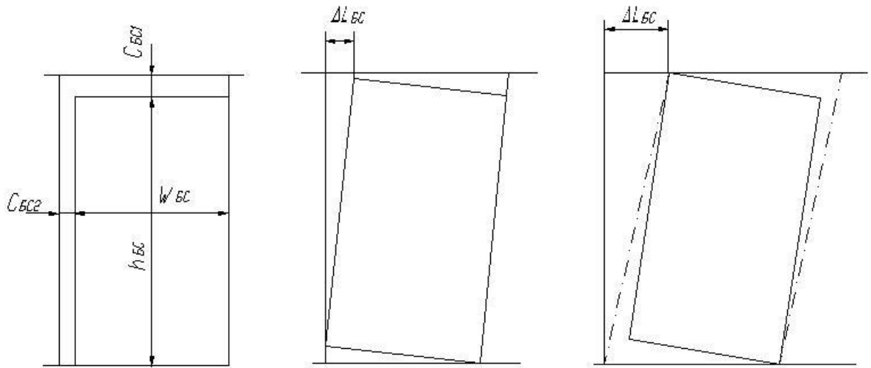
А.3-суреті - \Delta L_{БК} есептеу үшін қаптау тақтасының орын ауыстыруын шектейтін параметрлер
