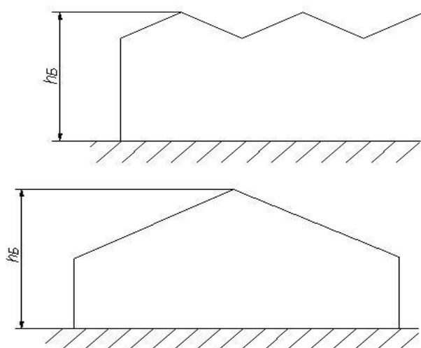
Б.1-суреті – Ангарлық және блоктық жылыжайларға арналған базалық биіктік h_B
