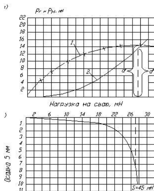
Рисунок Е.7 - Свая-штамп и ходограммы ее нагружения
