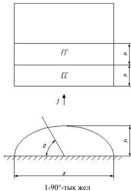
Б.20-суреті – Құламалары (бұғаттары) жоқ ангарлық жылыжайлардың күмбезді шатырына арналған аймақтар
