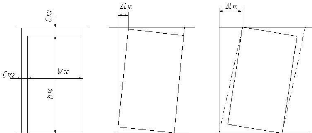
А.4-суреті - \Delta L_{IIIK} есептеу үшін қаптау тақтасының орын ауыстыруын шектейтін өлшемдер
