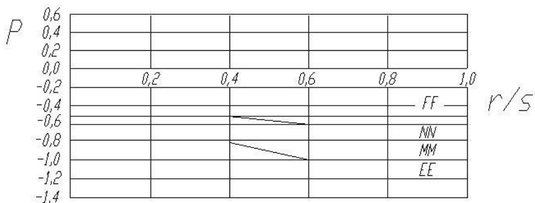
Рисунок Б.14 - Локальные коэффициенты давления r_H для стен и крыш
