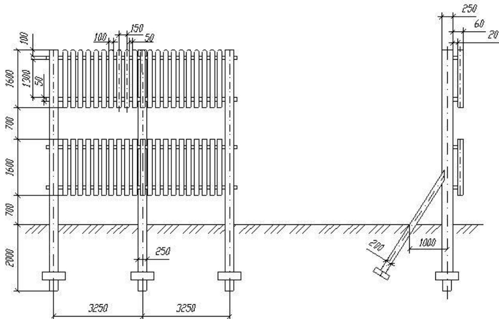
М.5-суреті – Сиретілген керегесі бар ағаш дуал түрі
