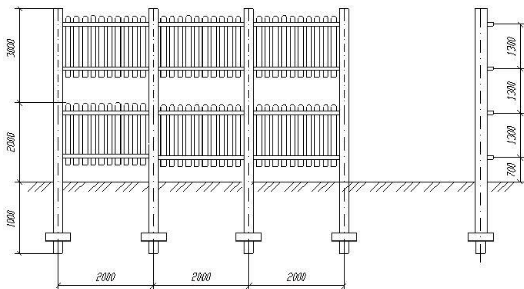
М.6-суреті – Алмалы қалқандары бар ағаш дуалдың түрі
