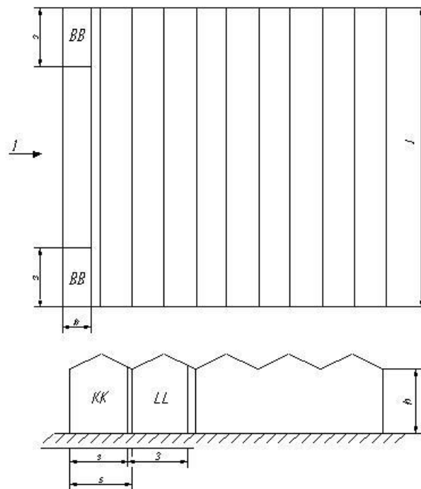
Б.11-суреті – Коньки бағытындағы жел үшін екі құламалы жылыжайлардың қабырғалары мен шатырларына арналған P_H қысымының жергілікті коэффициенттері
