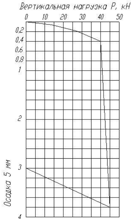
Рисунок Е.5 - График «осадка-нагрузка»
