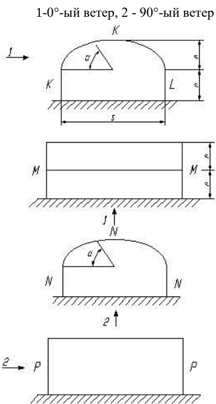
Рисунок Б. 17 - Зоны для сводчатой крыши и стен ангарных теплиц со свесами
