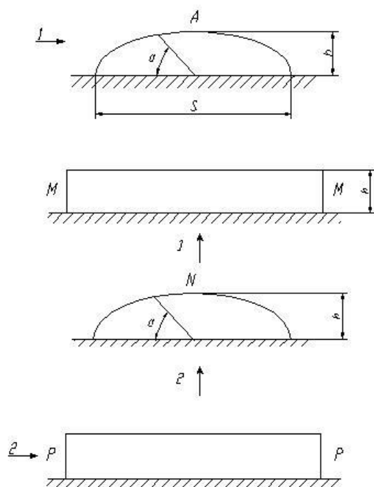
Рисунок Б.16 - Зоны для сводчатых крыш и стен ангарных теплиц без свесов (карнизов) крыш
