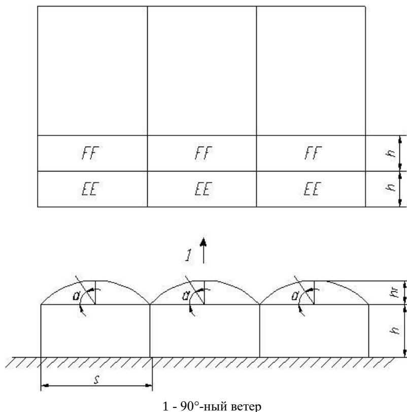
Рисунок Б.23 - Зоны для сводчатой крыши блочных теплиц со свесами (карнизами) и c(h/s) \geq 0,2
