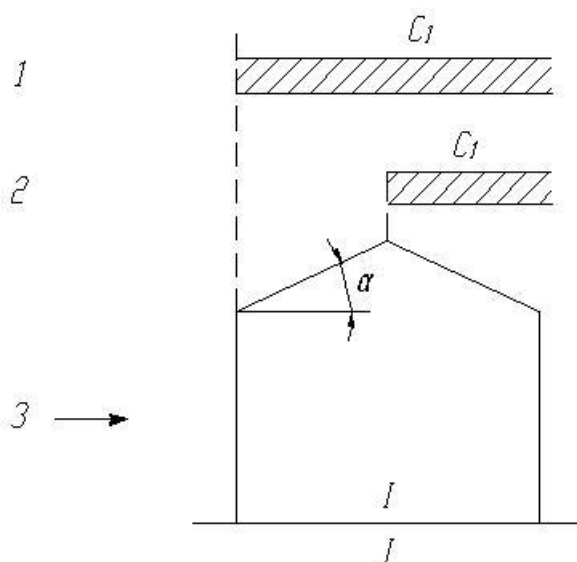
1- равномерная нагрузка, 2- неравномерная нагрузка, 3 - направление ветра
