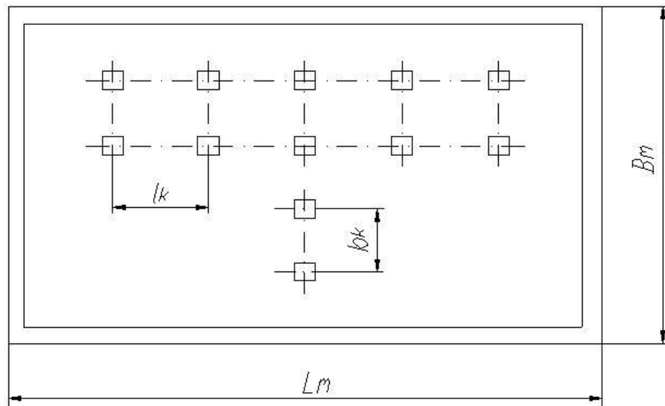
8-сурет -Бағаналар негіздерінің арасындағы көлденең қашықтық
