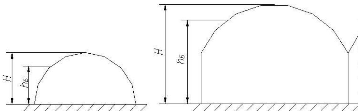
Б.15-суреті – Күмбезді шатырлары бар жылыжайларға арналған h_B базалық биіктік
