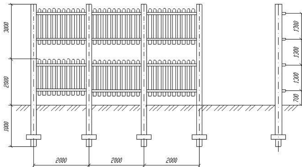
Рисунок М.6 - Вид деревянного забора со съемными щитами
