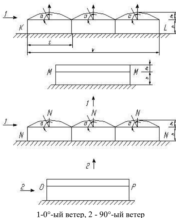
Рисунок Б.19 - Зоны для сводчатых крыш и стен блочных теплиц со свесами крыши (карнизами) и с (h/s) \geq 0,2
