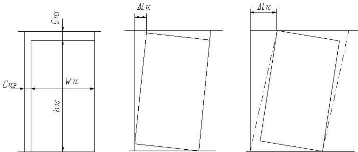
Рисунок А.4 - Параметры, ограничивающие перемещения облицовочной панели для расчета \Delta L_{ТС}
