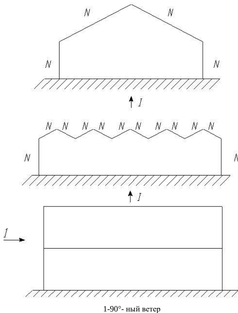
Рисунок Б.7 - Зоны для стен и крыш двускатных и блочных теплиц
