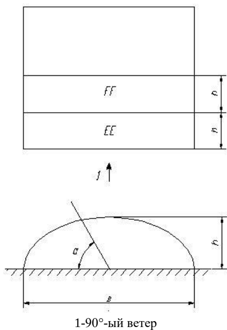
Рисунок Б.20 - Зоны для сводчатой крыши ангарных теплиц без свесов (карнизов)
