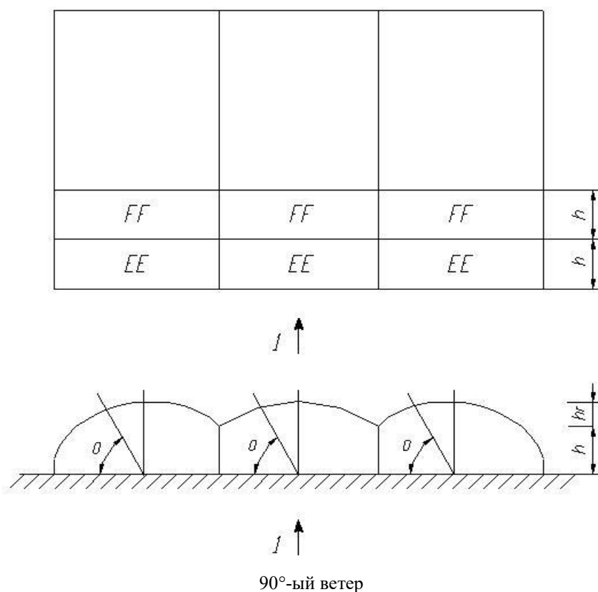
Рисунок Б.22 - Зоны для сводчатой крыши блочной теплиц без свесов (карнизов)1 –
