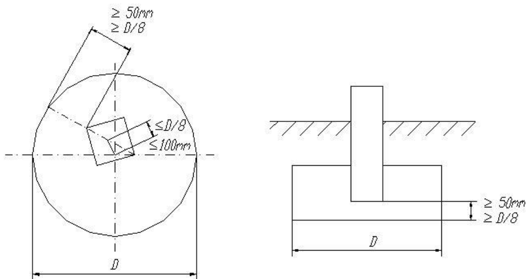
5-сурет – Әзірленген іргетас тіреуінің іргетастағы жетекші ұңғыманың қуысында орналасуы
