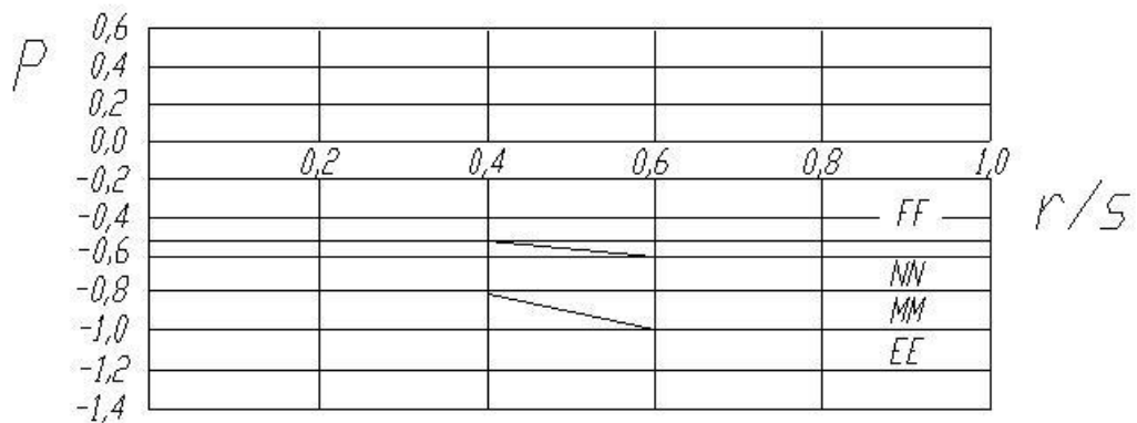
Рисунок Б.11 - Локальные коэффициенты давления p_n для стен и крыш двухскатных теплиц для ветра в направлении конька
