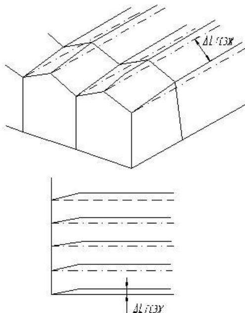
А.2 - суреті - Су ағатын науа деңгейіндегі су ағатын науаға тік бағыттағы жылыжайдың көлденең жылжуы
