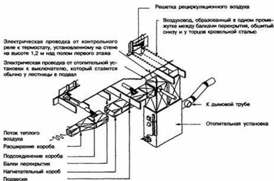
Рисунок 13.4 - Крепление воздуховодов
