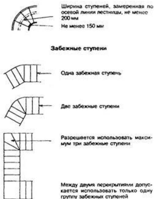
Рисунок 12.1 - Криволинейные лестницы и лестницы с забежными ступенями
