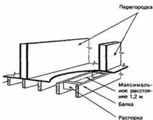
Рисунок 6.13 - Опираие перегородок
