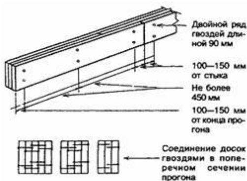
Рисунок 6.1 - Деревянные прогоны составного сечения
