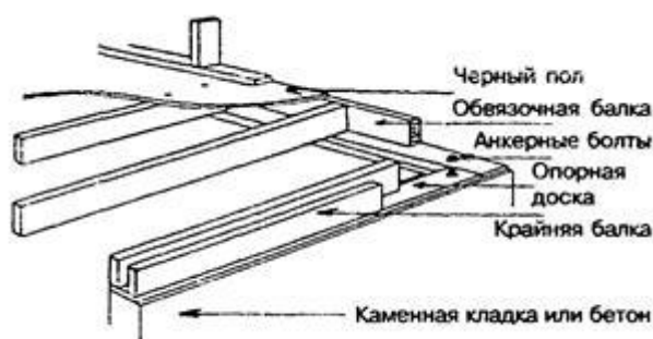
Рисунок 6.4 - Опирающие прогоны (балки) перекрытия на опорную доску, уложенную на фундаментную стену
