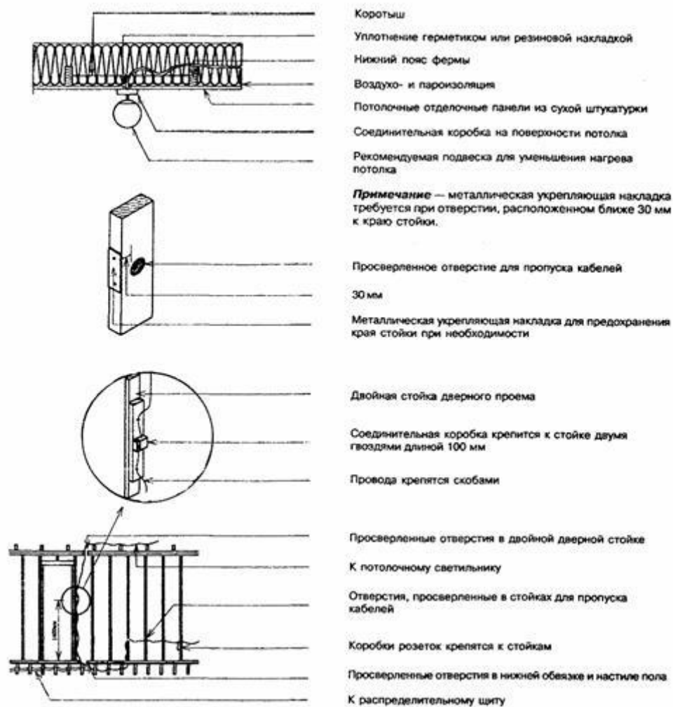
Рисунок 13.9 - Прокладка электрических проводов в элементах каркаса
