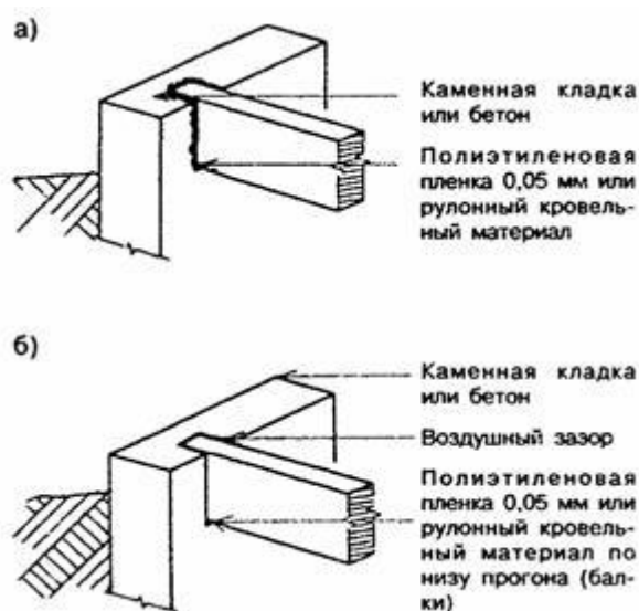
Рисунок 6.3 - Опирающие прогоны (балки) перекрытия с заделкой в фундаментную стену.
