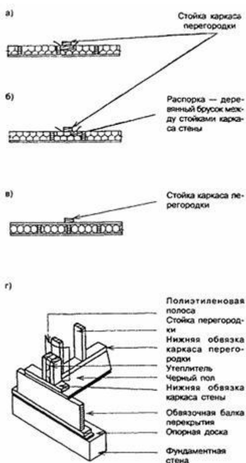
Рисунок 7.3 - Варианты примыкания перегородок к наружной стене
