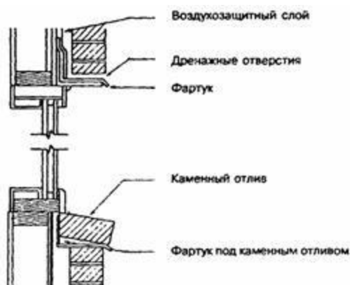
Рисунок 10.2 - Установка фартука под каменным отливом
