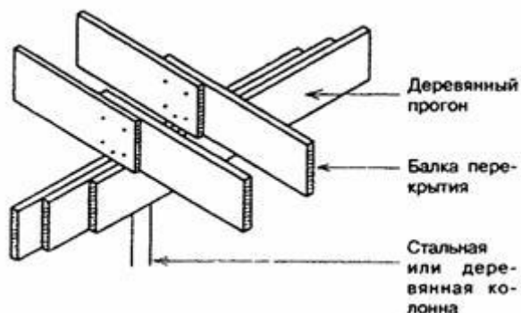
Рисунок 6.7 - Опираие балок перекрытия на деревянный прогон
