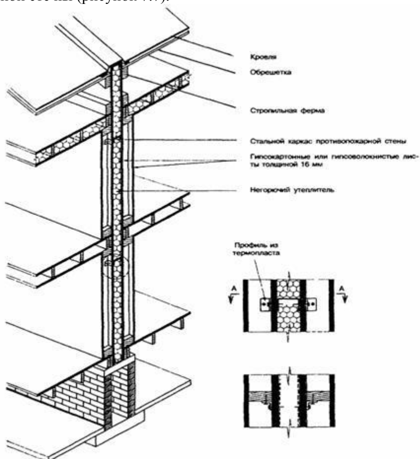
Рисунок 7.6 - Межквартирная противопожарная стена 2-го типа каркасной конструкции
