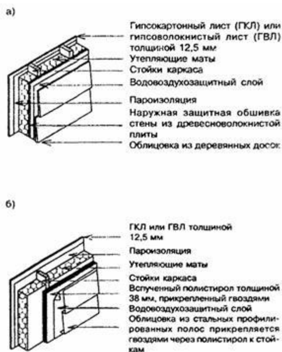
Рисунок 9.1 - Варианты размещения теплоизоляции в каркасной стене
