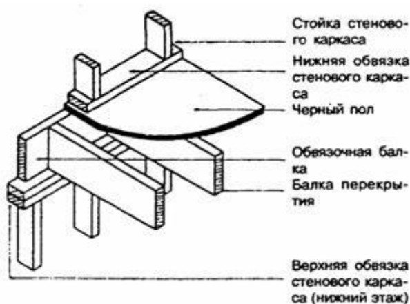
Рисунок 6.6 - Опираие балок перекрытия на каркас наружной стены
