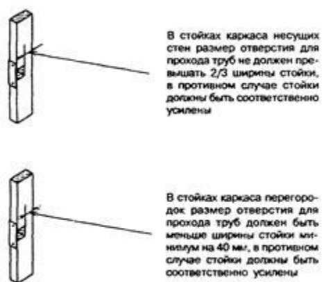
Рисунок 13.7 - Вырезы в стойках каркаса для прохода труб
