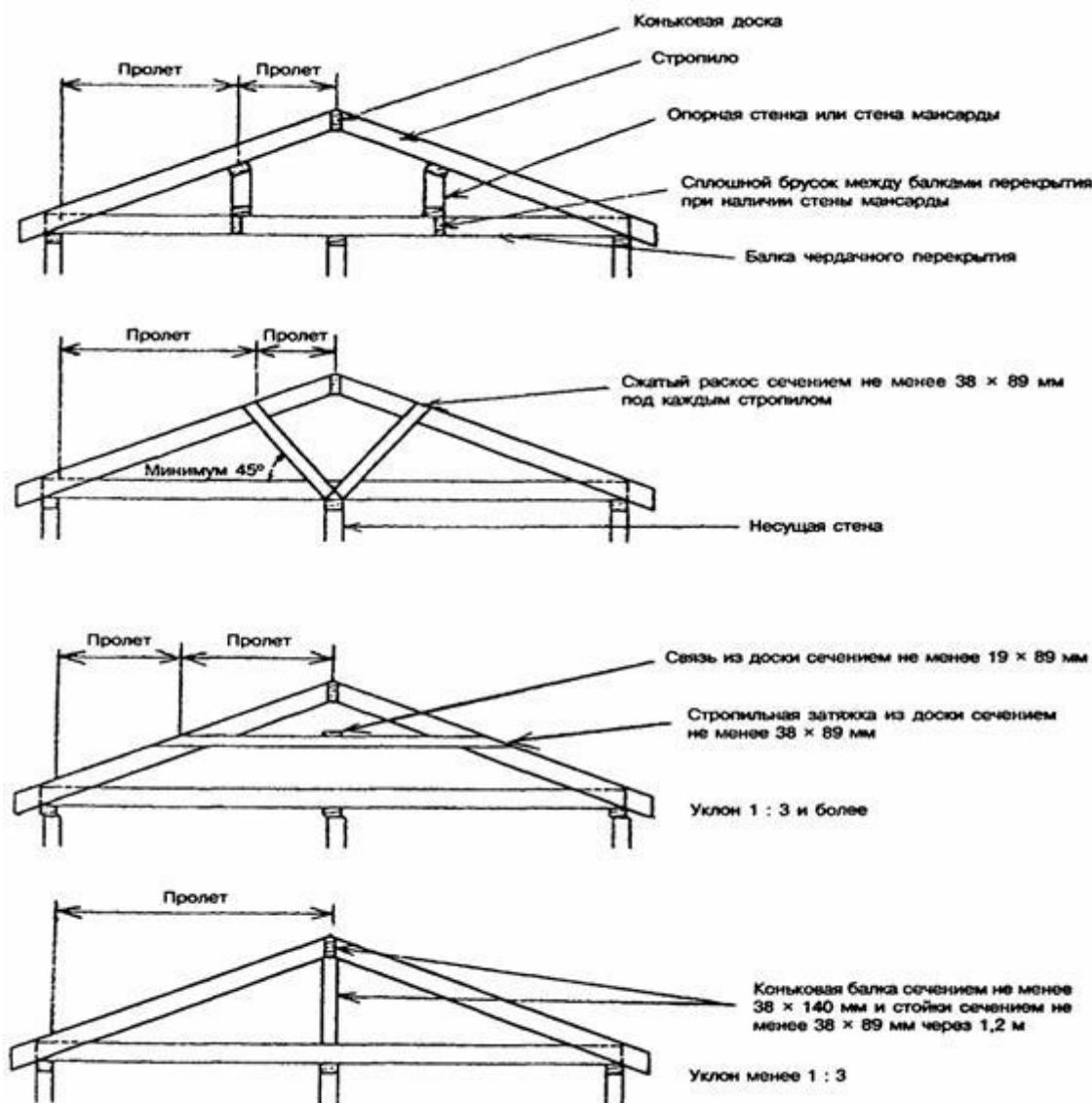
Рисунок 8.1 - Элементы несущего каркаса скатной крыши
