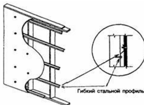
Рисунок 7.8 - Крепление обшивки каркаса для обеспечения звукоизоляции
