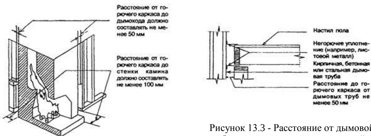
Рисунок 13.2 - Расстояние от стенок камина до каркаса здания
