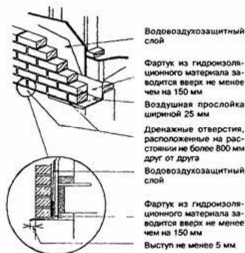
Рисунок 10.3 - Фартук под дренажными отверстиями каменной облицовки
