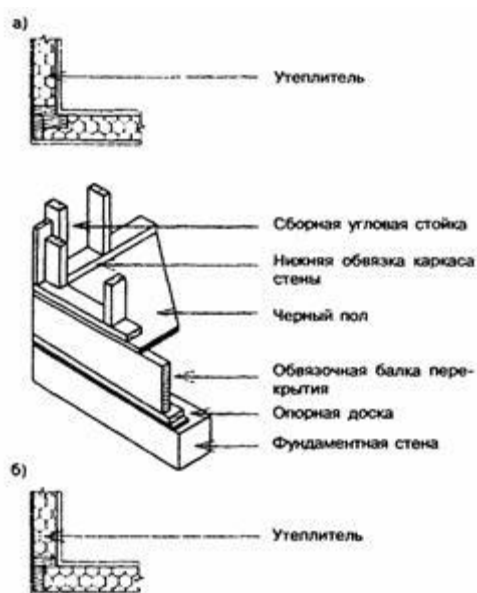
Рисунок 7.2-Угловое соединение несущих стен
