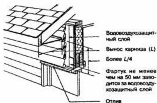
Рисунок 10.4 - Фартук над оконным (дверным) проемом
