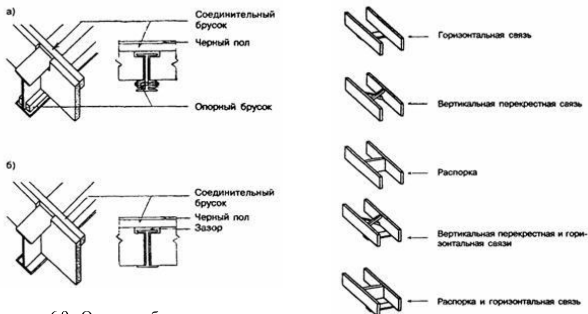
Рисунок 6.9 - Опираие балок перекрытия на стальные прогоны
