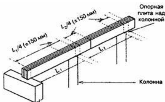
Рисунок 6.2 - Стыки досок в неразрезных прогонах составного сечения
