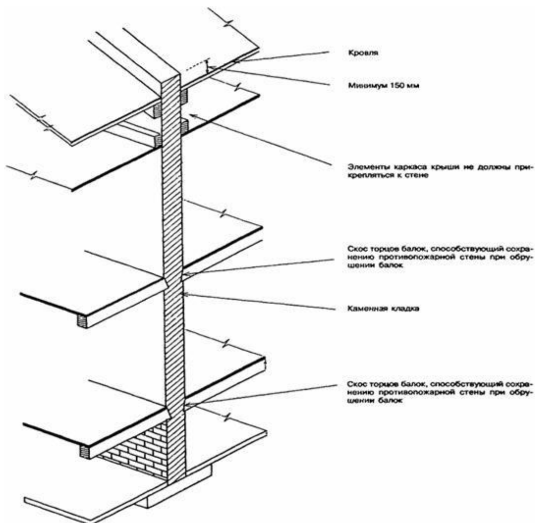
Рисунок 7.5 - Каменная противопожарная стена
