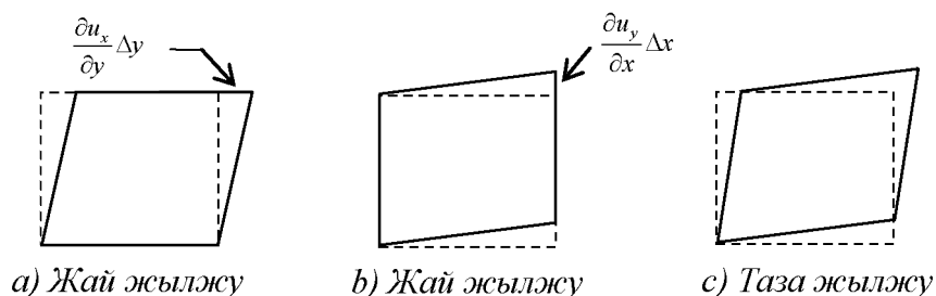
А.2-суреті – Жылжу деформациялары
