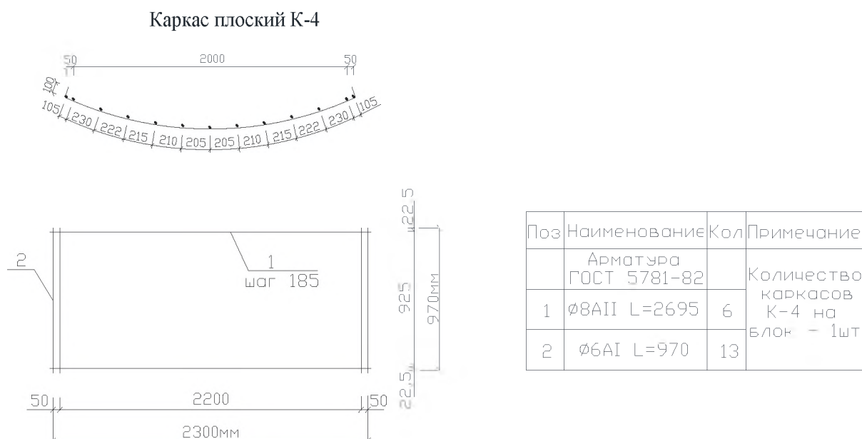
Рисунок Л.20 – Опалубочный и арматурные чертежи лоткового блока
