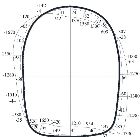
Рисунок Ж.3 - Эпюры усилий (сплошная линия и пунктир) в обделке при действии волны сжатия, падающей под углом 120^\circ к направленной вверх оси симметрии
