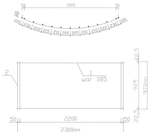
Л.20-суреті – Науалық блоктың қалыптық және арматуралық сызбалары
