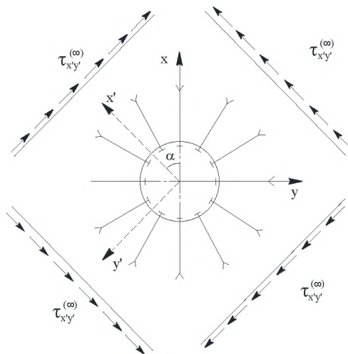
Рисунок 16 – Расчетная схема для определения продольных сил в анкерных стрижнях от действия длинной поперечной волны
