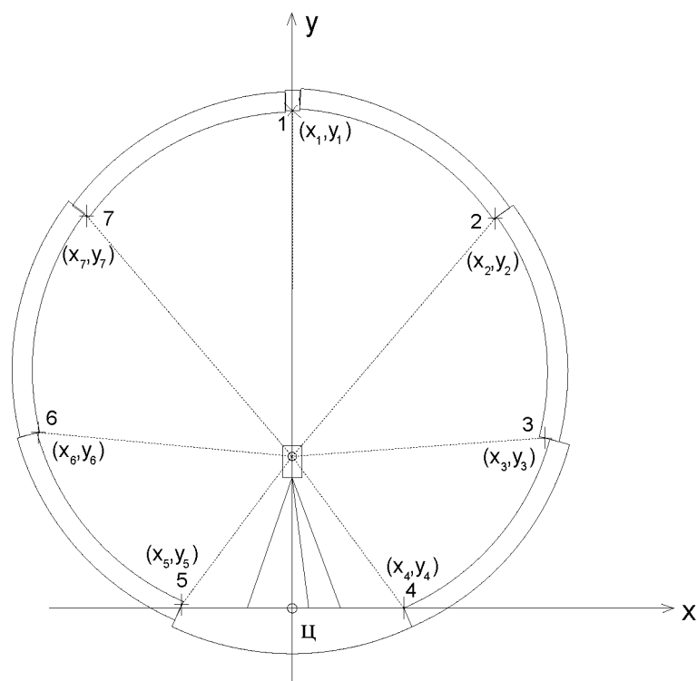
Л.2-суреті – Тахеометрдің төменгі нүктесіне қатысты қаптама блоктары түйіспелерінің координаттарын анықтауға:
