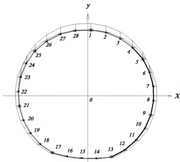
Л.10-суреті – Қаптама сақинасының есептік тәсілі және оның жүктелуі
