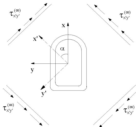
3-сурет – Көлденең сейсмикалық толқындардан қаптаманың кернеулі жағдайын анықтауға есептік тәсіл
