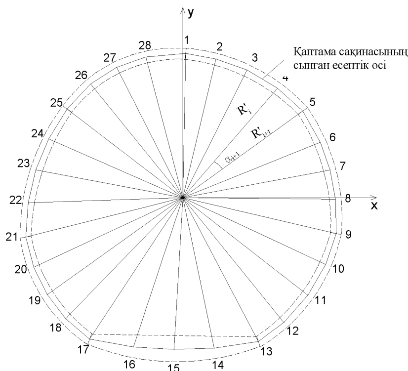
Л.7-суреті – Қаптаманың есептік өсін анықтайтын көпбұрыш шындарының аралық бұрыштарын, радиустарын және координаттарын анықтауға: 1÷28 – көпбұрыш шындары
