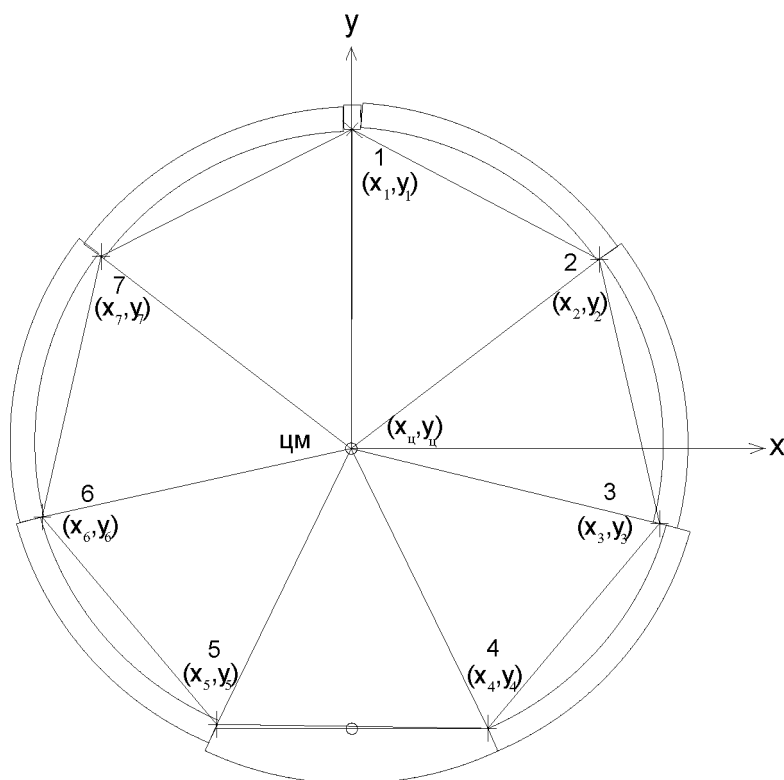
Л.4-суреті – Көпбұрыш орталығына қатысты қаптамалар блоктарының түйіспелері координаттарын анықтауға: цм – көпбұрыш орталығы
