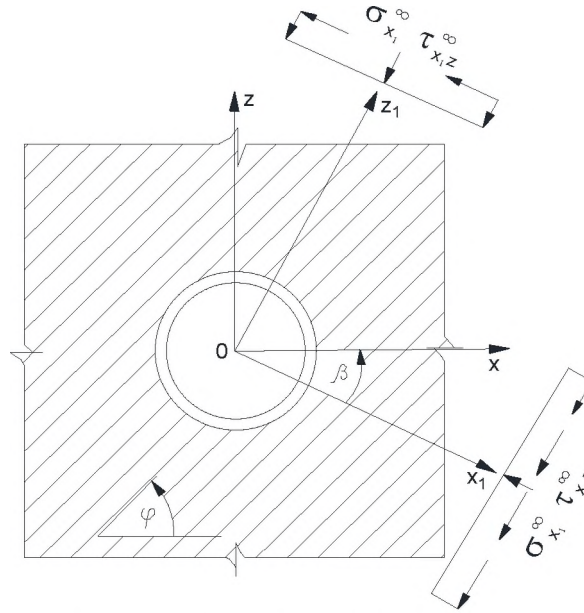
Рисунок 8 – Расчетная схема
