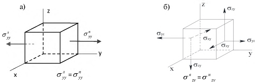
А.4-суреті – Тепе-теңдік кезінде кернеулер арасындағы арақатынас
