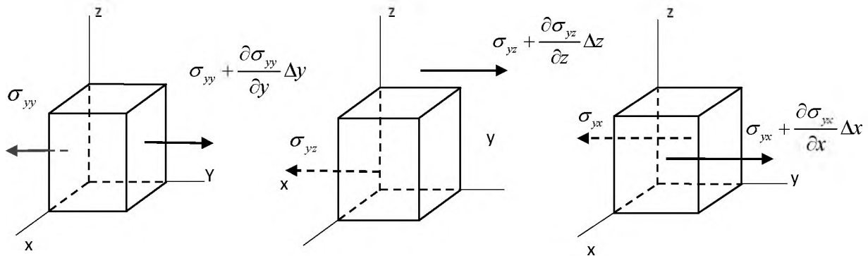
А.5-суреті – y өсінің бағытында қарапайым параллелепипедке әсер ететін ернеулер
