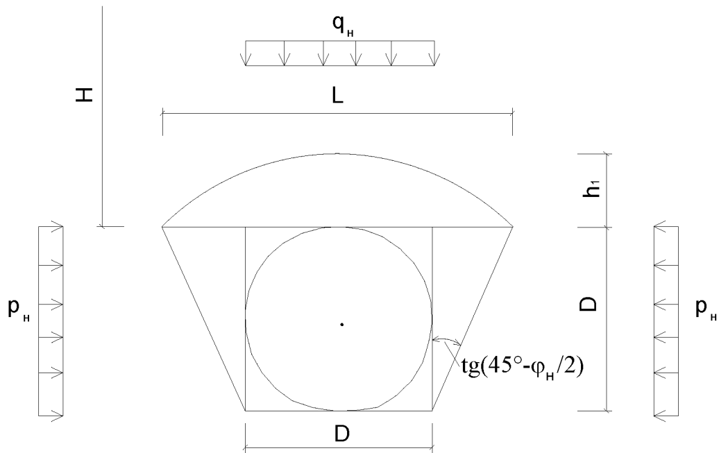
Л.9 –суреті – Қаптаманың сақинасына тау қысымын анықтауға арналған тәсіл
