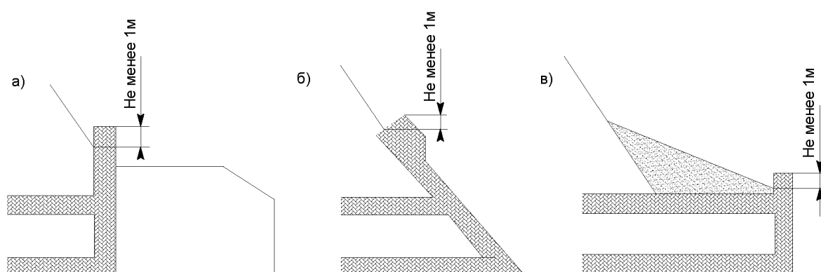
Рисунок 20 - Конструкции порталов тоннелей в сейсмических районах а – врезной, б - с наклонной лобовой подпорной стеной, в - выносной
