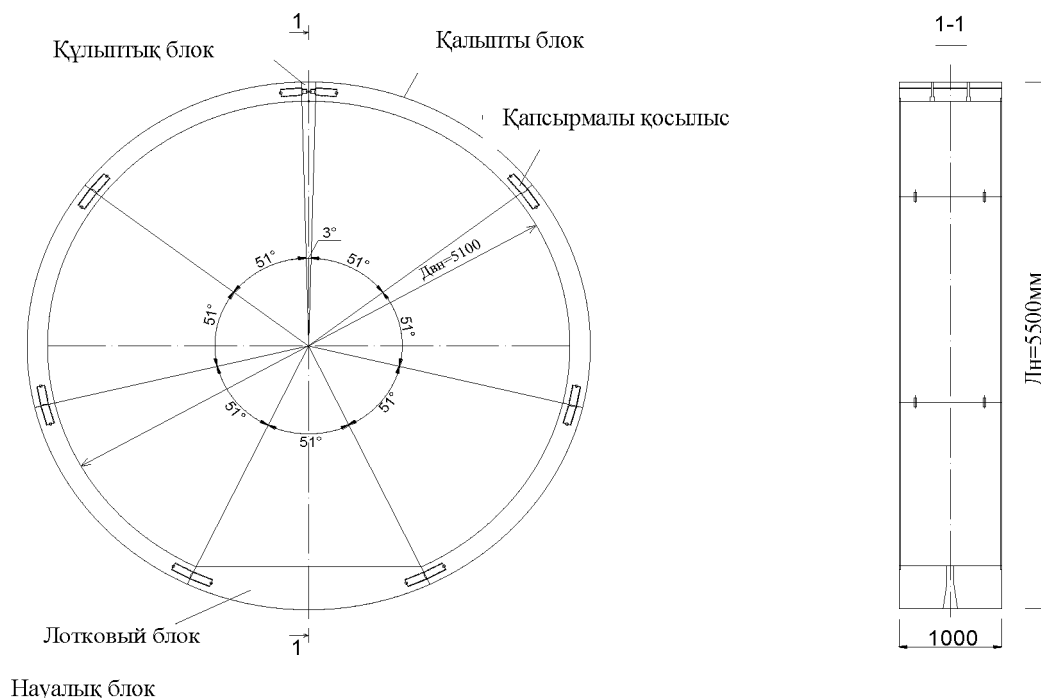
Л.1-суреті – Құрама темірбетон блоктардан тұратын айналма туннельдік қаптама сақинасының жобалық кескіні
