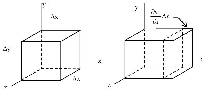
А.1-суреті – Деформация түрі. Қарапайым созылу
