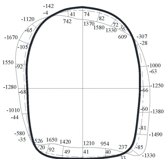
Ж.4-суреті – Қаптамадағы күштердің эпюралары (тұтас сызық және пунктир)
