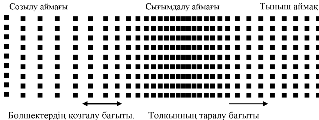
Б.1-суреті – Топырақ бөлшектерінің бойлық қозғалыстары
