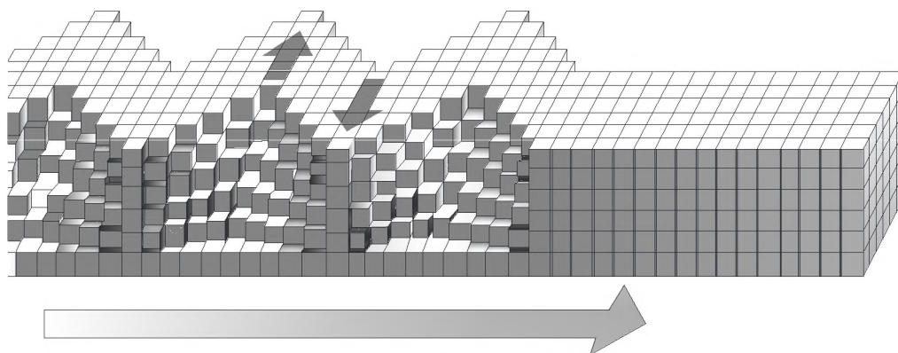
Б.5-суреті – Ляв толқыны таралған кезде топырақтың беткі қабаттарының деформациялануы
