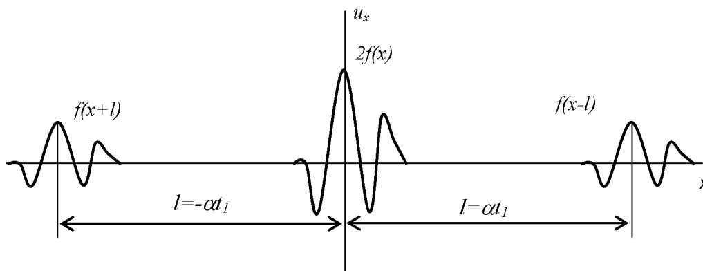
Б.2-суреті – Толқынның таралу мысалы
