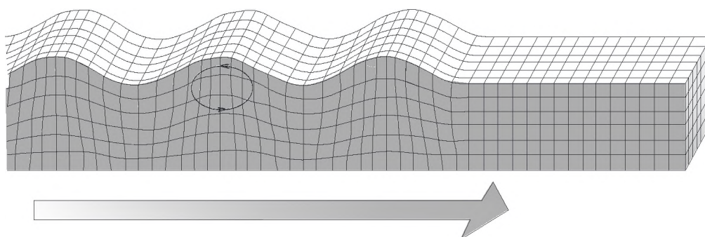
Б.6-суреті – Рэле толқындарының таралуы кезінде топырақтың беткі қабаттарының деформациялануы
