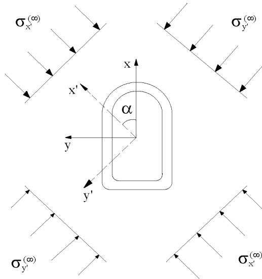
2-сурет – Бойлық сейсмикалық толқындардан қаптаманың кернеулі жағдайын анықтауға есептік тәсіл
