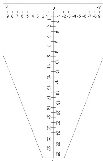
И.2-суреті - u_n^{(0)} мәндерін анықтауға арналған палетка
