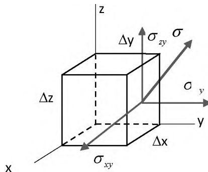
А.3-суреті – Параллелепипедтің қырына әсер ететін кернеулердің көрінісі
