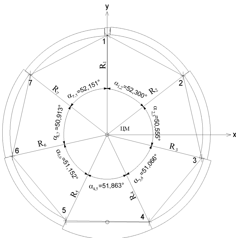
Рисунок Л.5 – К определению радиусов и углов стыков блоков обделки: R_1 \div R_7 – радиусы стыков, \alpha_{1,2} \div \alpha_{7,1} – углы стыков
