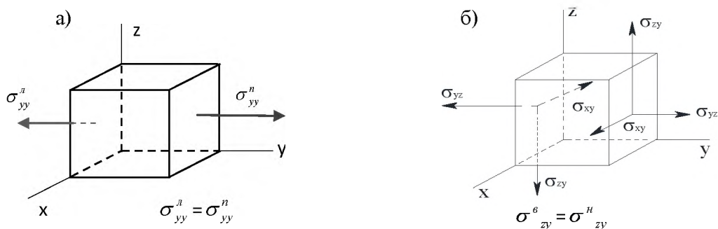
Рисунок А.4 – Соотношения между напряжениями при равновесии
