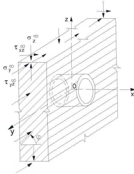
Рисунок 9 – Расчетная схема
