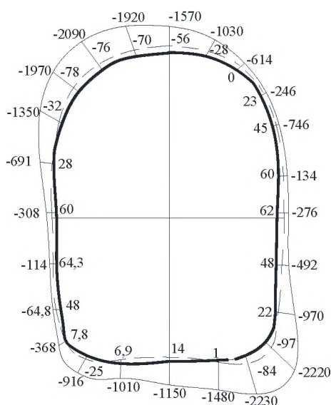
Ж.3-суреті – Жоғары бағытталған симметрия өсіне 120^\circ бұрышынан түсетін сығымдалу толқынының әсерінде қаптамадағы күштердің эпюралары (тұтас сызық және пунктир)
