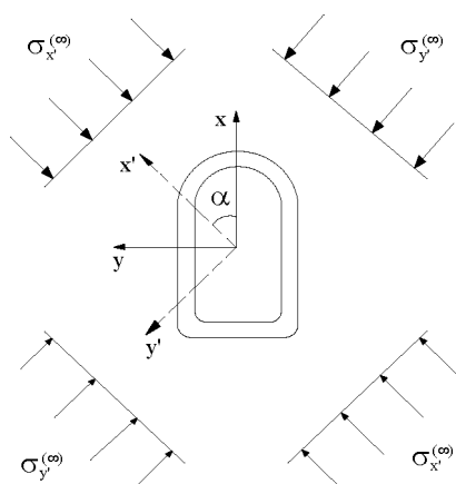
Рисунок 2 – Расчетная схема к определению напряженного состояния обделки от продольных сейсмических волн
