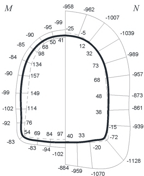
Ж.5-суреті. Теміржол туннелінің қаптамасындағы күштердің есептік эпюралары.
