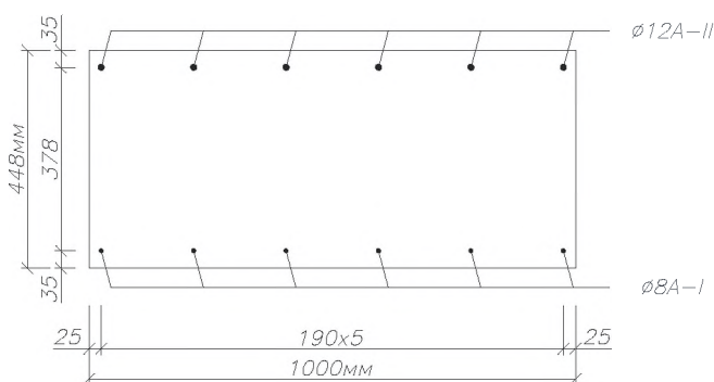
Л.22-суреті – Науалық блокты арматуралау тәсілі
