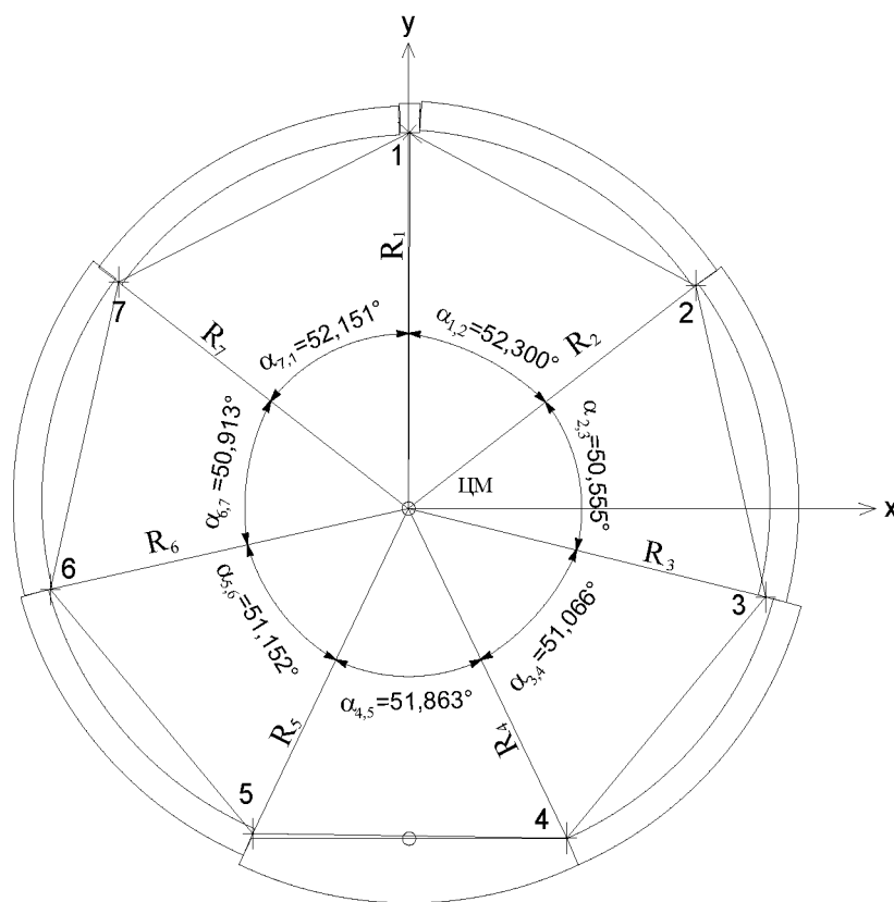
Л.5-сурет і– Қаптама блоктары түйіспелерінің радиустарын және бұрыштарын анықтауға:
