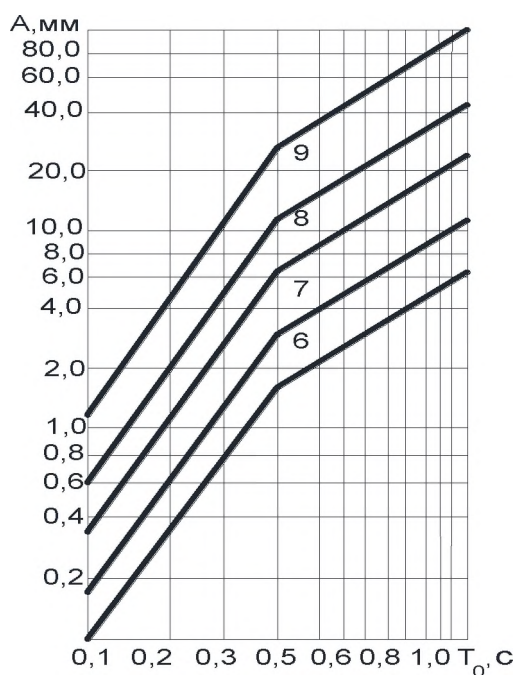
1-сурет – 6÷9 баллдық қарқындылықты жер сілкінісінен туындаған топырақ тербелісі кезінде T_0 кезеңдерінің және A ауысу амплитудаларының арақатынасы
