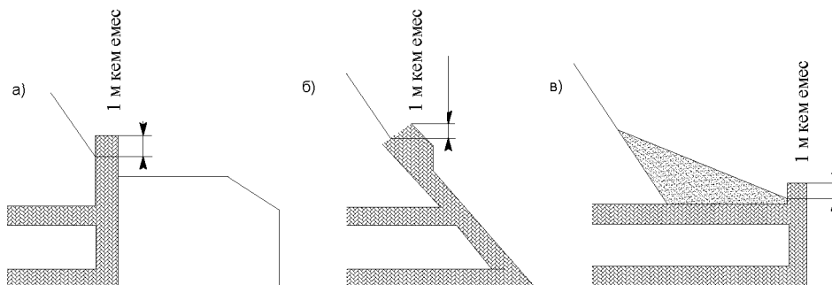
а – ойып орнатылатын, б – еңісті қарсы тіреуіш қабырғамен , в - шығыңқы 20-сурет – Сейсмикалық аудандардағы туннельдер порталдарының конструкциялары
