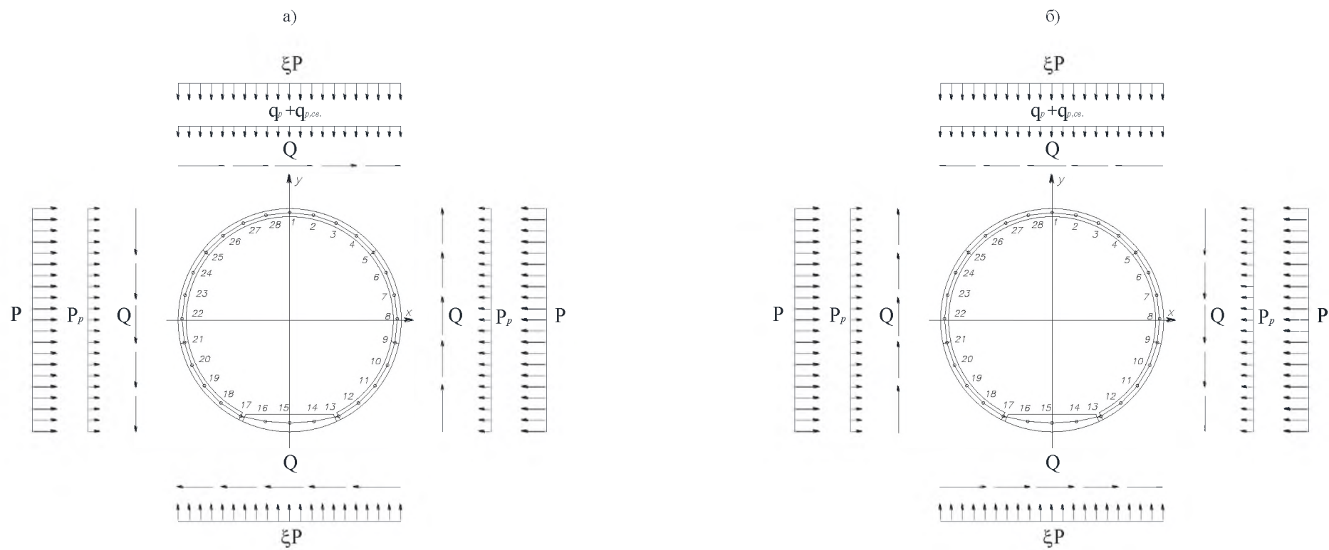
13-суреті – Жүктемелер әрекетінің ерекше үйлесімінде қаптама сакинасының есептік тәсілдері
