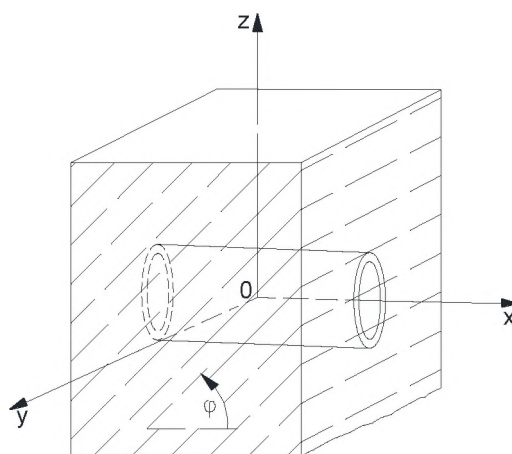
Рисунок 6 – Расчетная схема
