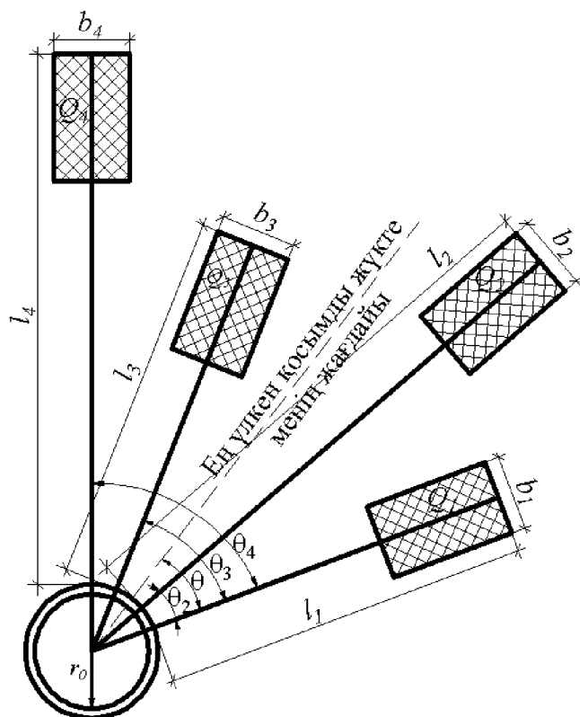
Б.1-сурет – Діңге жақын орналасқан ғимараттардан (имараттардан) пайда болатын жүктемелерді есептеуге арналған сұлба
