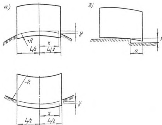
Рисунок И.1 Схемы вертикальных перемещении земной поверхности при подработке, вызванных кривизной (в) или образованием уступа (б)
