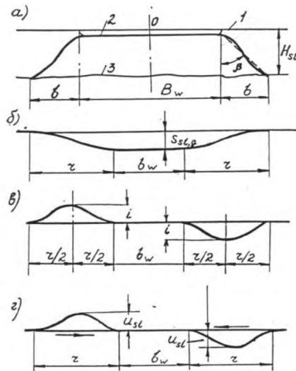
1-сурет – Шөгінді ойылма шегіндегі жер үстінің деформациясының даму сипаттамасы
