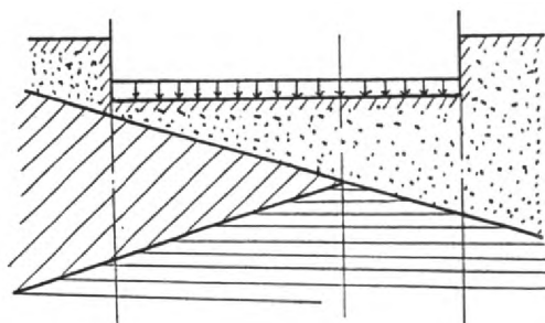
П.9.1-сурет – Біртекті емес іргенің геологиялық кесігі
