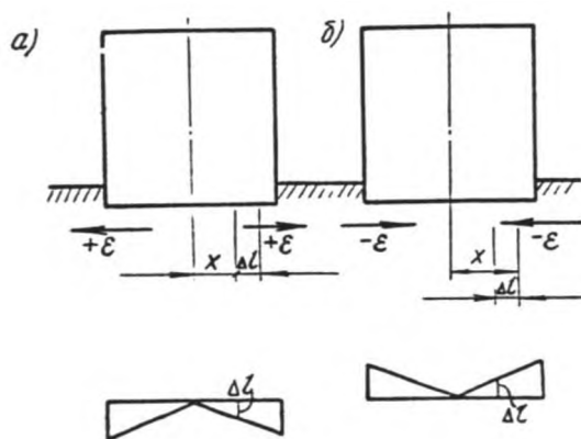
Рисунок И.2. Схемы к расчету перемещений точек земной поверхности под воздействием горизонтальных деформаций
