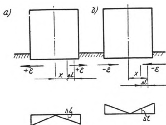
И.2-сурет – Горизонталь деформацияның әсер етуінен жер бетінің нүктелерінің орын ауысуын есептеуге арналған схемалар
