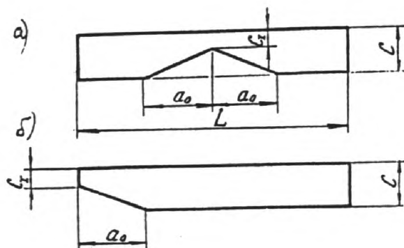
И.5-сурет – Шөгінділігі бойынша I типті топырақ жағдайындағы ірге қаттылығының өзгеру схемалары
