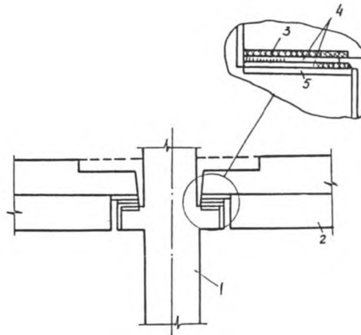
Рисунок Г.2 - Конструкция узла сопряжения ригелей с колонной
