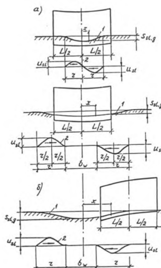
И.3-сурет – Топырақ сыртқы жүктемеден отырған кездегі ғимараттың (имараттың) іргесінің вертикаль орын ауысуының схемалары
