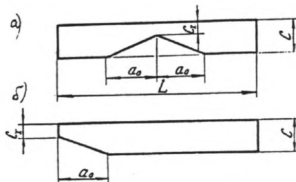
Рисунок II.5. Схемы изменения жесткости основания в грунтовых условиях 1 типа по просадочности
