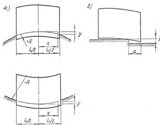
И.1-сурет – Қисықтан (а) немесе шыңның туынан (б) пайда болған өңдеу кезіндегі жер бетінің вертикаль орын ауысуының схемалары
