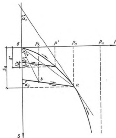
К.2-сурет – сызықтық емес деформацияланатын іргелерге арналған шөгінді мен қысым (дұрыс байланыс кернеуі) арасындағы есептік тәуелділік
