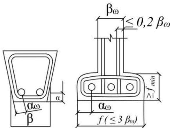
В.1-суреті - Аркалықтарды және арматура өсіне дейінгі арақашықтықты арматуралау
