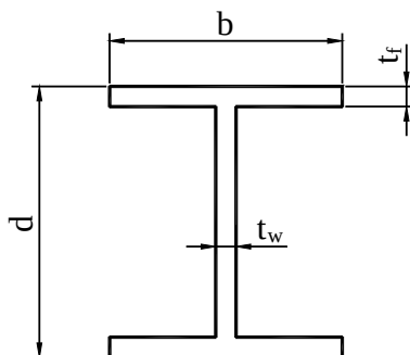
6.1 – сурет. Қос таврлы көлденең қиманың звеносына арналған белгілерді анықтау
