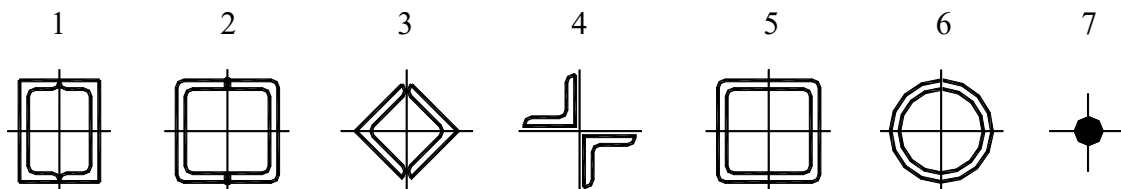
Рисунок А.15 – Сечения связей
