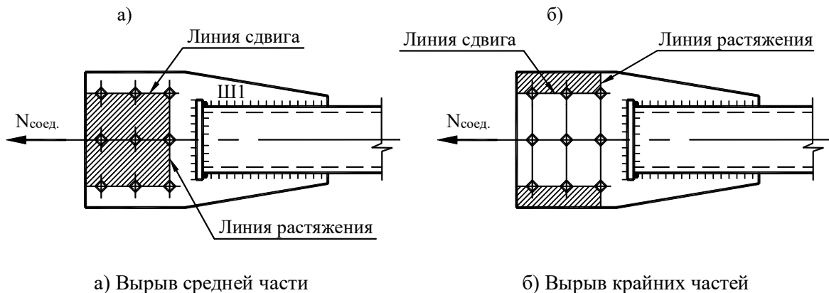
Рисунок Д.20 – Схемы вырыва материала врезной фасонки элемента связи
