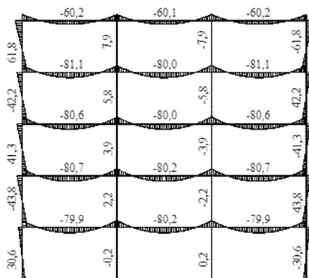
Рисунок Д.10 – Эпюры изгибающих моментов M_{Ed,G,y} от гравитационных нагрузок (ряд Б)
