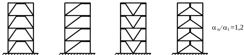
2.4-сурет. Эксцентристiк байланыстары бар қанқалар (диссипативтік аймақтар майысуға және ығысуға жұмыс iстейтiн сейсмикаға қарсы звеноларда).
