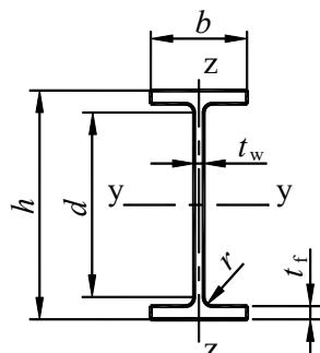
Рисунок Г.13 – Размеры сечения двутавровой колонны первого и второго этажей
