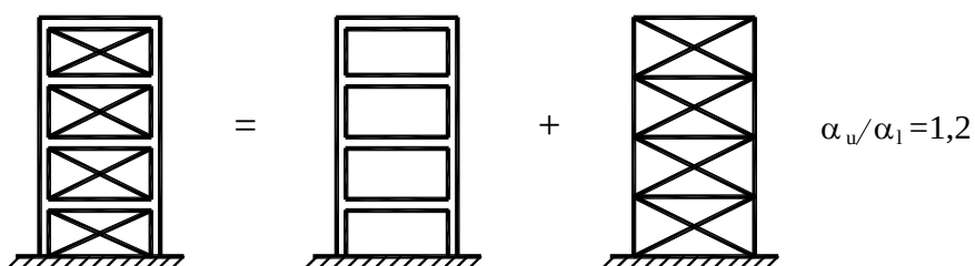
2.7 – сурет. Шоғырланған байланыстармен үйлестірілген моменттік жақтаулы қаңқалар (диссипативтік аймақтар моменттік жақтауда және созылған диагональдарда).
