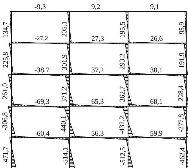
Д.12 – сурет. Сейсмикалық күштерден иілу моменттерінің M_{Ed,E,y} эпюрасы (Б қатары)
