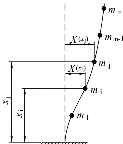
Рисунок В.4 – К определению значений коэффициентов \eta_{ik}
