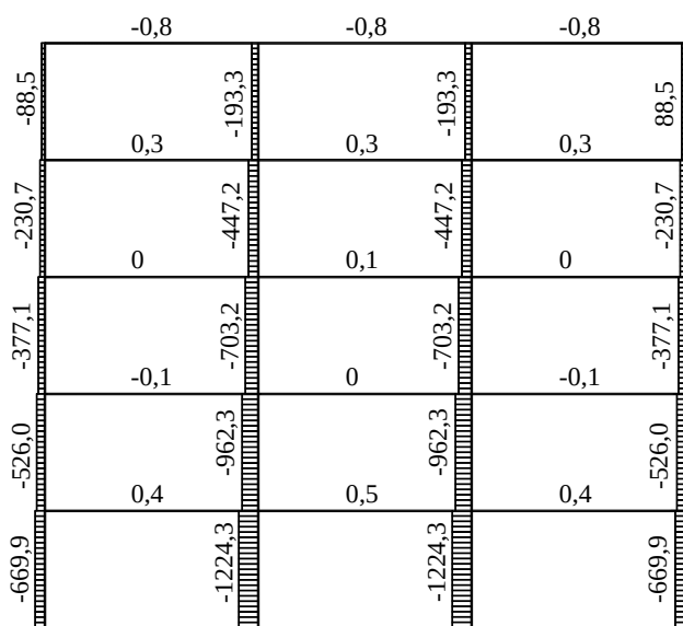
Д.9 – сурет. Гравитациялық күштерден
