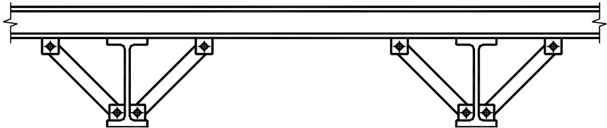
2.14 сурет– Бұралудан типтік қатты бекіту
