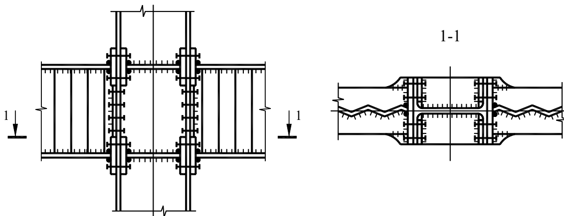
Рисунок А.8 – Болтовое соединение ригелей с колоннами двутаврового сечения
