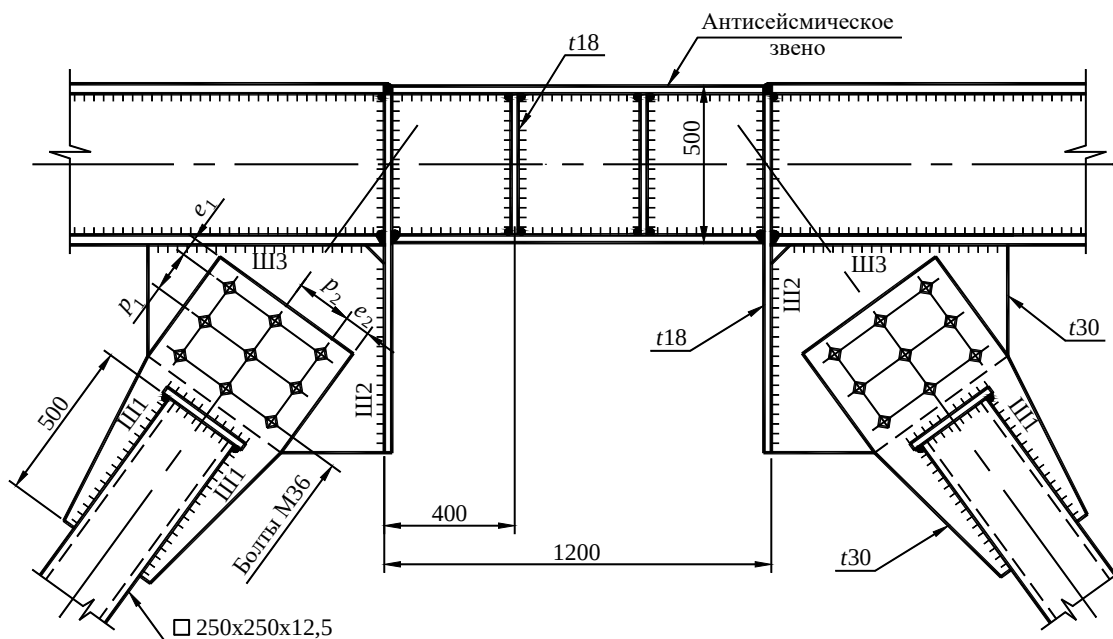
Д.19 –сурет – Эксцентрлік байланыстарды бекіту түйінінің кестесі және антисейсмиялық буын
