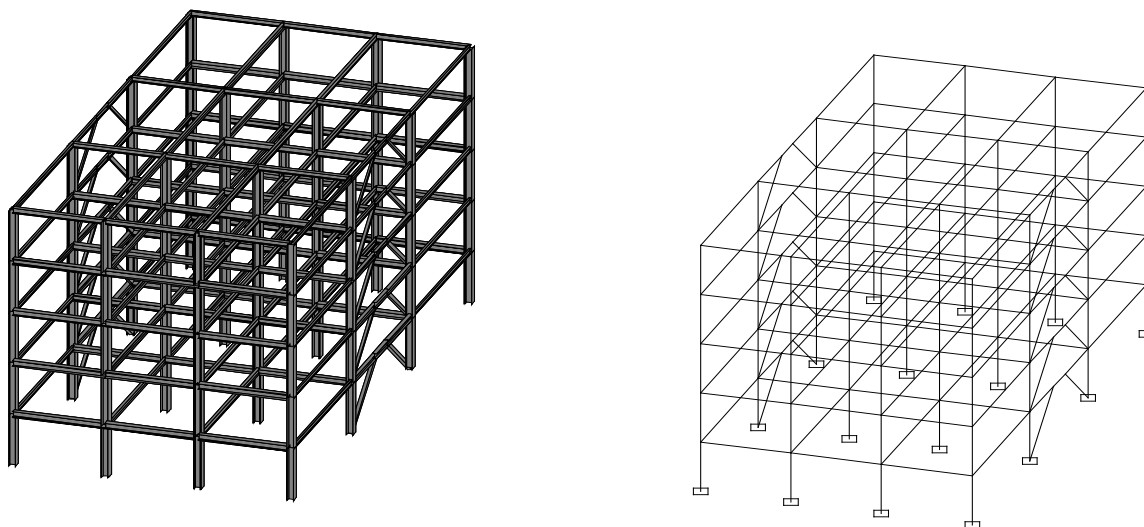
Д.3 – сурет. Ғимараттың конструктивтік және есептік моделі
