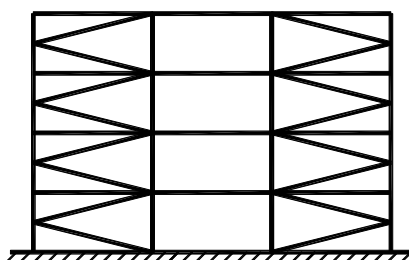
Рисунок 2.9 – Каркас с К-образными связями (не допускается к применению)
