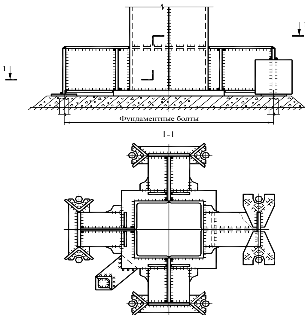
Рисунок А.14 – База колонны квадратного трубчатого сечения
