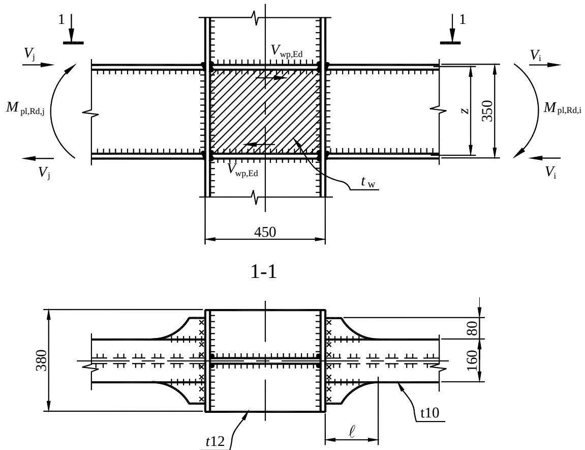
Д.2 2 сурет – Ұстынға арқалық-ригелін бекіту торабы
