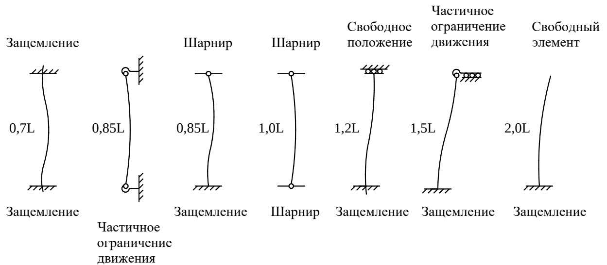
Е.2 сурет – Қысылған элементтердің L_{cr} есептік ұзындығының номиналды есептік ұзындықтары
