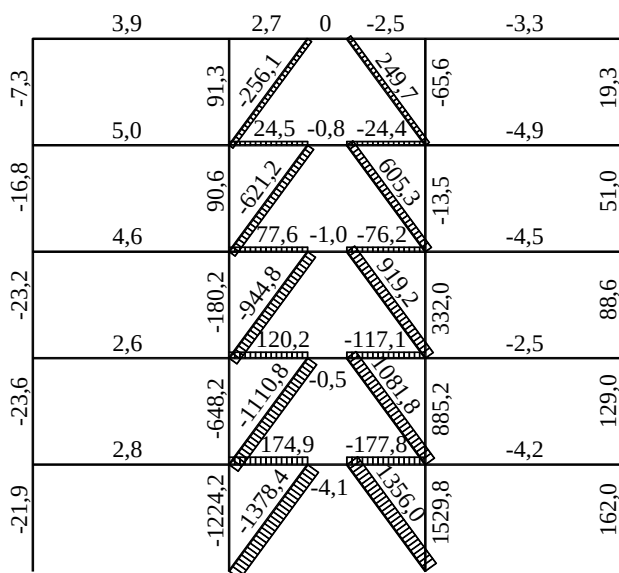
Д.13 – сурет. Сейсмикалық күштерден осьтік күштердің N_{Ed,E} эпюрасы (1-ось)
