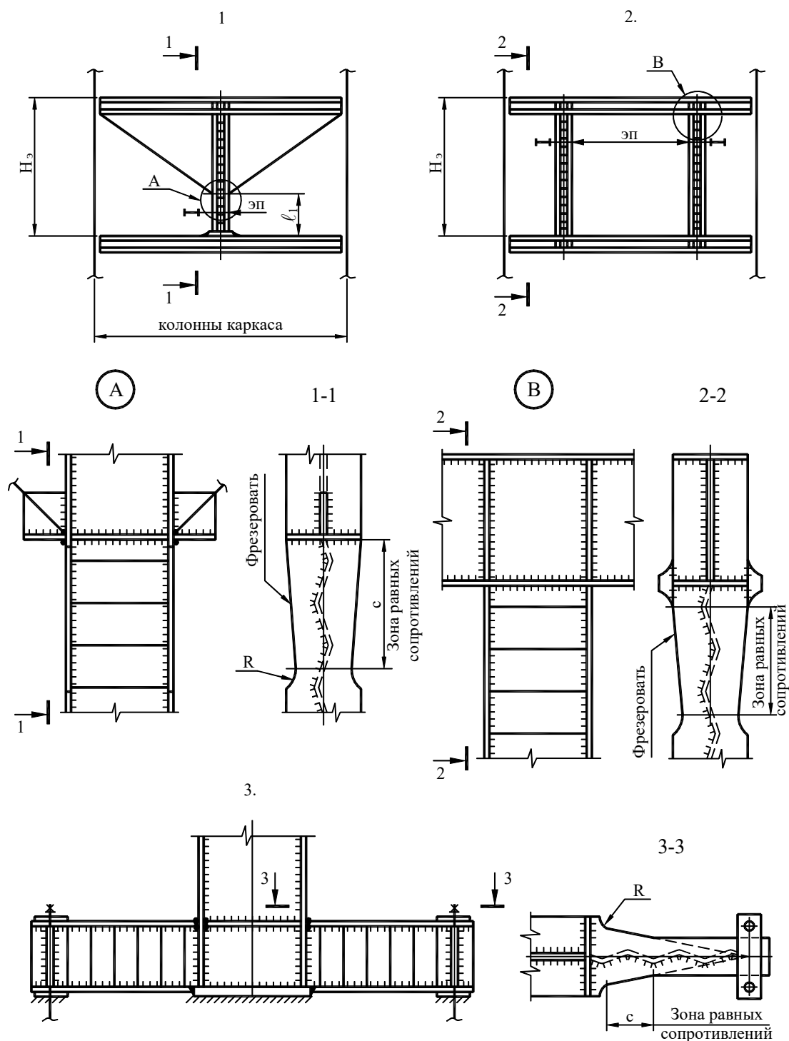
Рисунок Б.4 – Энерглопоглотители балочного типа
