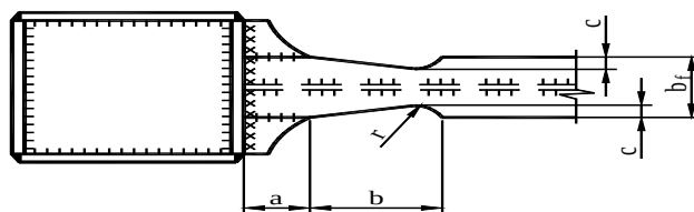
В.17-сурет – RBS аймақтарында бағанның білікпен қосылған тармақтарының нұсқасы
