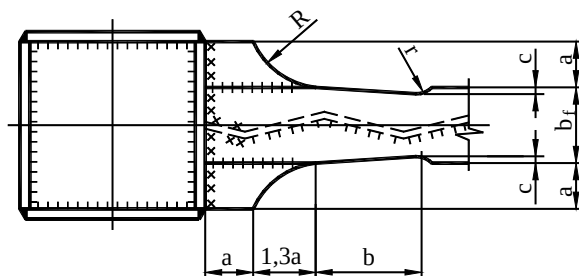
В.18 сурет –Қазақстанда қолданылатын тең кедергі аймақтары бар бағандармен біріктірілген біліктердің қосылу тармақтарының нұсқасы
