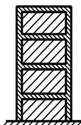
2.8 –сурет. Толтырулармен үйлестірілген моменттік жақтаулы қаңқалар
