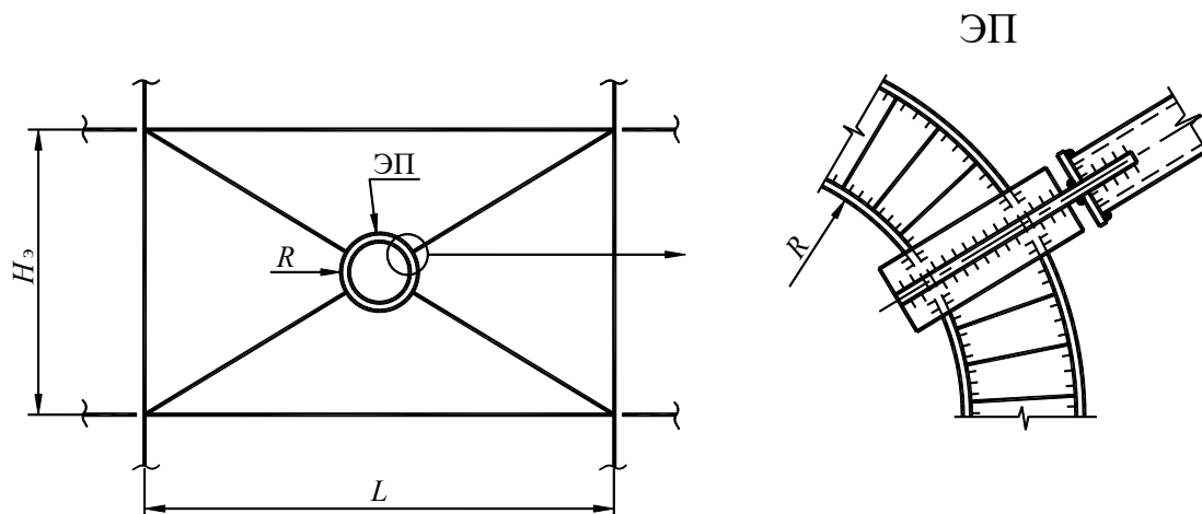
Рисунок А.24 – Крестовая связь с кольцевым энергопоглоителем
