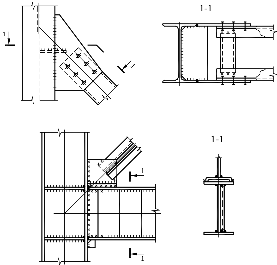
А.18 сурет –рамалы-қоспалы қаңқа торабы
