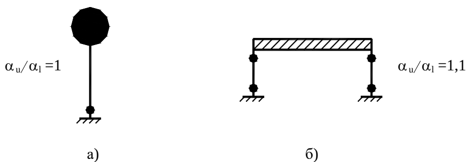
2.5 –сурет. Кері маятник: а) диссипативтік аймақтар колонна негіздемесінде; б) диссипативтік аймақтар колонналарда ( N_{Ed} / N_{pl,Rd} < 0,3 );
