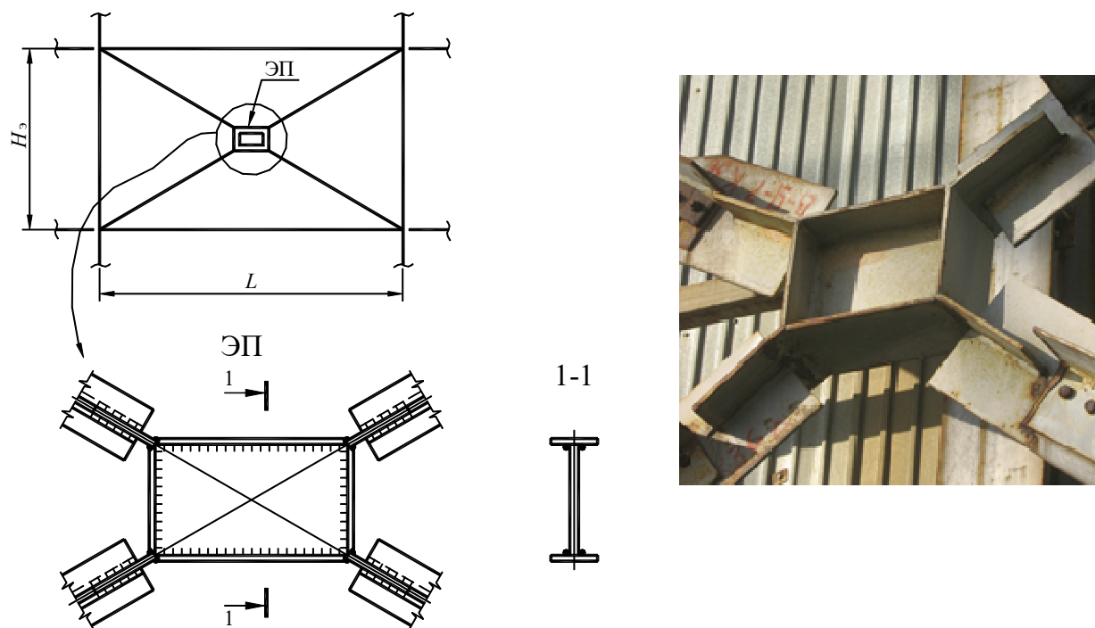
Рисунок А.23 – Крестовая связь со сдвиговым энергопоглотителем
