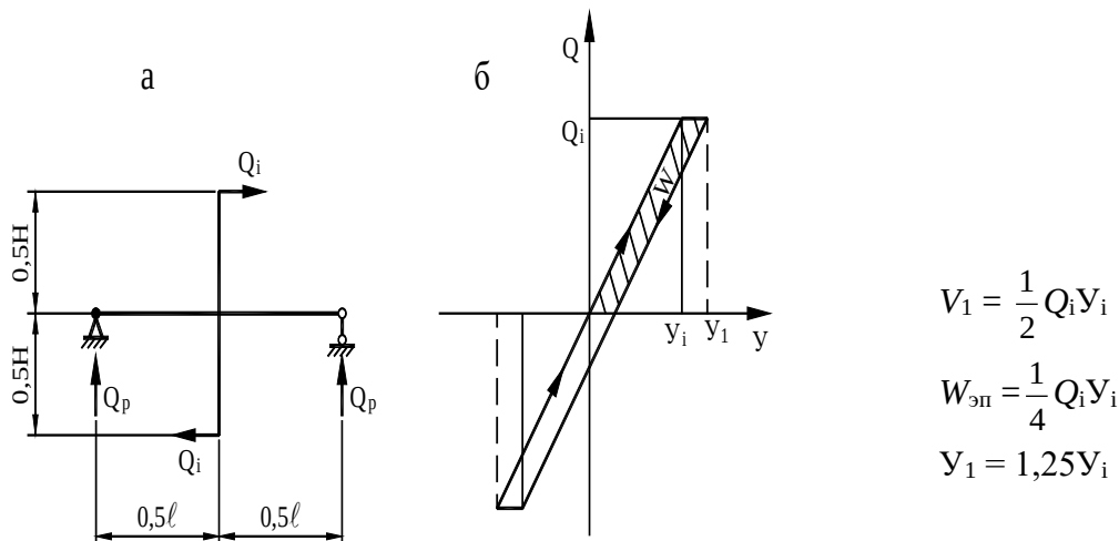
Б.2 сурет – көлденең сейсмикалық жүктемемен белгі ауысу жүктемесі кезінде (б) оның жұмысының циклограммасы мен рамалы қаңқа (а) 2-ші қабатының айшық тәрізді элементі
