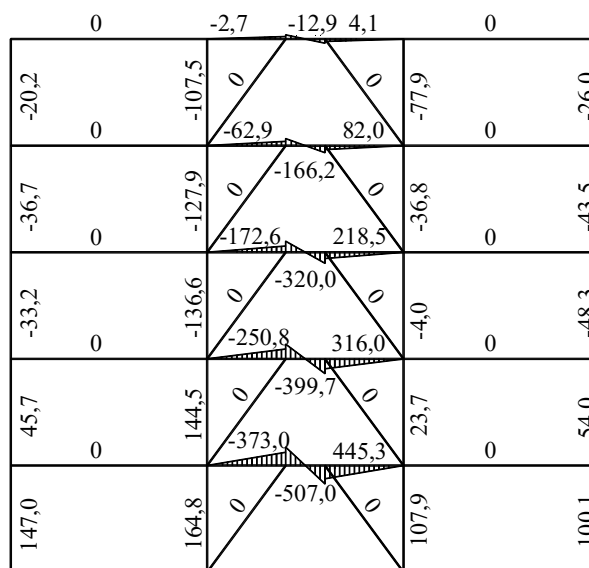
Рисунок Д.14 – Эпюра изгибающих моментов M_{Ed,E,y} от сейсмических нагрузок (ось 1)
