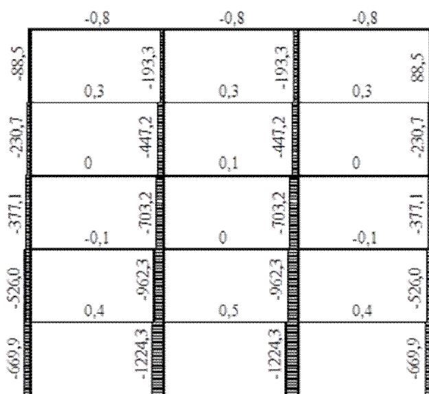
Рисунок Д.9 – Эпюры осевых сил N_{Ed,G} от гравитационных нагрузок (ряд Б)
