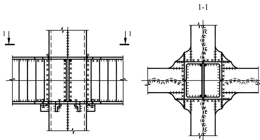
Рисунок А.9 – Сварной рамный узел каркаса с колоннами трубчатого сечения из 4-х уголков
