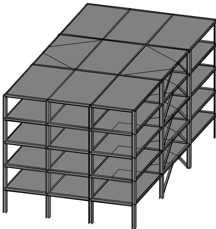
Д.2 – сурет. Ғимарат қаңқасының жалпы түрі
