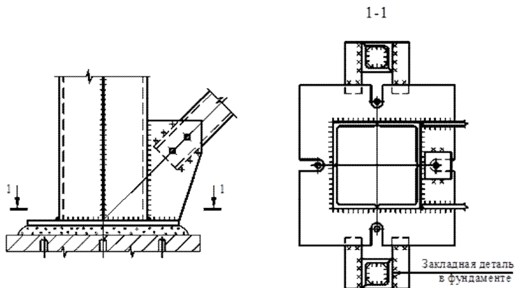
Рисунок А.22 – База колонны трубчатого сечения
