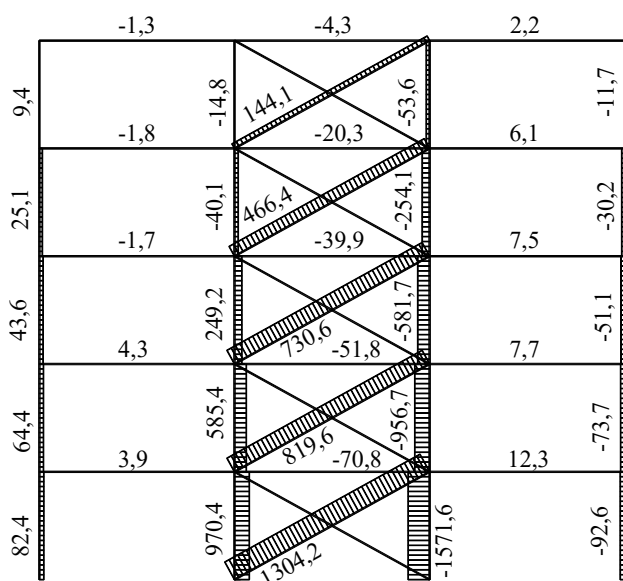
Рисунок Г.10 – Эпюры осевых сил N_{Ed,E} от сейсмических нагрузок
