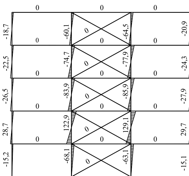
Рисунок Г.11 – Эпюры изгибающих моментов M_{Ed,E,y} от сейсмических нагрузок
