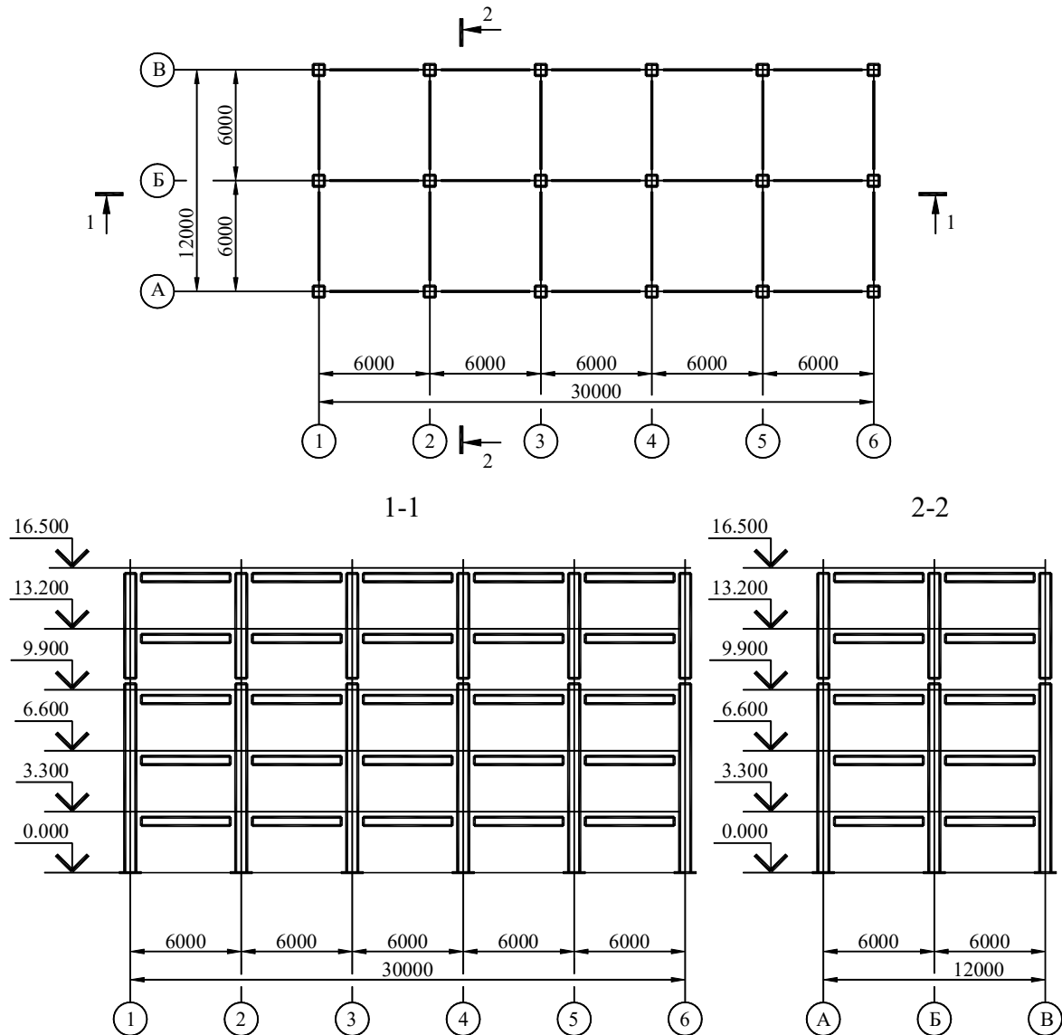
Рисунок В.1 – Схематический план и разрезы каркаса здания
