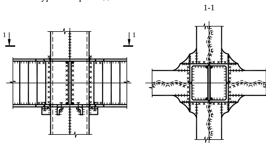
А.9 сурет – 4- бұрыштан түтікті қиылыс ұстындарымен қаңқаның дәнекерлі рамалы торабы
