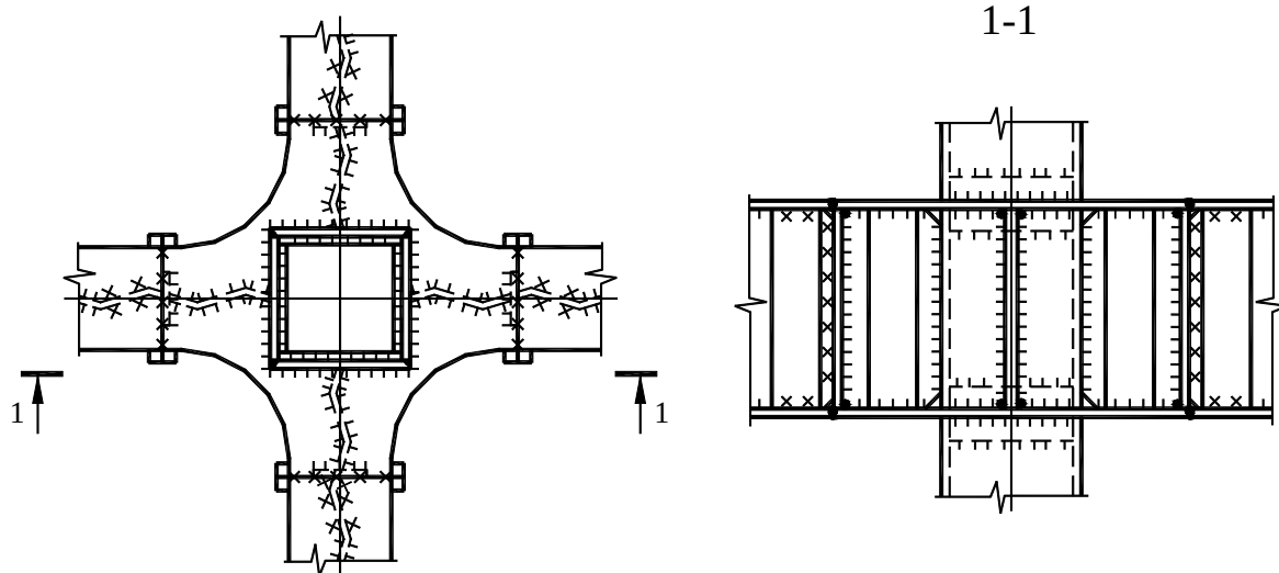
А.11 сурет – Төрт табақтан түікті қиылысты ұстындарымен қаңқаларға арналған жоғары беріктіліктің дәнекерлі рамалы торап
