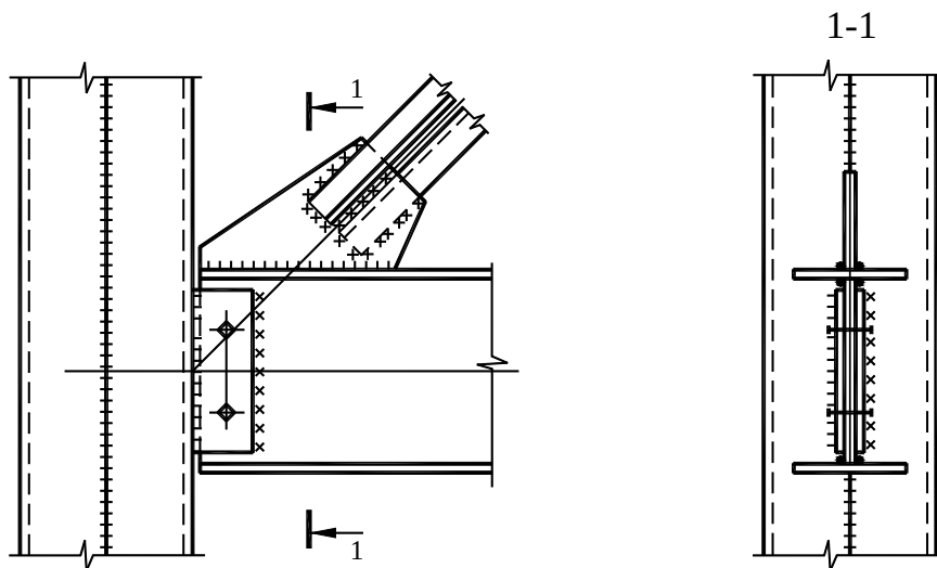
А.19 сурет – Қоспалы қаңқа торабы
