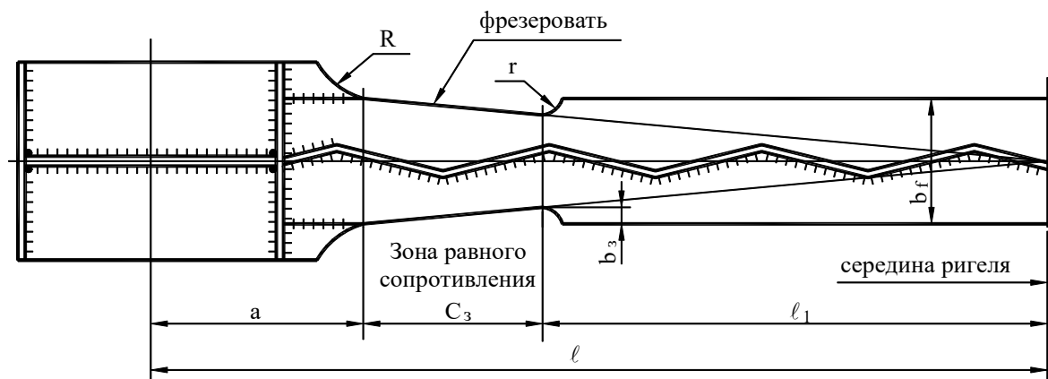
Рисунок Б.1 – Нижний пояс двутаврового ригеля с поперечно-гофрированной стенкой и зоной равного сопротивления
