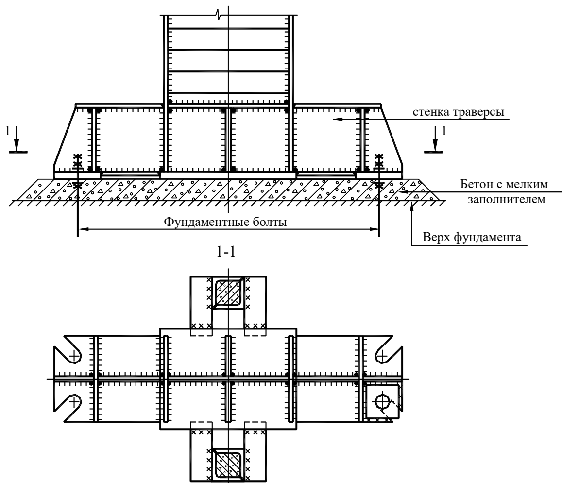
Рисунок А.13 – База колонны двутаврового сечения
