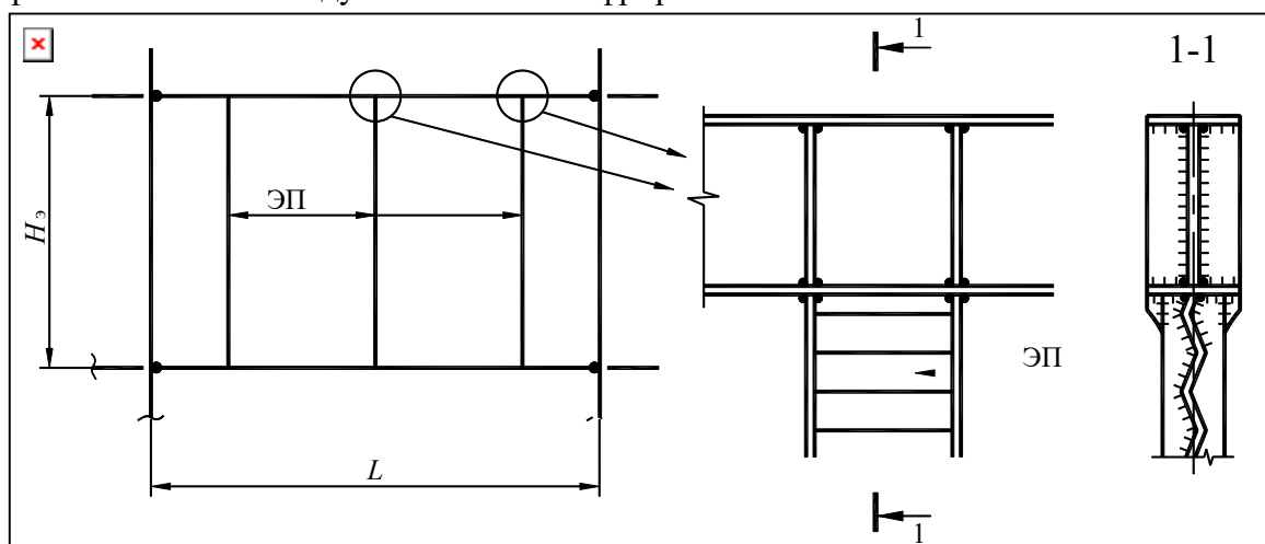
Рисунок А.28 – Связь рамного типа с балочным энергопоглопителем
