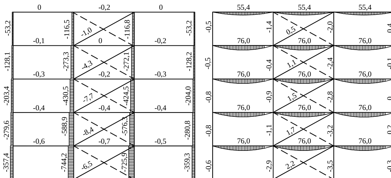
Г.8 Сурет –Гравитациялық жүктемелерден осьтік күштердің эпюрасы N_{Ed,G}
