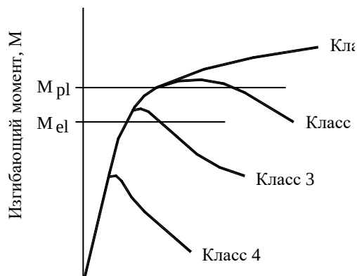
2.10 сурет – Иілу сәті мен айналу қабілеттілігі арасындағы байланыс
