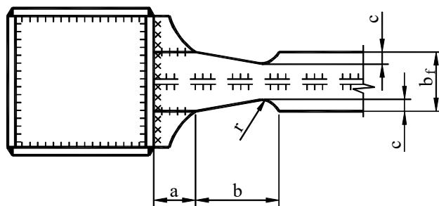
Рисунок В.17 – Вариант узла соединения балки с колонной с зонами RBS
