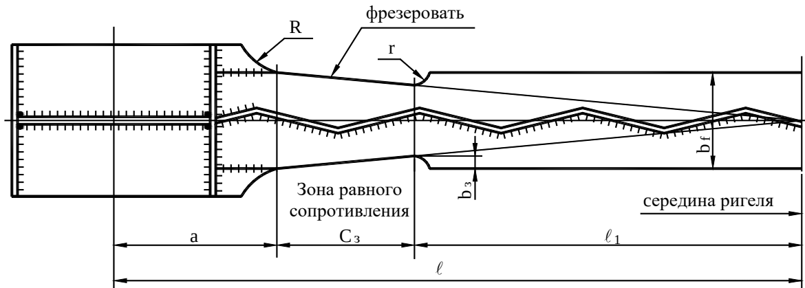
Б.1 сурет – Тең кедергі аймағы мен көлденең-гофрленген қабырғамен екі таврлы ригельдің төменгі белдеуі
