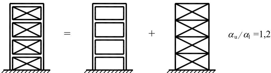
Рисунок 2.7 – Моментные рамные каркасы, комбинируемые с концентрическими связями (диссипативные зоны в моментной раме и в растянутых диагоналях). Принимаемое по умолчанию значение \alpha_u / \alpha_1 (см. 2.3.2.3 и Таблицу 2.5)
