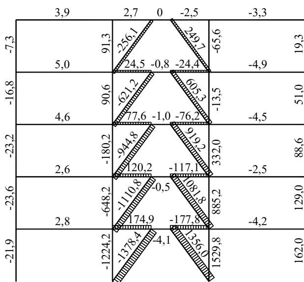
Рисунок Д.13 – Эпюра осевых сил N_{Ed,E} от сейсмических нагрузок (ось 1)
