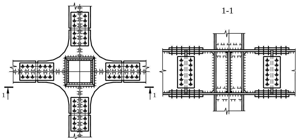
А.12 сурет – Төрт табақтан түікті қиылыс ұстындарымен қаңқаларға арналған жоғары беріктіліктің рамалы торапта ұстындармен ригельдердің бұрандалы қосылыстары
