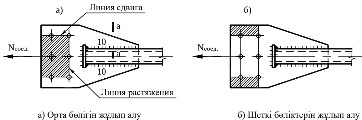
Г.16 Сурет – Байланыстың диагоналды элементінің кесінді фасонкасының материалын жұлып алу схемалары
