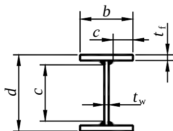
Д.18 – сурет. Бірінші қабаттың сейсмикаға қарсы буыны қимасының өлшемдері
