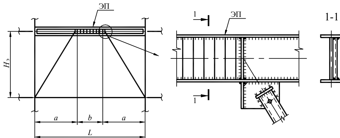
Рисунок А.27 – Полураскосная связь с балочным энергопоглопителем
