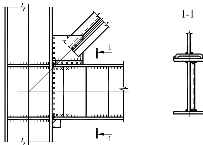
Рисунок А.18 –Узел рамно-связевого каркаса
