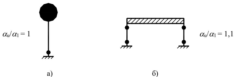
Рисунок 2.4 – Каркасы с эксцентрическими связями (диссипативные зоны в антисейсмических звеньях, работающих на изгиб и сдвиг). Принимаемое по умолчанию значение \alpha_w/\alpha_1 (см. 2.3.2.3 и Таблицу 2.5)
