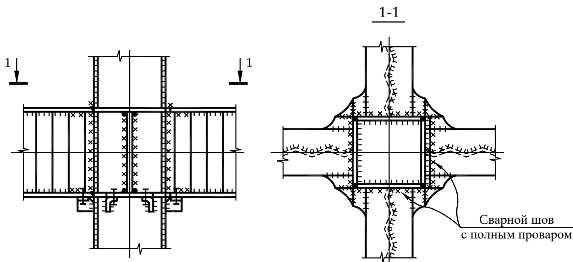
А.10 сурет – 4 табактан түтікті қиылыс ұстындарымен қаңқаның дәнекерлі рамалы торабы
