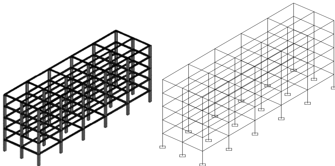
Рисунок В.3 – Конструктивная и расчетная схемы здания
