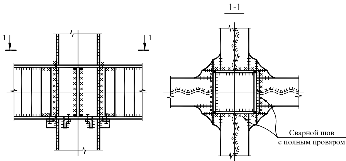
Рисунок А.10 – Сварной рамный узел каркаса с колоннами трубчатого сечения из 4-х листов
