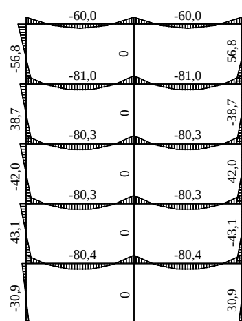
В.9-сурет – сейсмикалық емес M_{Ed,G} кезеңдердің мәні
