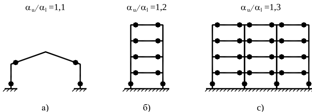
2.1-сурет. Моменттік жақтаулы қанқалар (арқалықтардағы және колонналардың төменгі бөлігіндегі диссипативтік аймақтар).
