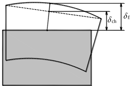
Рисунок 2.10 – К классификации перекрытий по жесткости в соответствии с условием (2.2)
