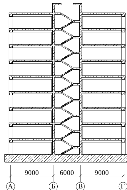
РАЗРЕЗ 1-1
