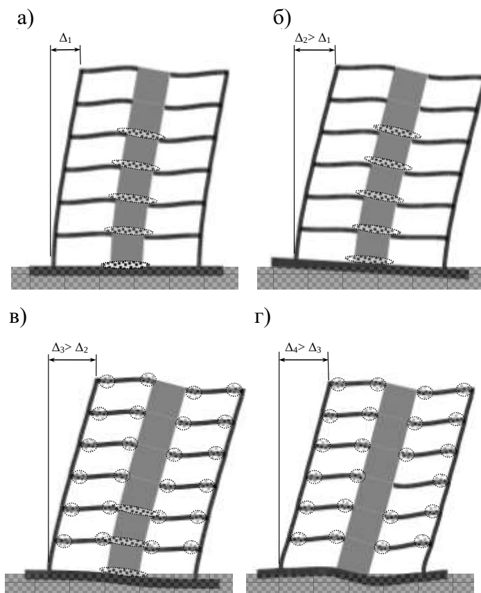
6.1-сурет – Қаңқалы конструктивтік жүйенің көлденең жүктемелеріндегі деформациялану схемалары: а) қатты негізде қысылған іргетас тақтасымен; б) иілгіш негізде жазықтықтан қатты іргетас тақтасымен; в) иілгіш негізде жазықтықтан иілгіш іргетас тақтасымен; г) иілгіш негізде жазықтықтан икемді іргетас тақтасымен
