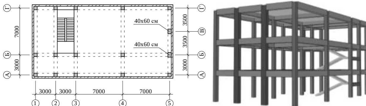
Рисунок Г.4 – Схематический план и общий вид каркаса
