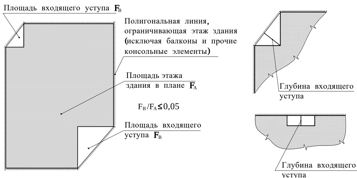
3.4-сурет – Ғимарат конфигурацияларын жіктеуге
