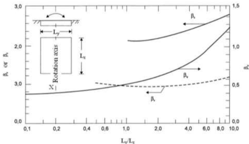
Е.2 суреті – \beta_x , \beta_z және \beta_{\psi} коэффициенттерінің мәндерін анықтауға (исправить рисунок)
