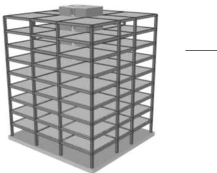
Рисунок Г.7 – Общий вид и расчетная схема конструктивной системы здания
