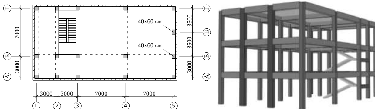
Г.4 суреті – Схемалық жоспар және қаңқаның жалпы көрінісі
