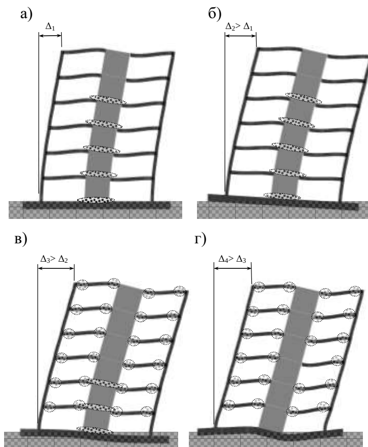
Рисунок 6.1 – Схемы деформирования при горизонтальных нагрузках каркасной конструктивной системы: а) с фундаментной плитой, защемленной в жестком основании; б) с жесткой из плоскости фундаментной плитой на податливом основании; в) с податливой из плоскости фундаментной плитой на податливом основании; г) с гибкой из плоскости фундаментной на податливом основании
