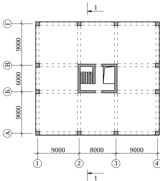
Г.6 суреті – Ғимараттың схемалық жоспары және қимасы
