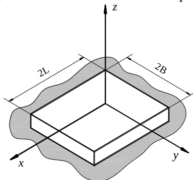
Рисунок Е.1 – Схема расположения осей фундаментной плиты
