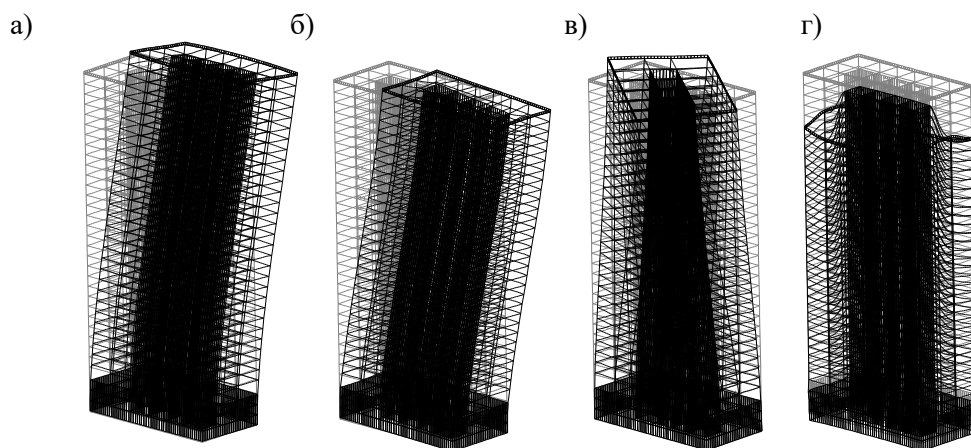
3.1-сурет – Жүйелі конструктивтік жүйенің тербелістерінің негізгі нысандары:
