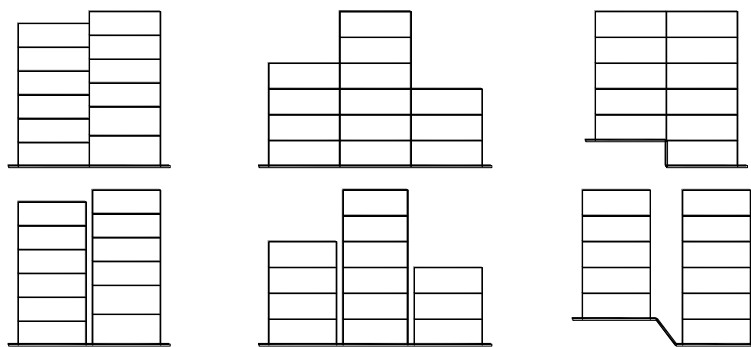
2.5-сурет – Күрделі конфигурациялары бар ғимараттарды биіктігі бойынша динамикалық тәуелсіз бөліктерге бөлу мысалдары
