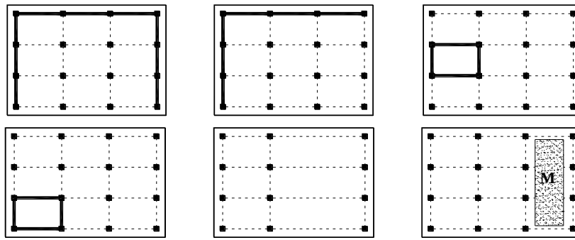
2.8-сурет – Қаттылықтардың және/немесе массалардың (М) жоспардағы теңгерімсіз бөлінуімен конструктивтік схемалардың мысалдары
