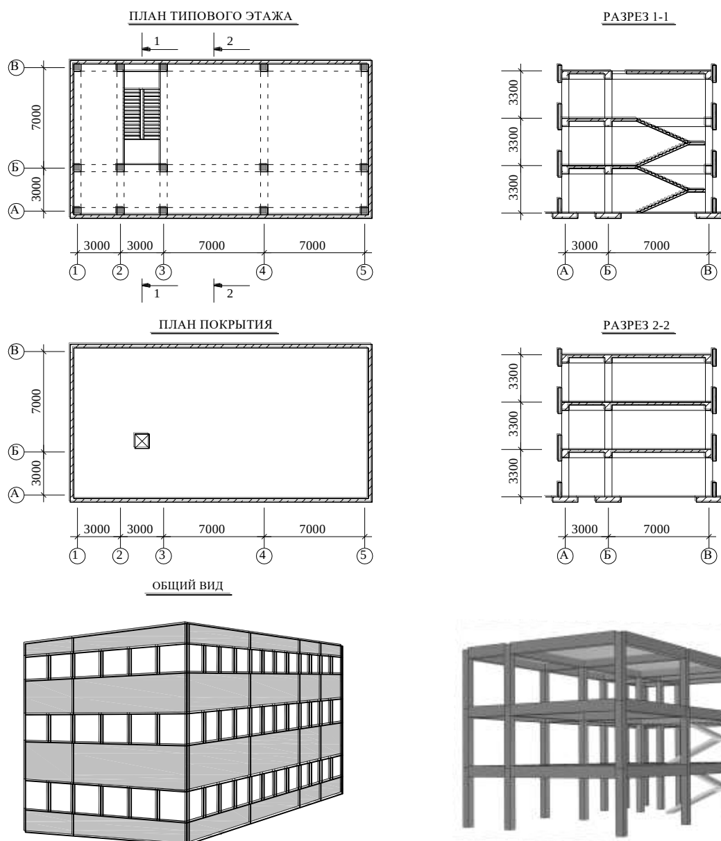
Г.1 суреті – Схемалық жоспар, қималар және ғимарат пен қаңқаның жалпы түрлері.
