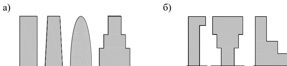
2.2-сурет – Ғимараттың биіктігі бойынша конфигурациясы: а) қолайлы және б) қолайлы емес
