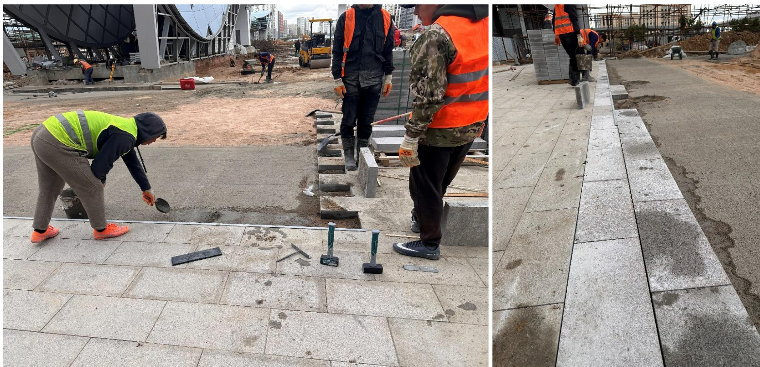
4-сурет – Гранитті плиталарды төсеу
