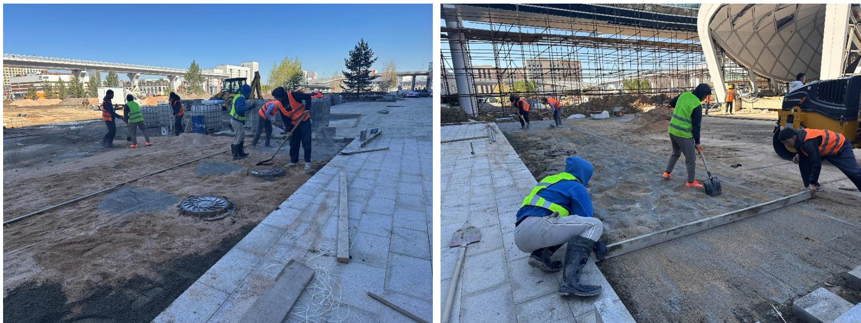
3-сурет – Цемент-құм қоспасынан тегістеу қабатын орнату
