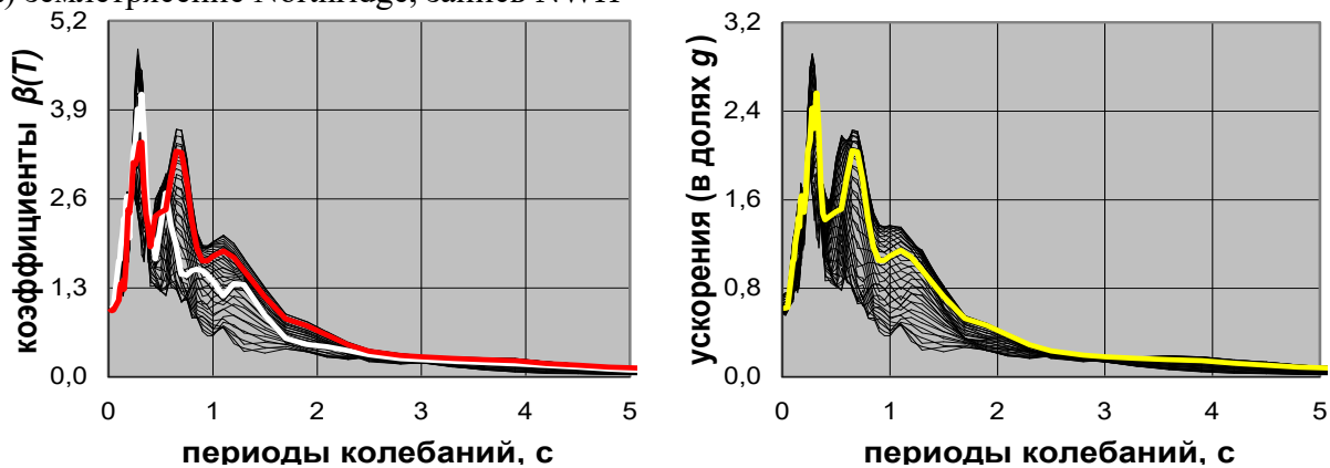
Рис. 3.2.16. Сопоставление семейств графиков \beta(T) с парами индивидуальных графиков \beta(T) , построенных по инструментальным записям на ортогональных направлениях, и семейств спектров реакции с огибающими пар индивидуальных спектров
