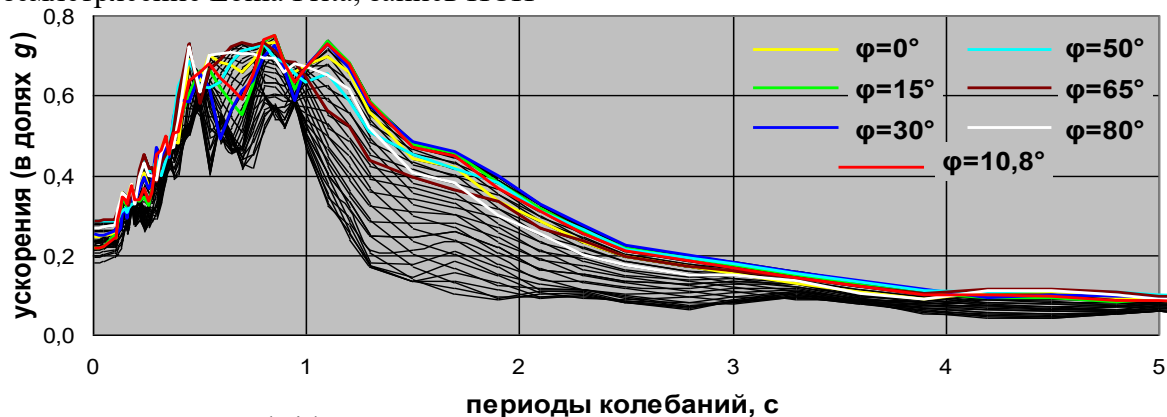
в) землетрясение Northridge, запись SCS
