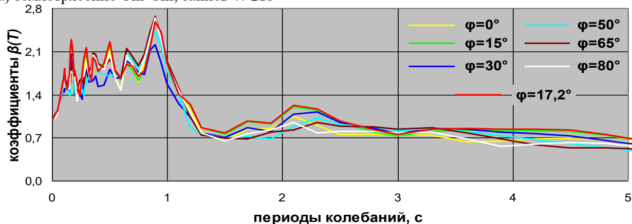
б) землетрясение Loma Prieta, запись HCH
