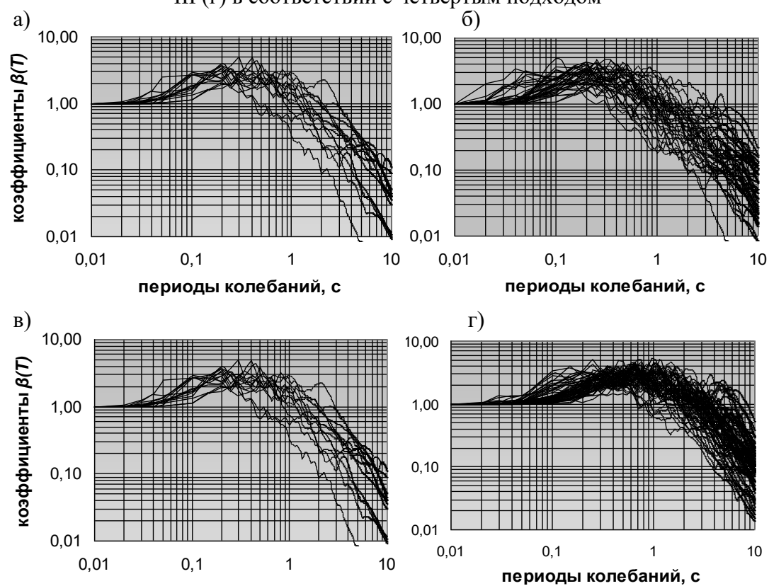
Рис. 3.2.5. Выборки, сформированные для грунтов категорий IA (а), IB (б), II (в) и III (г) в соответствии с пятым подходом
