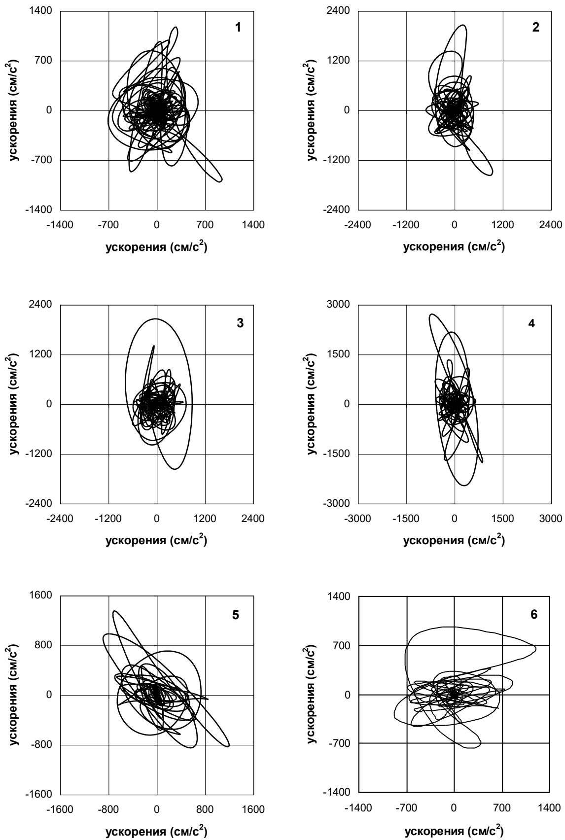
Рис. 8.1. Траектории ускорений, отвечающие воздействиям, зарегистрированным при землетрясении Loma Prieta (ст. Sylmar).
