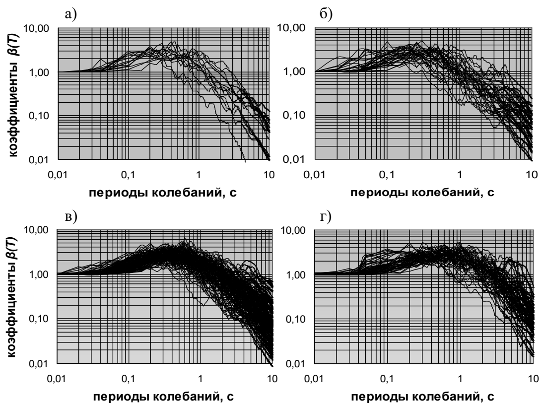
Рис. 3.2.4. Выборки, сформированные для грунтов категорий IA (а), IB (б), II (в) и III (г) в соответствии с четвертым подходом
