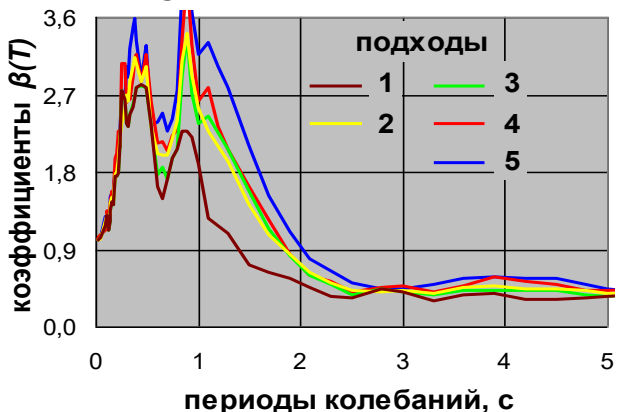
Рис. 3.2.18. Кривые \beta(T) , характеризующие динамические эффекты восьми сейсмических процессов в соответствии с подходами 1-5
