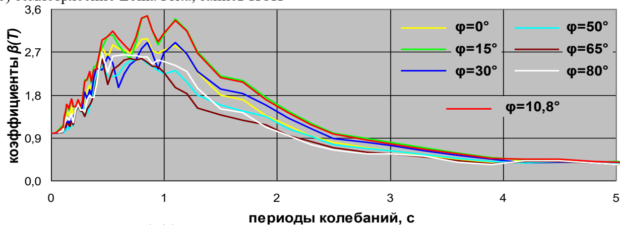
в) землетрясение Northridge, запись SCS
