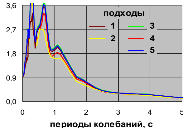
Рис. 3.2.18. Кривые \beta(T) , характеризующие динамические эффекты восьми сейсмических процессов в соответствии с подходами 1-5
