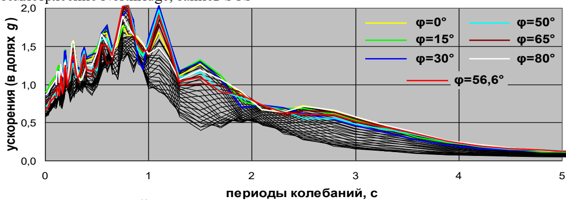
г) землетрясение Косаели, запись ATS
