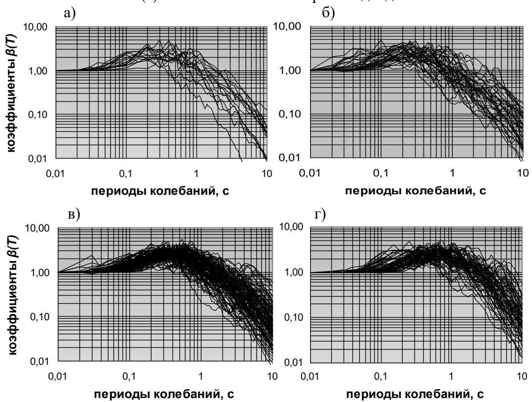
Рис. 3.2.3. Выборки, сформированные для грунтов категорий IA (а), IB (б), II (в) и III (г) в соответствии с третьим подходом
