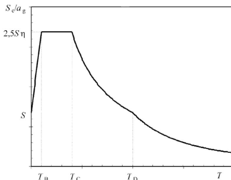
Рис. 2.1. Спектр упругой реакции для горизонтальных сейсмических воздействий
