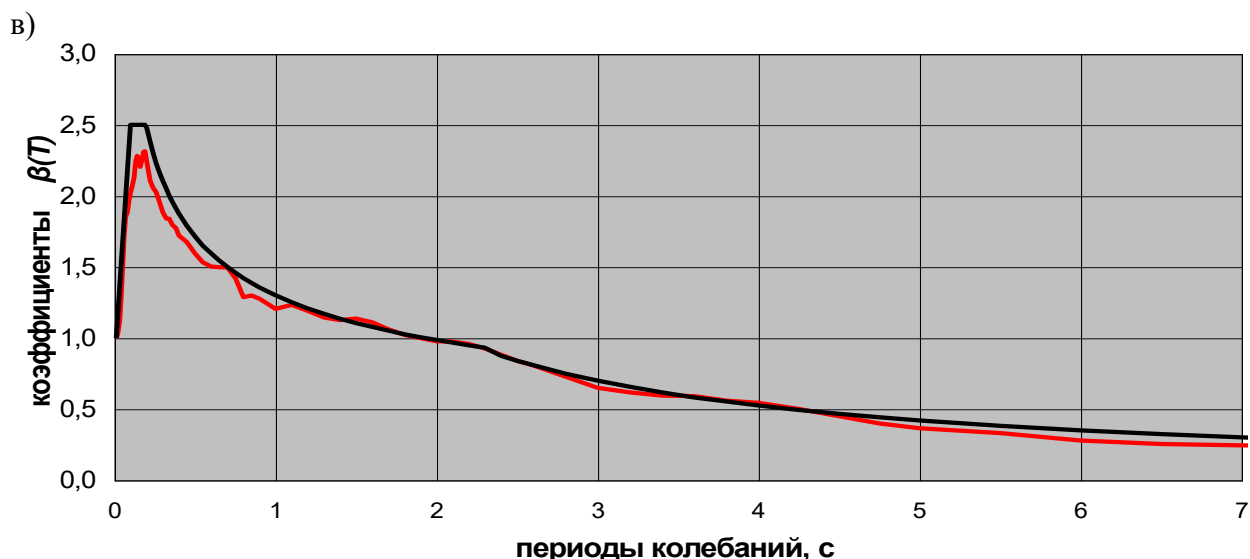
Рис. 3.4.2. «Средние» огибающие (красные линии) и аппроксимирующие их кривые, построенные по записям на грунтах категорий I (а), II (в) и III (г)
