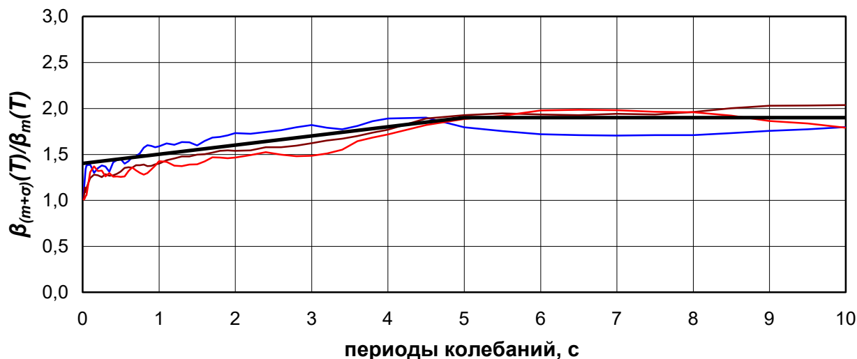
Рис. 5.2. Графики \beta_{(m+k\sigma)}/\beta_m , построенные для грунтов категорий I (синяя линия), II (коричневая линия) и III (красная линия) при значении k=1,0 и аппроксимирующий их график (черная линия)
