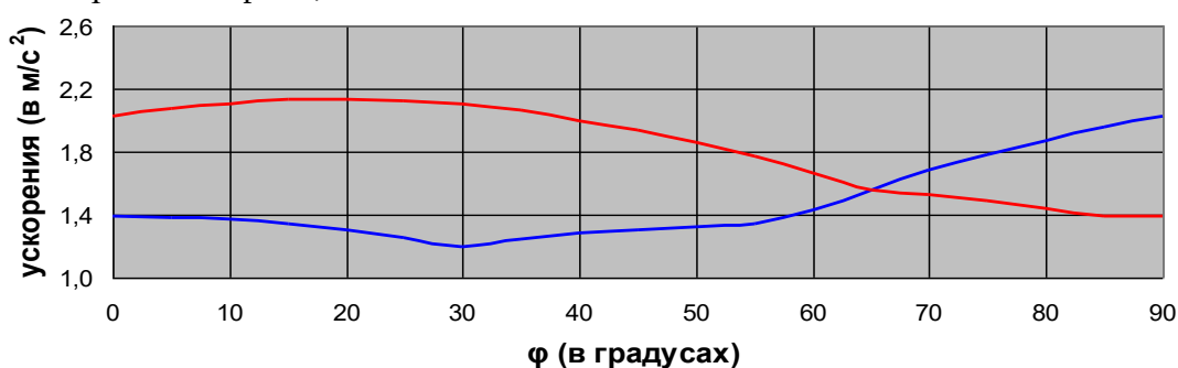
Рис. 3.2.11. Величины максимальных ускорений сейсмических процессов на разных азимутальных направлениях
