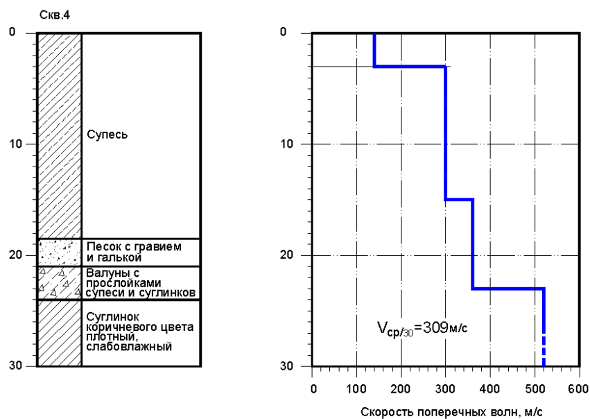
Рис. 1.9. Скорость распространения поперечных волн в 30-метровой поверхностной толще грунтов вблизи площадки ТЭЦ-2
