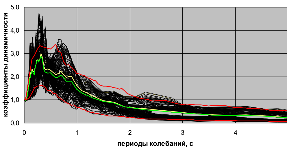
Рис. 3.2.9. Группа «семейств» графиков \beta(T) , построенных по записям на грунтах категории II землетрясений Kobe (запись KJM), Landers (запись ABY), Northridge (запись NWH) и Hector Mine (запись 2108), и «средние» графики \beta(T) , вычисленные для группы индивидуальных графиков \beta(T) , построенных по инструментальным записям этих же землетрясений
