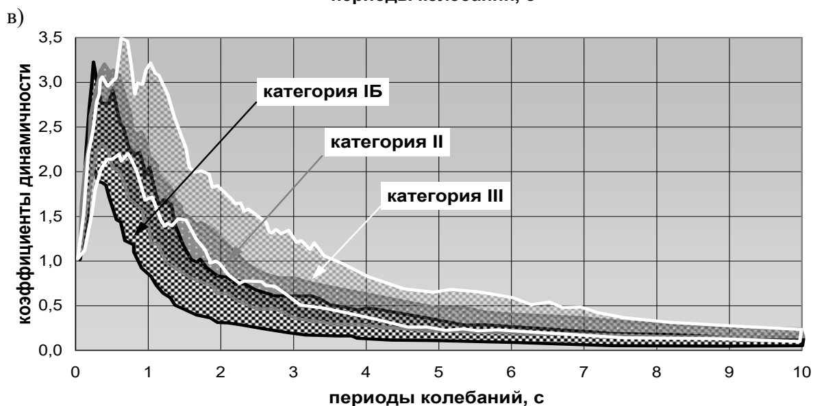
Рис. 3.2.6. Сопоставление областей, в пределах которых сформированные выборки содержат 50% данных
