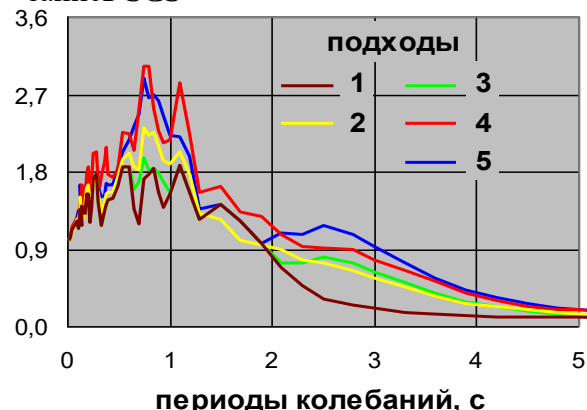
г) землетрясение Kobe, запись TAK
