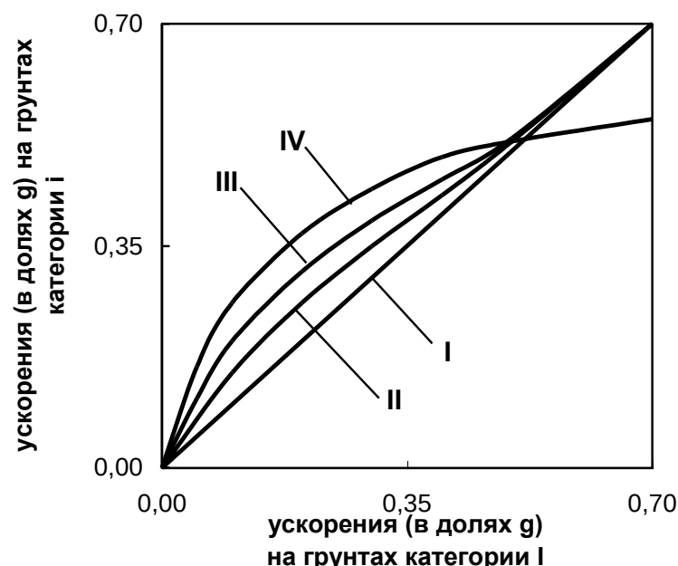
Рис. 7.2. Схема влияния деградации жесткости и прочности грунтов на величины пиковых ускорений по /6/
