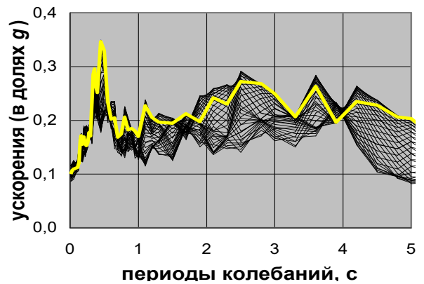
Рис. 3.2.15. Сопоставление кривых, огибающих пары индивидуальных спектров, построенных для ортогональных направлений
