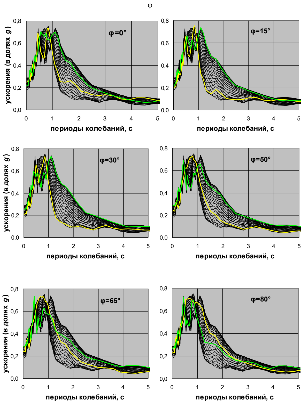
Рис. 3.2.12. «Семейство» спектров реакции, построенное по записям землетрясения Chi-Chi, и пары индивидуальных спектров реакции, полученные с помощью акселерограмм, вычисленных для ортогональных направлений при разных значениях \varphi
