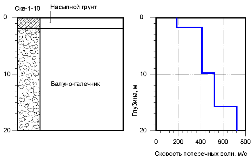
Рис. 1.8. Скорость распространения поперечных волн в 30-метровой поверхностной толще грунтов площадки №9
