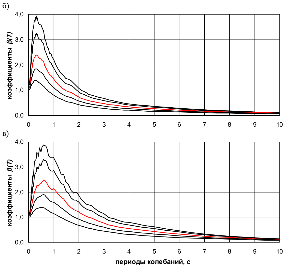
Рис. 4.1. Обобщенные графики \beta(T) , построенные при значениях коэффициента вязкого демпфирования 1%, 2%, 5%, 10% и 20% на основании подхода 2 по инструментальным записям, зарегистрированным на грунтах категорий I (а), II (б) и III (в).
