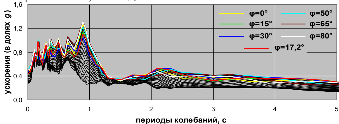
б) землетрясение Loma Prita, запись HCH
