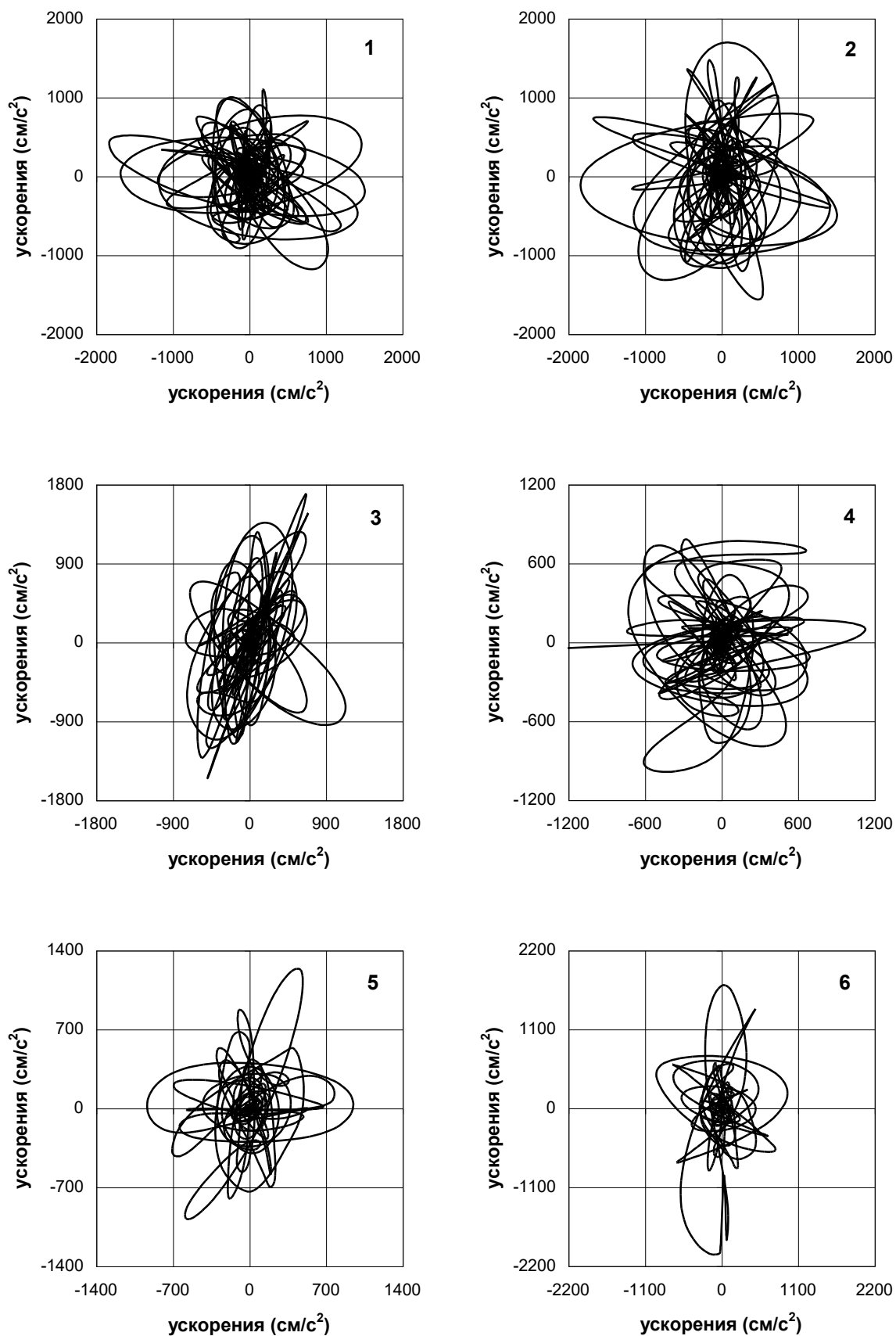
Рис. 8.2. Траектории ускорений, отвечающие воздействиям, зарегистрированным при землетрясении Loma Prieta (ст. Newhall)
