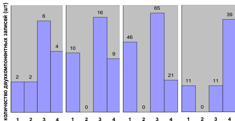
Рис. 3.1.4. Данные о количестве двухкомпонентных записей, зарегистрированных на грунтах категорий IA (а), IB (б), II (в) и III (г) при землетрясениях с разными механизмами очагов
