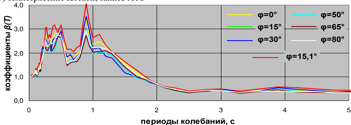
г) землетрясение Kocaeli, запись ATS
