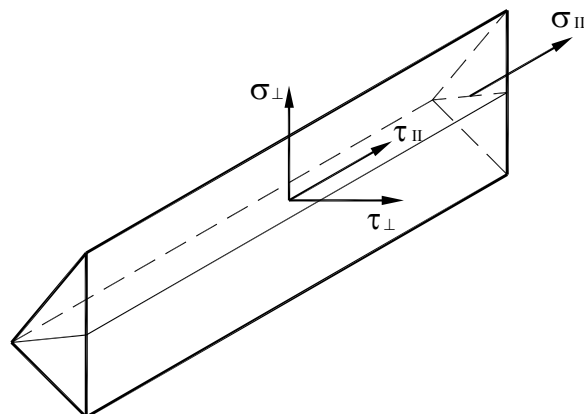
Рисунок 6.20 – Напряжения в поперечном сечении углового сварного шва
