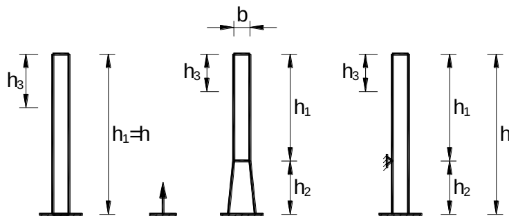
2.9 Сурет. Түгін мұржаларына арналған өлшемдер
