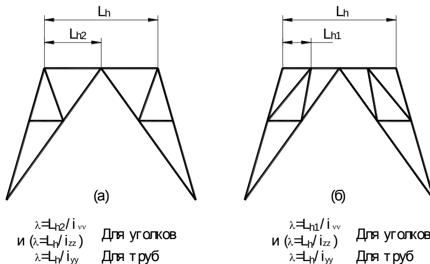
Рисунок 6.10 – Горизонтальные элементы К-образных расколов без диафрагм
