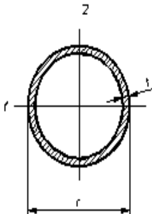
А.5 Сурет. Дөңгелек құбыр қиылысының мөлшерлері
