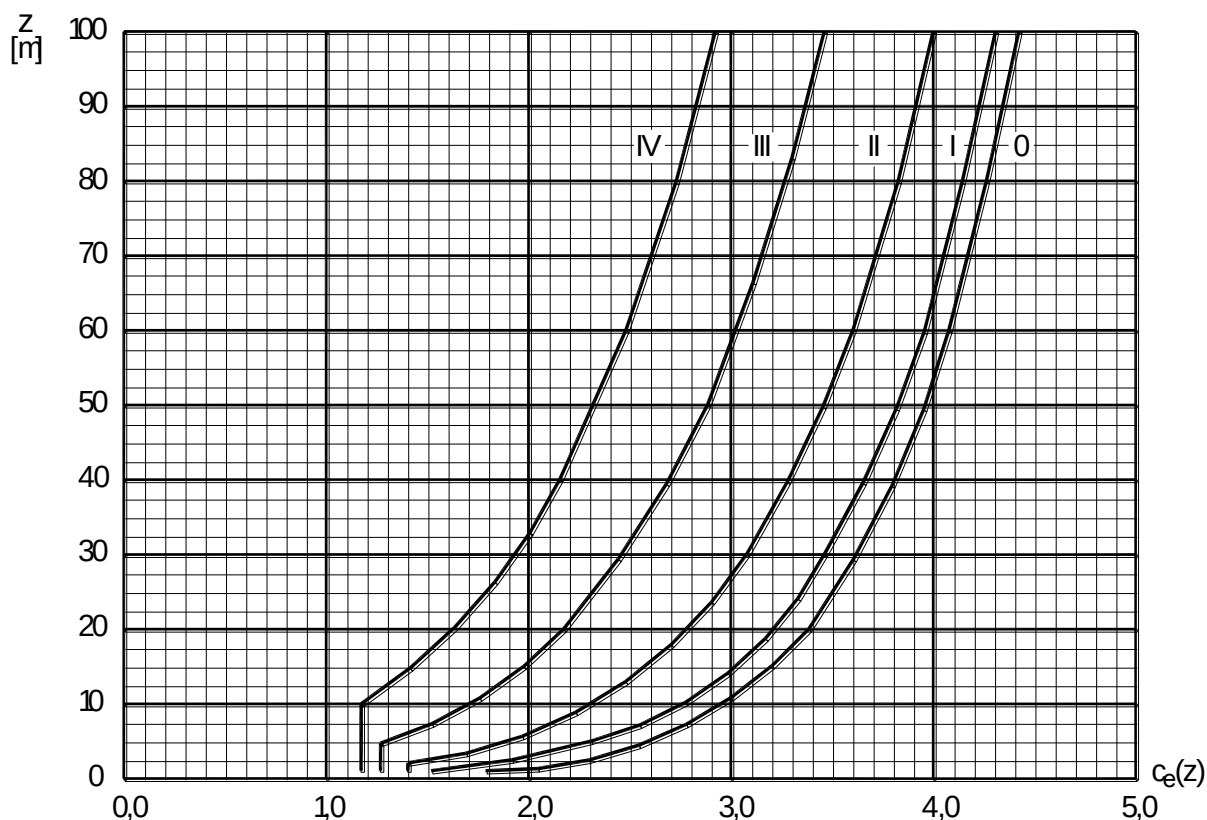
Рисунок 2.6 – Графическое представление коэффициента экспозиции c_e(z) для c_0 = 1,0 , k_i = 1,0
