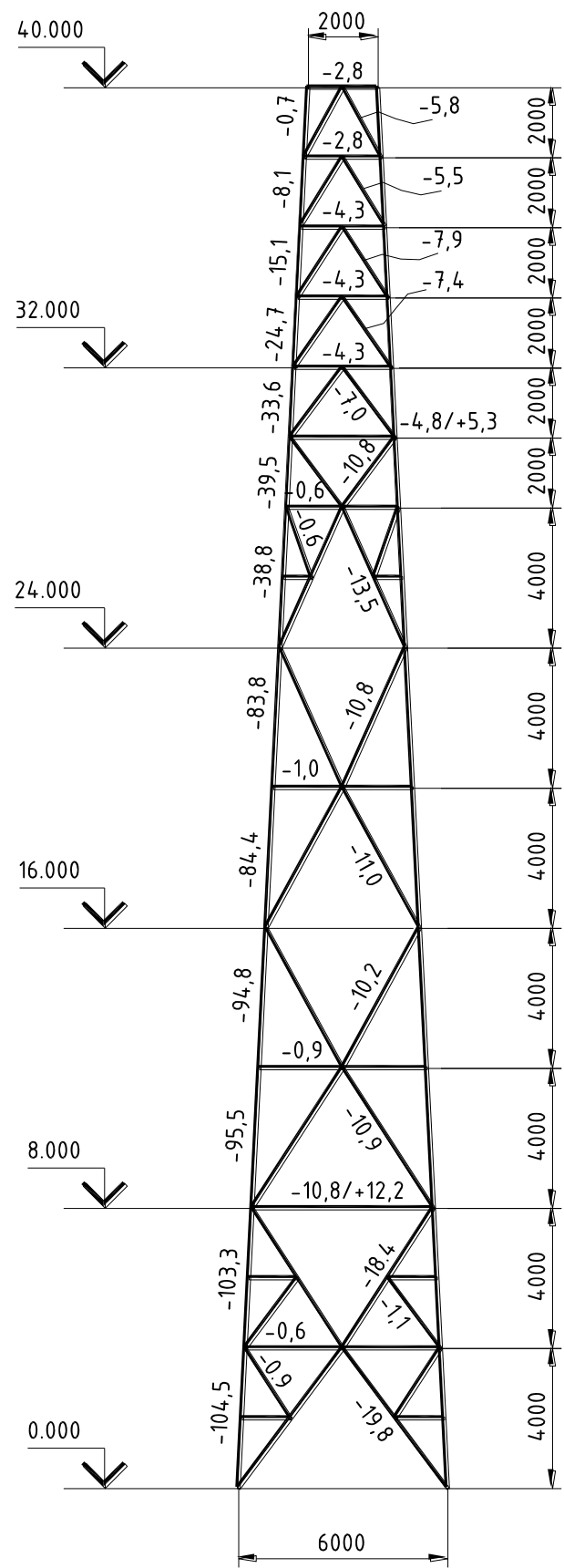
Рисунок А.8 – Схема максимальных усилий в элементах башни (в тс)
