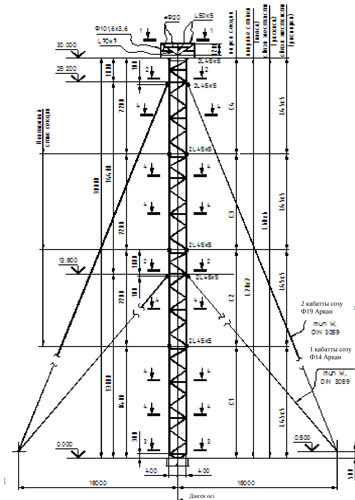
Б.1 Сурет – Баған элементтерінің және биіктігі 30,0 м діңгек тартылымы сызбасы
