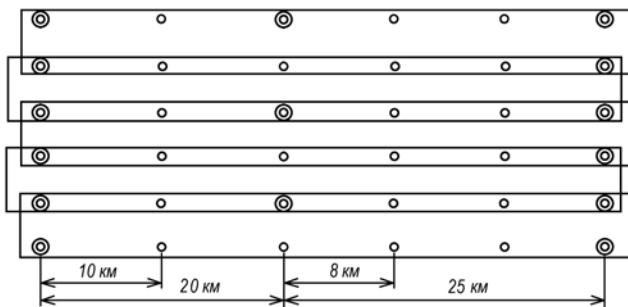
Рис. 6. Съемка в масштабе 1:25 000 с сечением рельефа через 2,5 м
