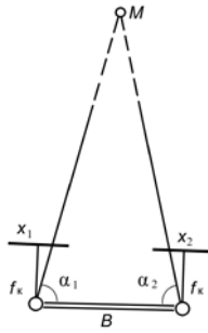
Рис. 38. Схема измерения контрольных направлений
