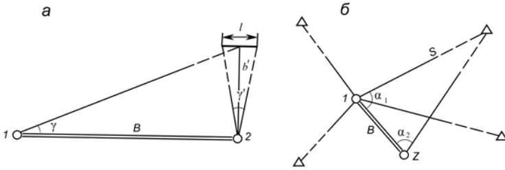
Рис. 37. Схемы определения длины базиса фотографирования: а) с помощью вспомогательного базиса; б) из неполного треугольника
