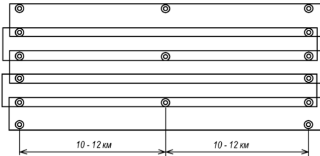
Рис. 5. Съёмка в масштабе 1:10 000 с сечением рельефа через 5,0 м
