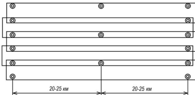
Рис. 8. Съемка в масштабе 1:25 000 с сечением рельефа через 10,0 м
