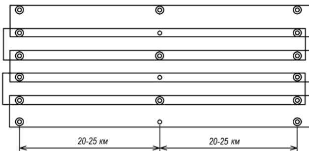
Рис. 7. Съемка в масштабе 1:25 000 с сечением рельефа через 5,0 м
