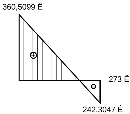
10.18 сурет — Ұстық су аккумулятор багының IV белдеуінің желілік температура ауысуының эпюрасы (360,51 K; 273 K; 242,3045 K)
