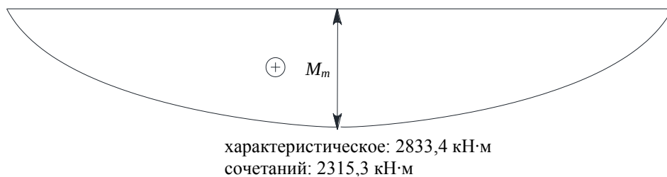
Рисунок 9.31 — Изгибающий момент вследствие приложения характеристического значения транспортных нагрузок (тротуар) (к примеру 9)
