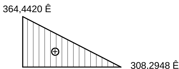
10.25 сурет — Ыстық су аккумулятор багыныңVIжәнеVIII белдеулерінің желілік температура ауысуының эпюрасы (364,4420 К; 308,2948 К)
