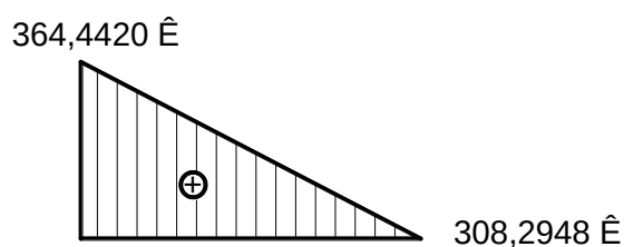
Рисунок 10.24 — Эпюра линейного температурного перепада для V пояса бака-аккумулятора горячей воды (364,4420 К; 308,2948 К)
