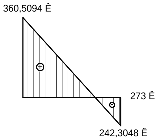
10.20 сурет—Ұстық су аккумулятор багының VI және VII белдеулерінің желілік температура ауысуының эпюрасы
