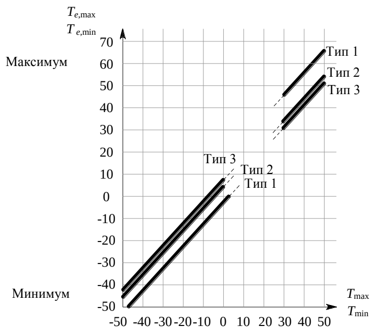
Рисунок 9.4 [6.1] — Корреляция между минимальной/ максимальной температурой наружного воздуха ( T_{\min}/T_{\max} ) и минимальной/максимальной составляющей равномерно распределенной температуры для мостов ( T_{e,\min}/T_{e,\max} )
