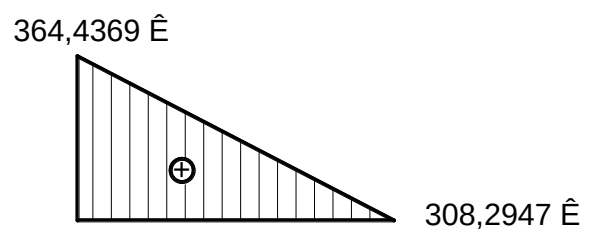
10.20 сурет—Ұстық су аккумулятор багының VI және VII белдеулерінің желілік температура ауысуының эпюрасы
