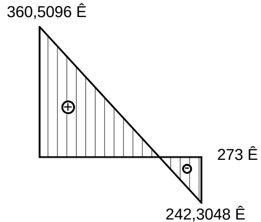
10.19 сурет- Ұстық су аккумулятор багының V белдеуінің желілік температура ауысуының эпюрасы (360,5102 K; 273 K; 242,3045 K)
