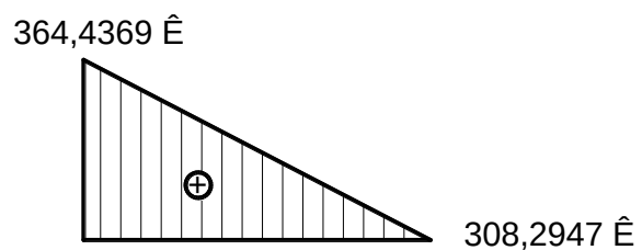
Рисунок 10.22 — Эпюра линейного температурного перепада для III пояса бака-аккумулятора горячей воды (364,4369; 308,2947 К)
