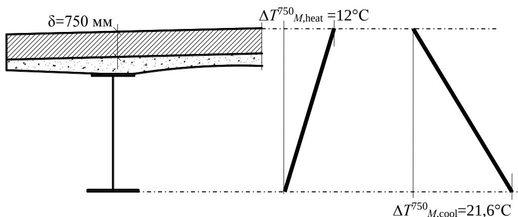
Рисунок 9.12 – Линейный температурный перепад проектируемого моста по пролетному строению с засыпным покрытием толщиной 750 мм (к примеру 6)
