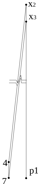
Рисунок 14.29 – Схема определения углового коэффициента облученности от прямоугольника 4-7-X_3-X_2 стороны пламени E-F
