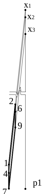
Рисунок 14.27 – Схема определения углового коэффициента облученности для стороны A-B от прямоугольника 1-7-9-2 стороны пламени E-F
