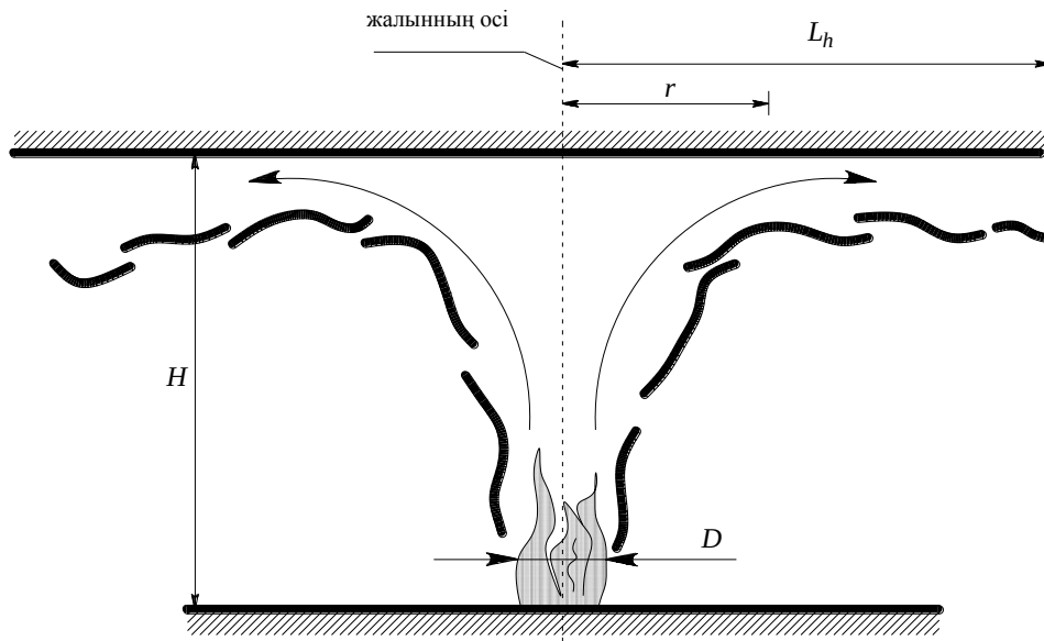
10.2-сурет – Локалдык өрт ( L_f \geq H )
