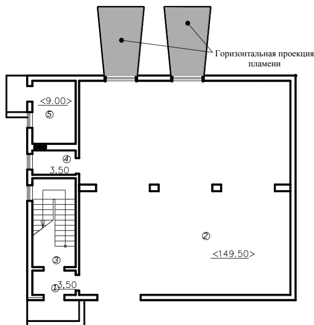
Рисунок 14.25 – Горизонтальная проекция фронта пламени из проемов производственного помещения (поз.2 план на отм. 0.000)
