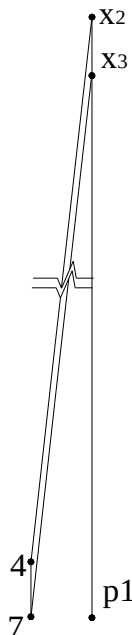
14.29-сурет – Жалынның E-F жағының 4-7- X_3 - X_2 тік бұрышынан сәулелендірудің бұрыштық коэффициентін анықтаудың схемасы
