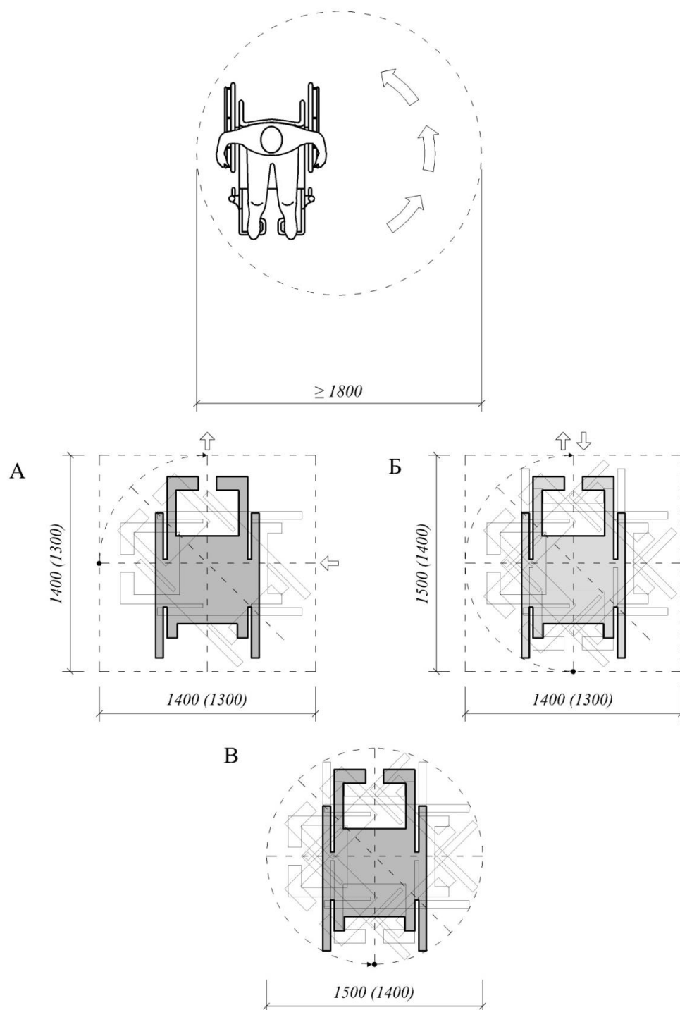
Рисунок В.1 - Габариты занимаемой зоны при вращении кресла-коляски
