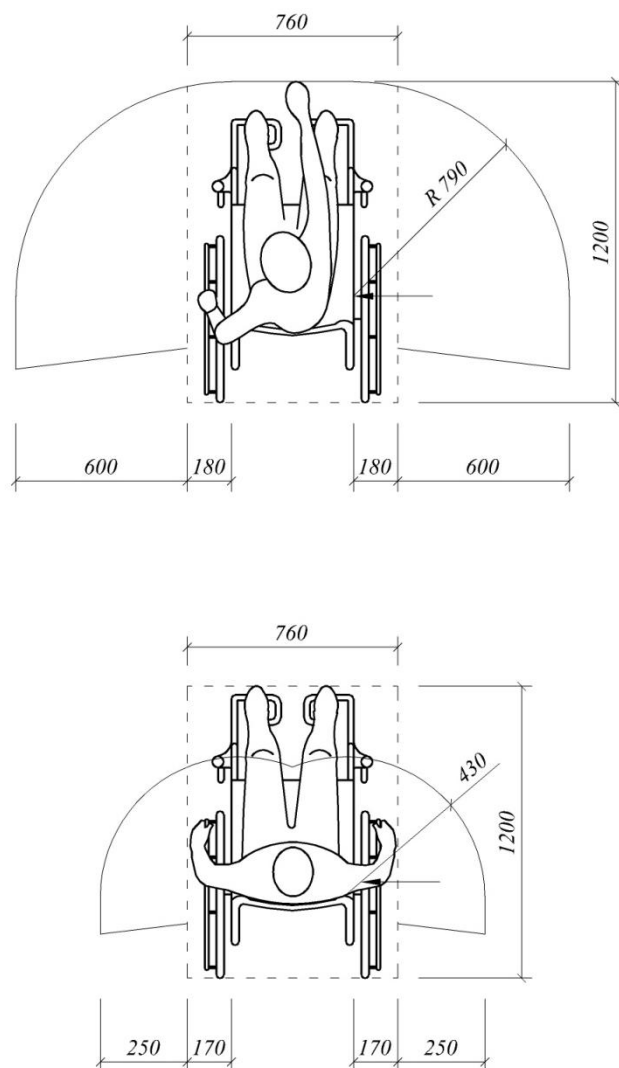
Рисунок Б.2 – Радиус доступности для людей на креслах-колясках
