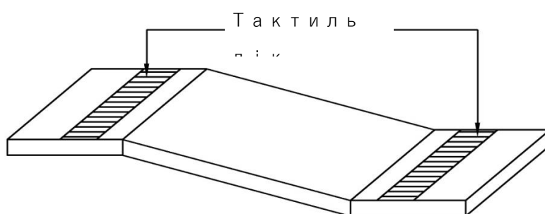
И.2-сурет. Пандустардағы ескертпе жолақтардың орналасуы
