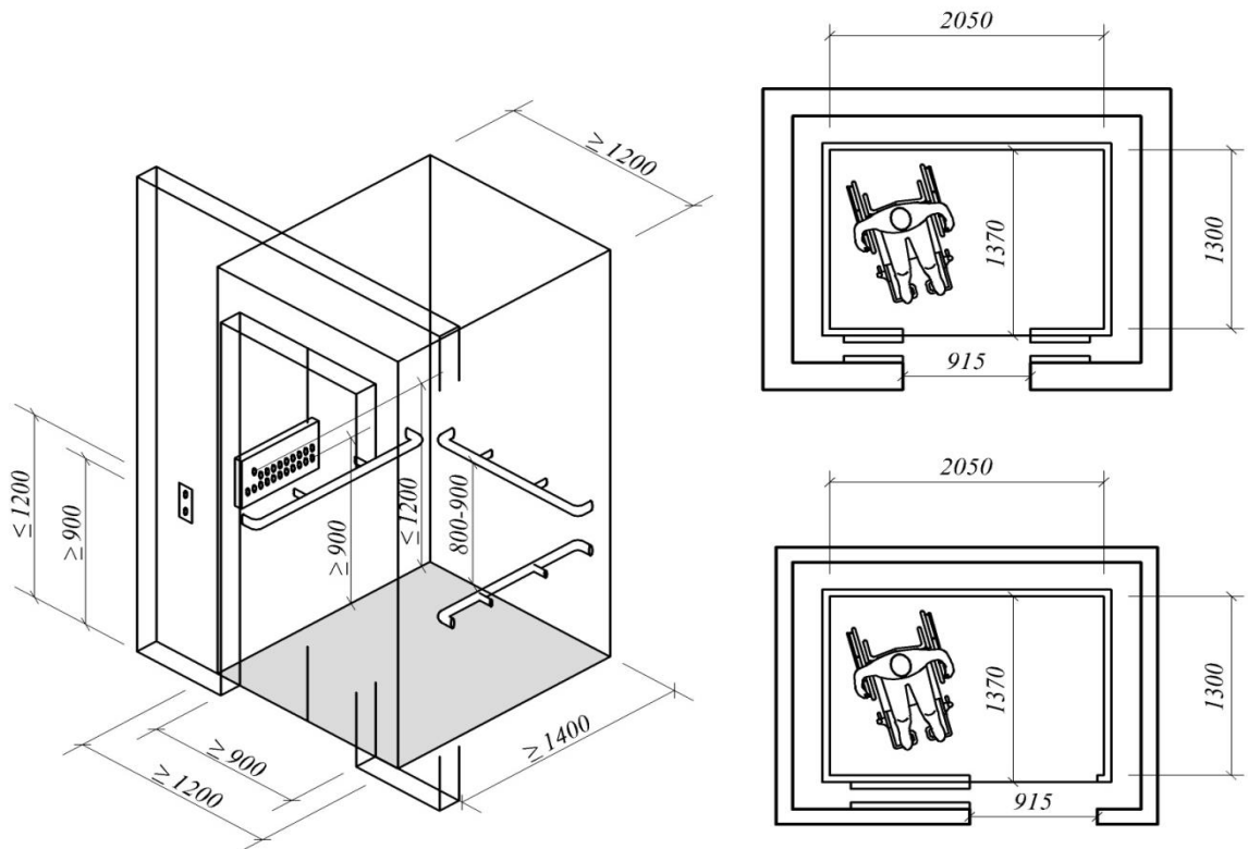
Л.1-сурет. Лифтінің ең төменгі габариті
