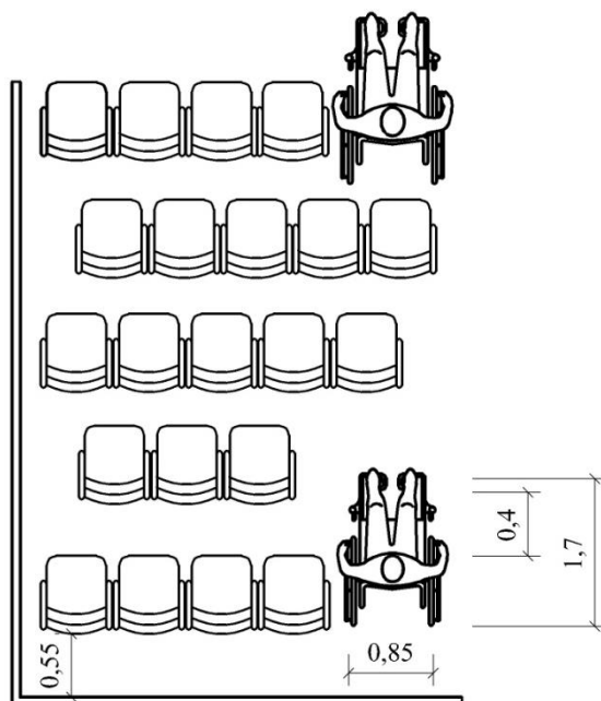
Рисунок Н.6 - Места в зрительных залах для лиц с инвалидностью на креслах-колясках
