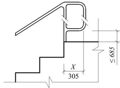
И.3-сурет. Баспалдақ тұтқаларының орналасуы
