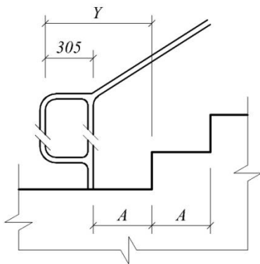
И.3-сурет. Баспалдақ тұтқаларының орналасуы
