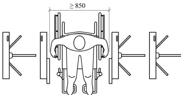
Н.1-сурет. Турникет арқылы кресло-арбамен қозғалатын мүгедектігі бар адамдарға арналған өту жолы
