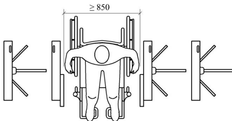
Рисунок Н.1 - Проезд для лиц с инвалидностью на креслах-колясках через турникет
