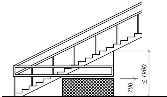
И.3-сурет. Баспалдақ тұтқаларының орналасуы
