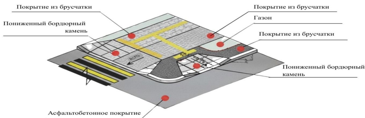
* Рисунок 4 – Пример трапециевидного бордюрного пандуса (Изм.ред. – Приказ КДСиЖКХ от 26.05.2026 г. №57-НК)
