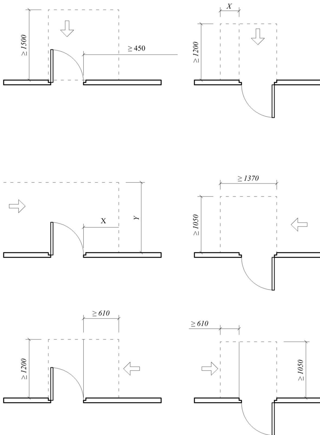
Ж.1-сурет. Мүгедектігі бар адамдар арбасындағы адамдардың жолын ескере отырып, есіктерді орналастыру мен өлшемдер нұсқалары
