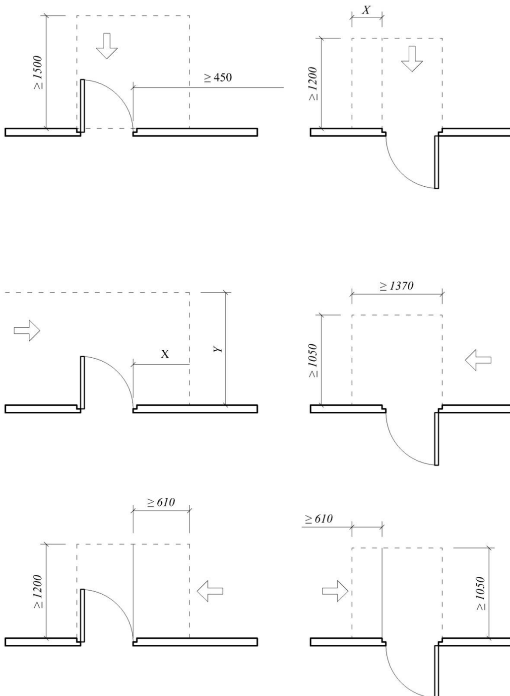
Рисунок Ж.1 – Варианты расположения и параметров дверей с учетом проезда лиц с инвалидностью на креслах-колясках
