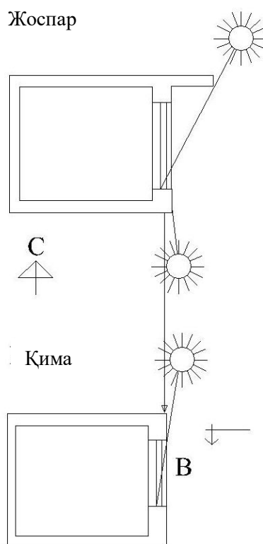
Л.4-суреті – Қабырғаға жалғасқан терезеге есептік нүктені анықтау сызбасы
