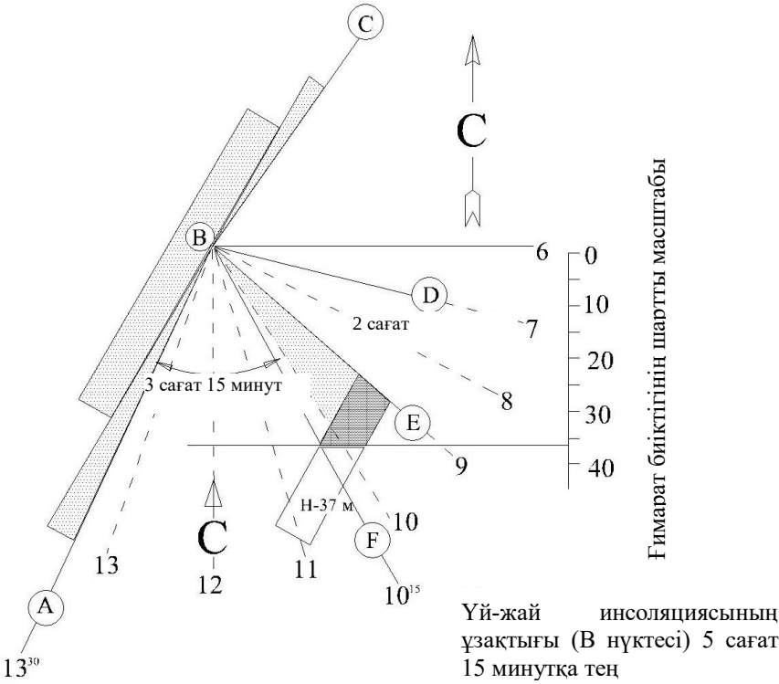
Л.5-суреті - Инсоляцияны анықтау сызбасы
