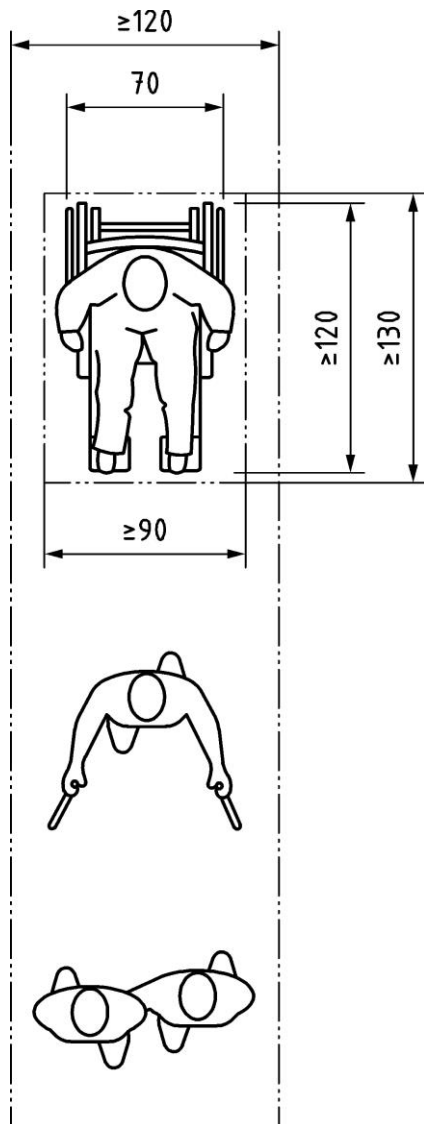
Б.1-суреті – Қимыл бағытын ауыстырусыз епті әдіске қажетті аудан және алаңша
