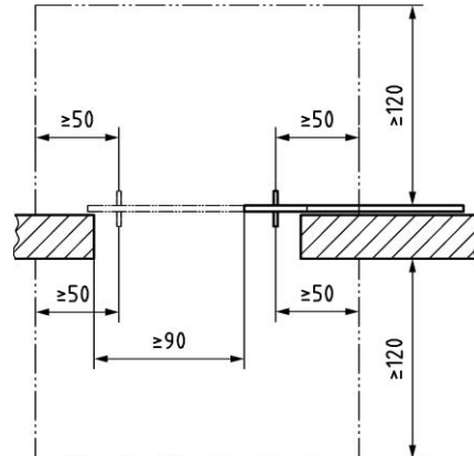
Б.4-суреті – Жылжымалы есіктер алдындағы епті әдіске арналған алаңшалар
