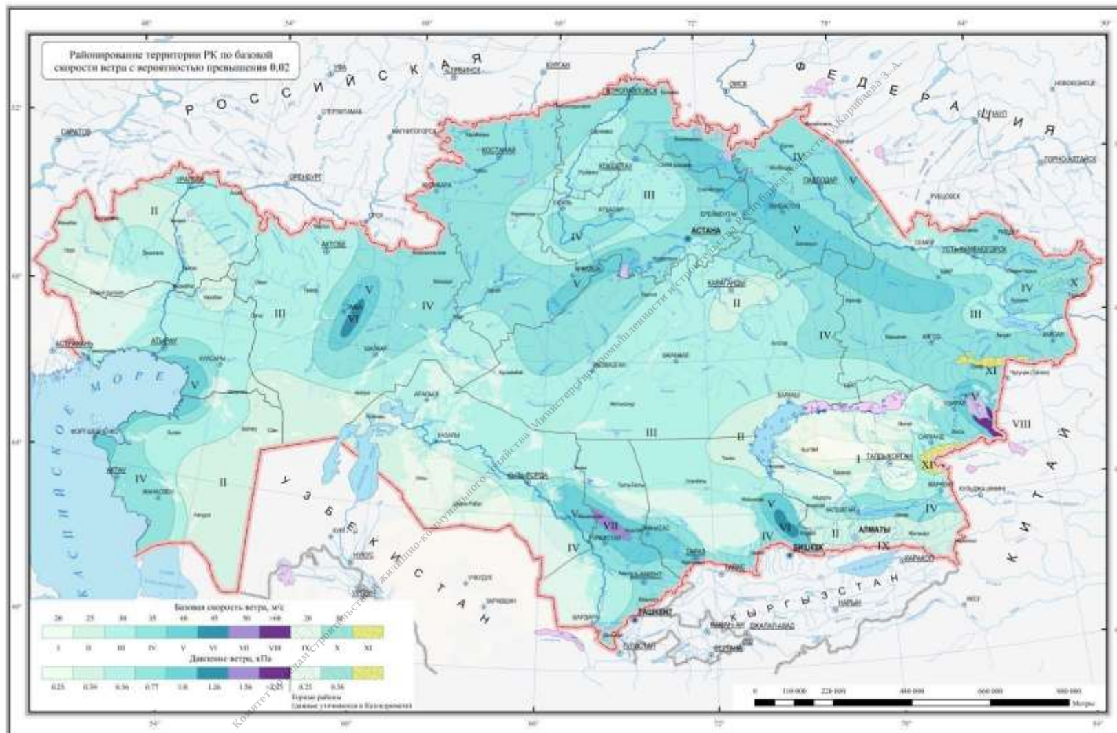
А.3-сурет Желдің негізгі жылдамдығының схемалық картасы
