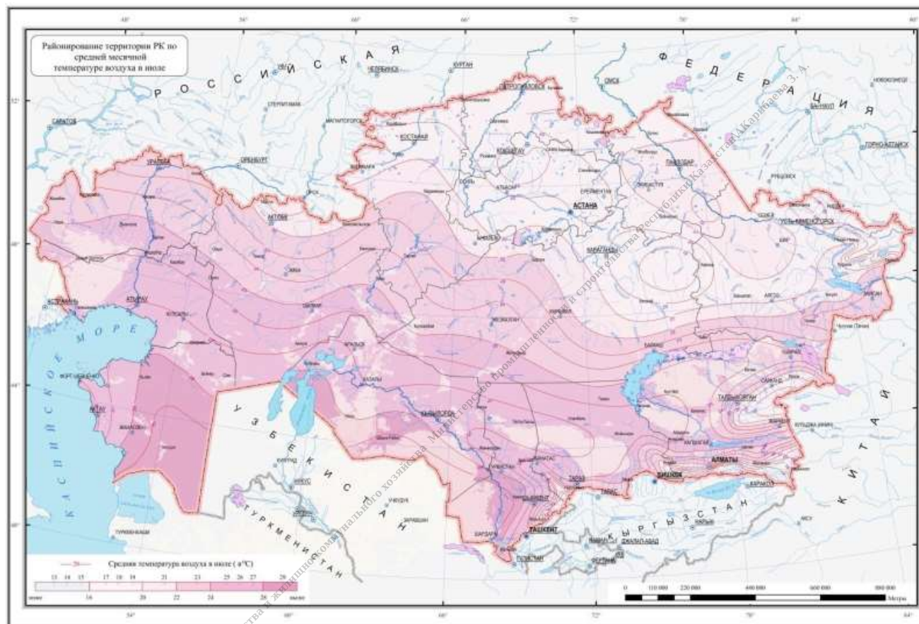
Рисунок А.5 - Схематическая карта средней месячной температуры воздуха в июле
