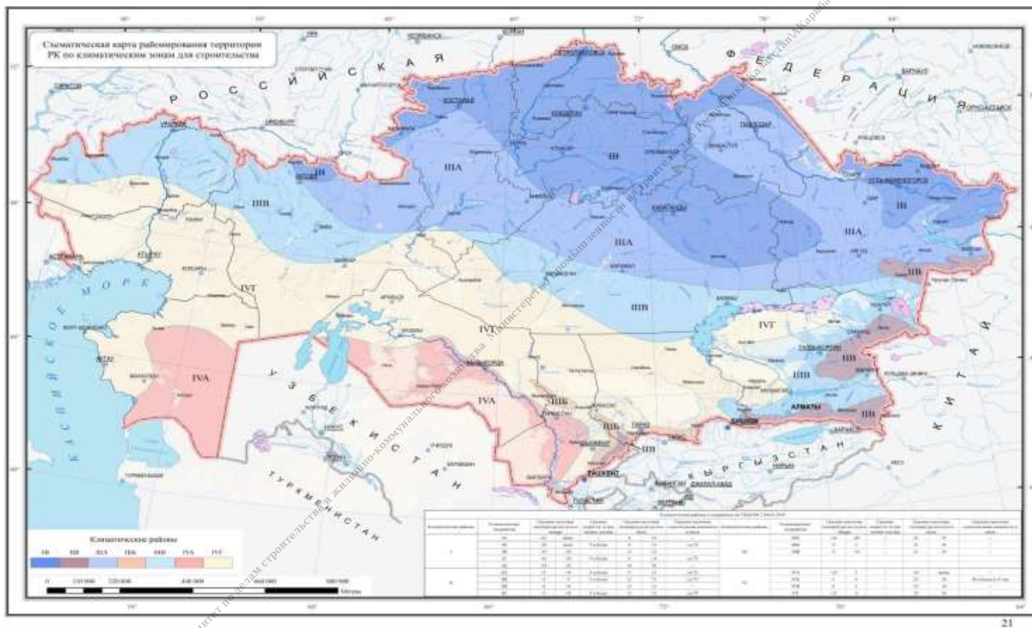
А.1-сурет Қазақстан Республикасы аумағындағы құрылыс үшін климаттық аудандастырудың схемалық картасы
